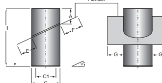
Standard A-Maß TGR
