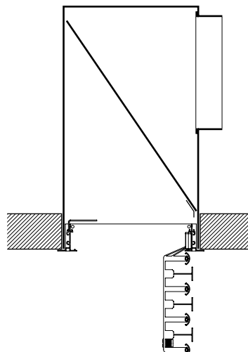
LINED® Linear EO mit Anschlusskasten, öffnenbar, mit Filter, S2 Befestigung
