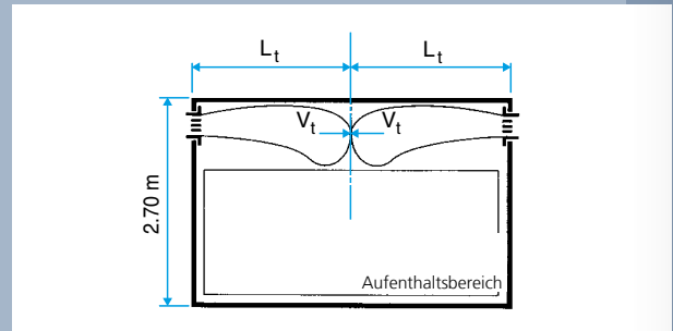
Deckenhöhe von weniger als 3 m - Wanddurchlässe
