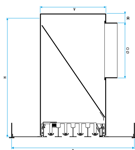
LINED® TP EO, Deckenmontage mit T-Profilen, Abluft mit Filter
