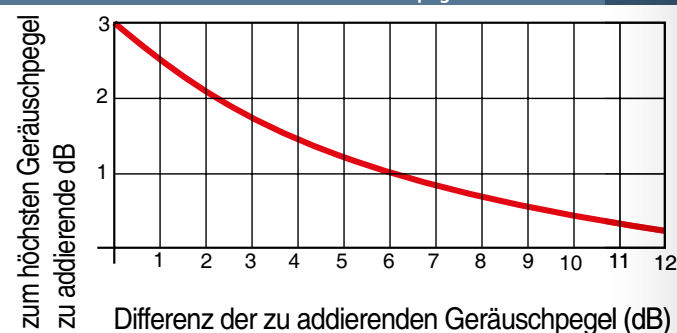
Addition von zwei unterschiedlichen Geräuschpegeln
