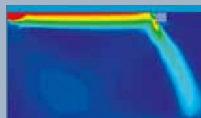
Ein Hindernis wird dann zu einem regelrechten Abweiser, wenn er im Luftstrom, vor allem in den Kaltluftströmen, falsch platziert ist.
