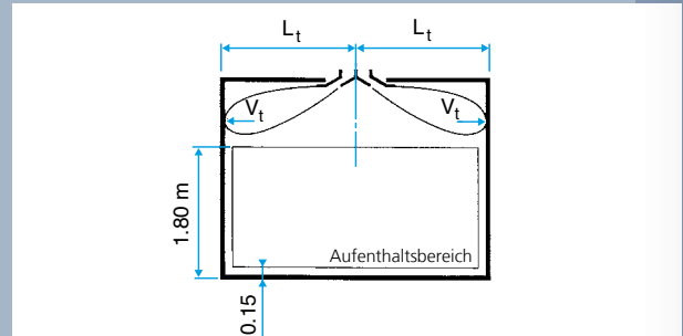
Deckenhöhe von weniger als 3 m - Deckendurchlass
