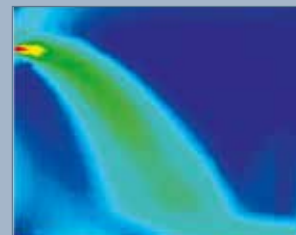
Dieser ohne Coanda-Effekt eingeblasene Zuluftstrom weist einen zu kurzen Luftweg auf und sorgt somit für eine „kalte Dusche“.
