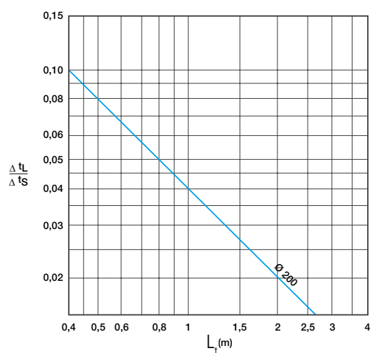
Mischrate für Durchlässe der Reihe LINED®
