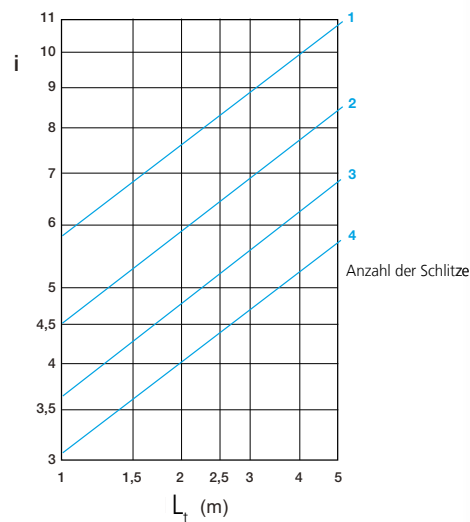
Induktionsrate für Durchlässe der Reihe LINED®
