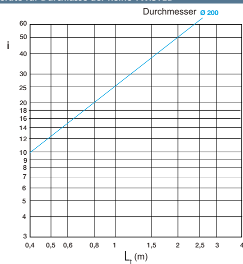
Induktionsrate für Durchlässe der Reihe TWISTED®
