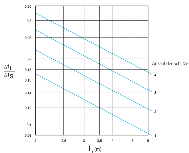
Mischrate für Durchlässe der Reihe LINED®
