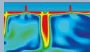
Die Kreuzung der Luftströme mit Geschwindigkeiten von mehr als 0,5 m/s sollte vermieden werden.
