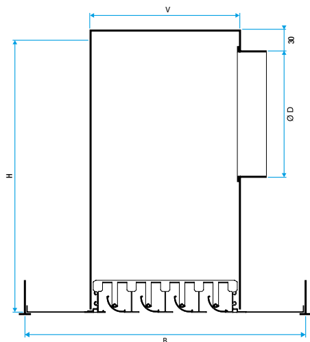
LINED® TP S, Deckenmontage mit T-Profilen, nicht öffnenbar, Zuluft
