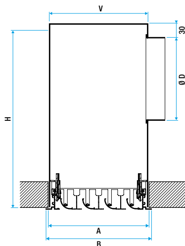
LINED® Linear S mit Anschlusskasten, nicht öffnenbar, S3 Befestigung
