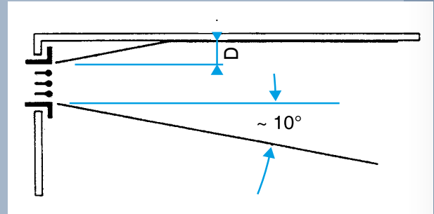
Der Coanda-Effekt ist für einen Abstand D von weniger als 30 cm optimal
