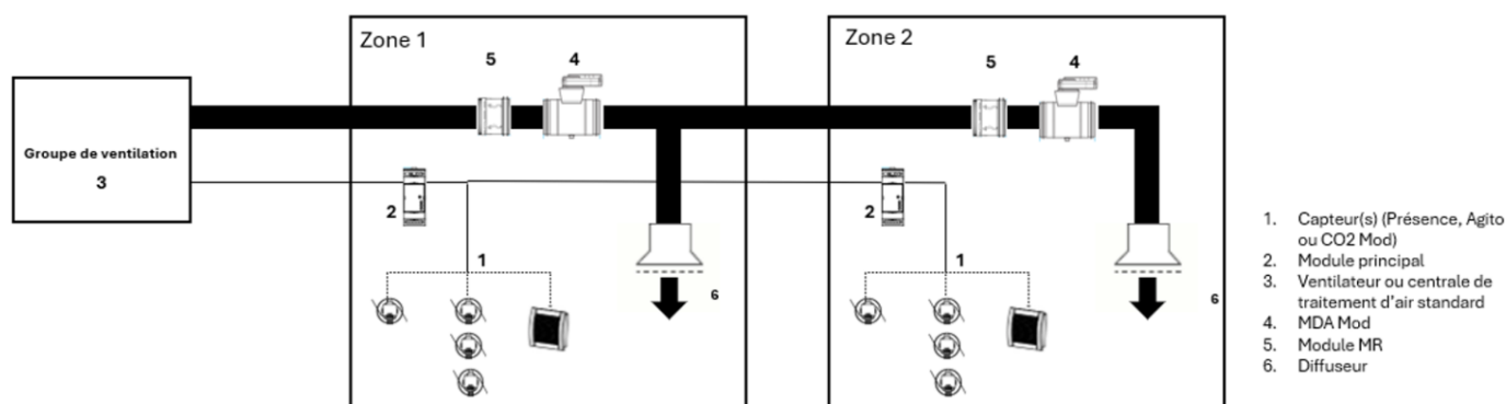
Figure 3 - Cas 1 en zone 1 : branche pilotée directement via le module VMT et le MDA Mod et les capteurs Présence, Agito ou CO 2 -Mod
