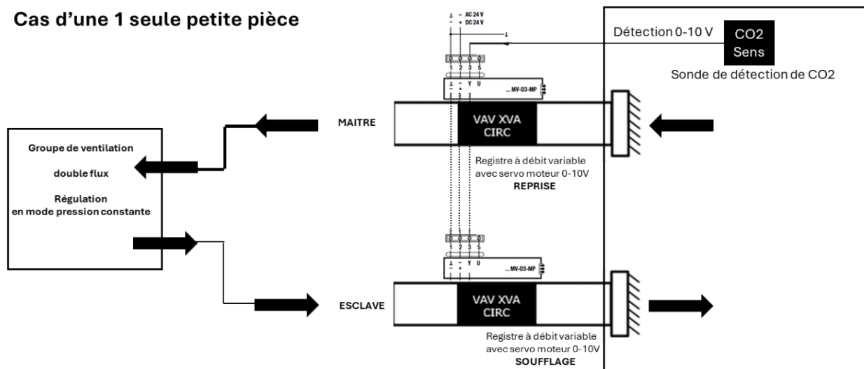
Figure 12b - Pilotage de plusieurs registres à débit variable VAV XVA CIRC en fonctionnement « Maître-Esclaves » : cas d'une petite pièce
