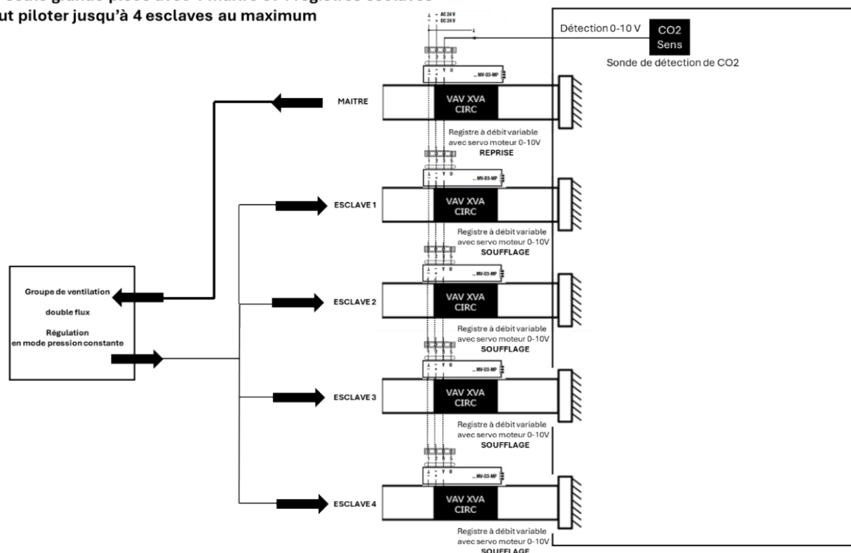
Figure 12d - Pilotage de plusieurs registres à débit variable VAV XVA CIRC en fonctionnement « Maître-Esclaves » : cas d'une grande pièce avec 1 maître et 4 registres esclaves (max)
