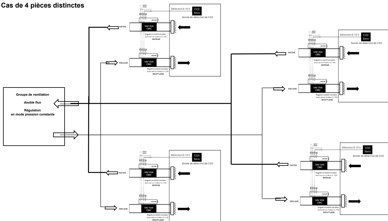
Figure 12e - Pilotage de plusieurs registres à débit variable VAV XVA CIRC en fonctionnement « Maître-Esclaves » : cas de 4 pièces distinctes
