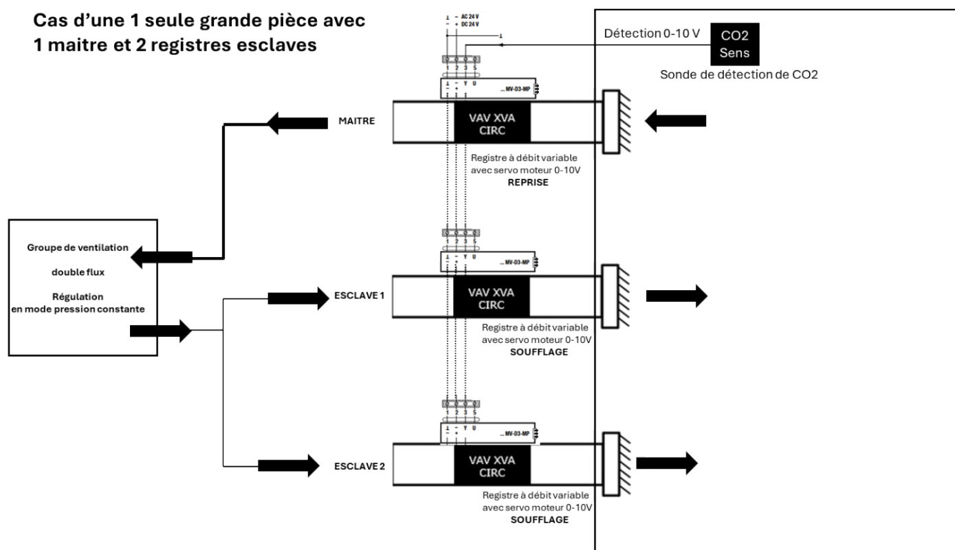
Figure 12c - Pilotage de plusieurs registres à débit variable VAV XVA CIRC en fonctionnement « Maître-Esclaves » : cas d'une grande pièce avec 1 maître et 2 registres esclaves
