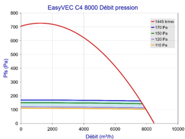
Figure 56 – EasyVEC C4 8000 (avec ou sans T.Flow Hygro+/T.Flow Nano ou T.Flow 105 / T.Flow 180)
