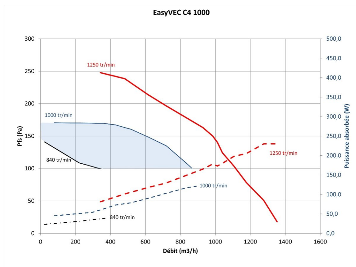
Figure 50 - EasyVEC C4 1000 (avec ou sans T.Flow Hygro+/T.Flow Nano ou T.Flow 105 / T.Flow 180)
