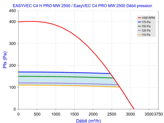
Figure 79 – EasyVEC C4 (H) PRO MW 2500 (avec ou sans T.Flow Hygro+/T.Flow Nano ou T.Flow 105 / T.Flow 180)
