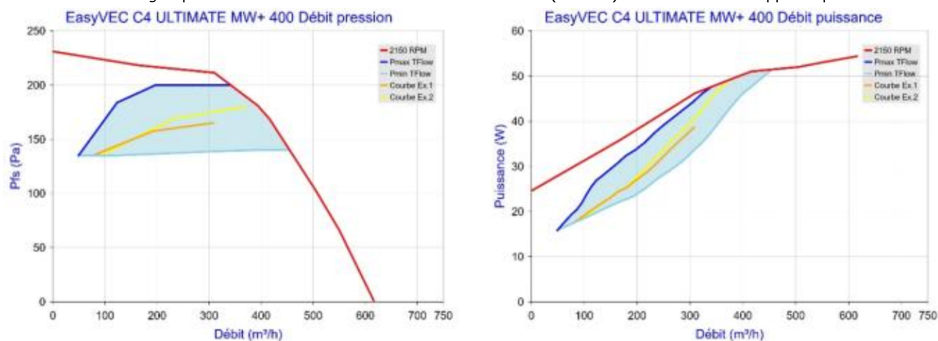
Figure 106 - EasyVEC C4 ULTIMATE MW+ 400 avec T.Flow Hygro+/T.Flow Nano ou T.Flow 105 / T.Flow 180
