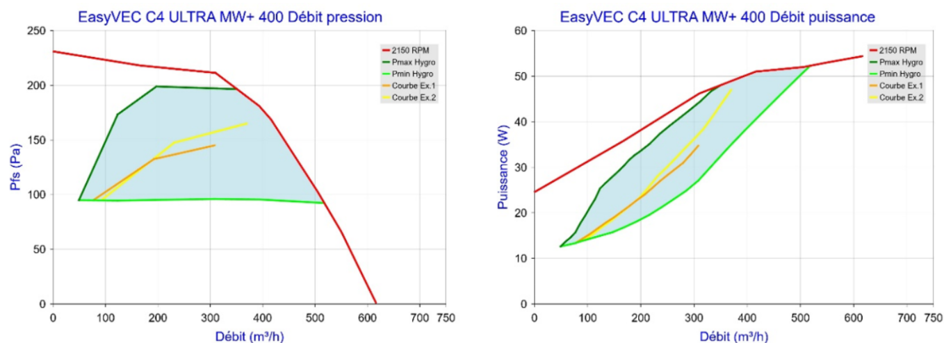
Figure 82 - EasyVEC C4 ULTRA MW+ 400 (sans T.Flow Hygro+/T.Flow Nano ou T.Flow 105 / T.Flow 180)
