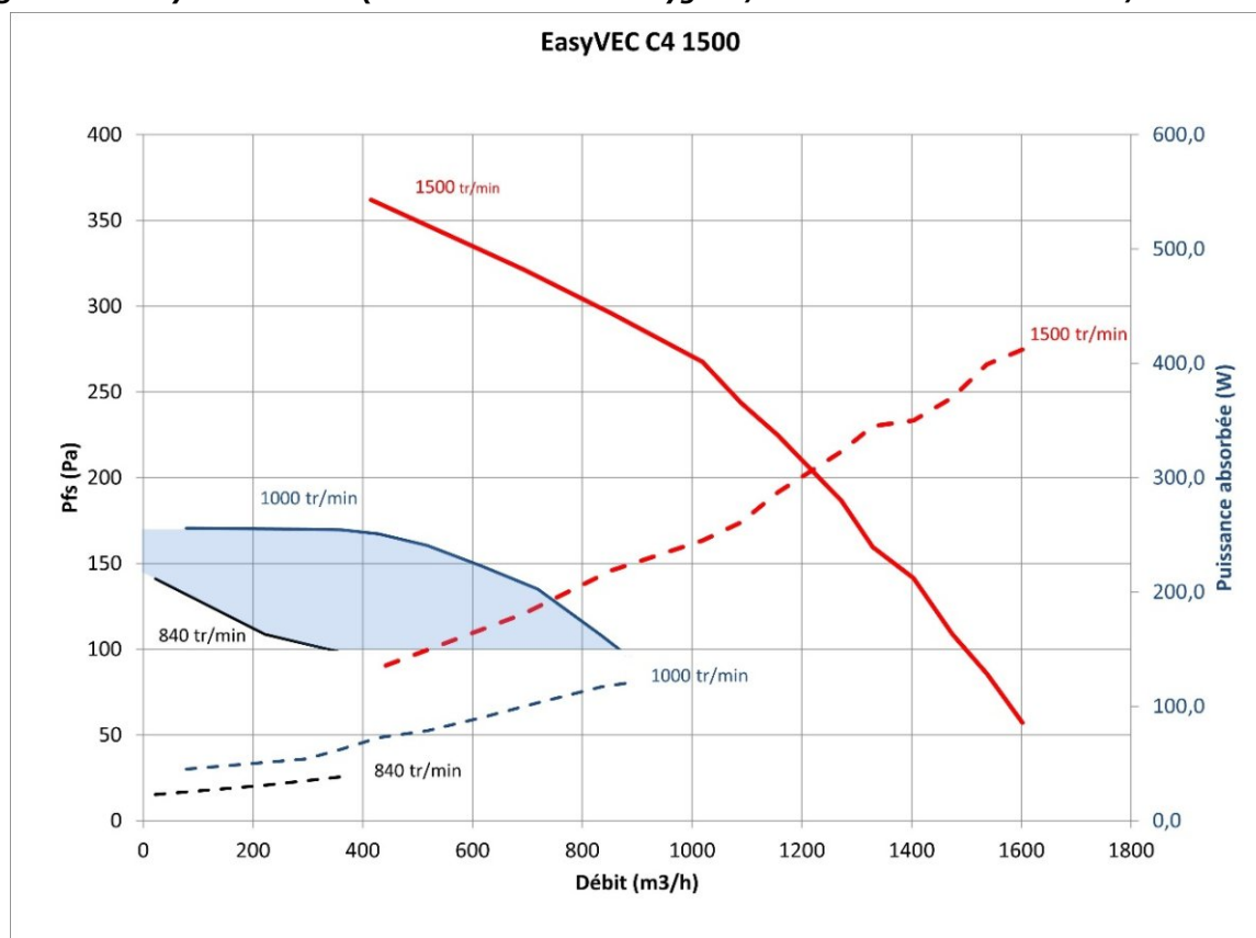
Figure 51 - EasyVEC C4 1500 (avec ou sans T.Flow Hygro+/T.Flow Nano ou T.Flow 105 / T.Flow 180)
