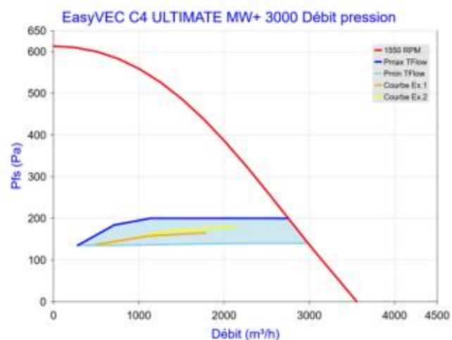
Figure 112 - EasyVEC C4 ULTIMATE MW+ 3000 avec T.Flow Hygro+/T.Flow Nano ou T.Flow 105 / T.Flow 180
