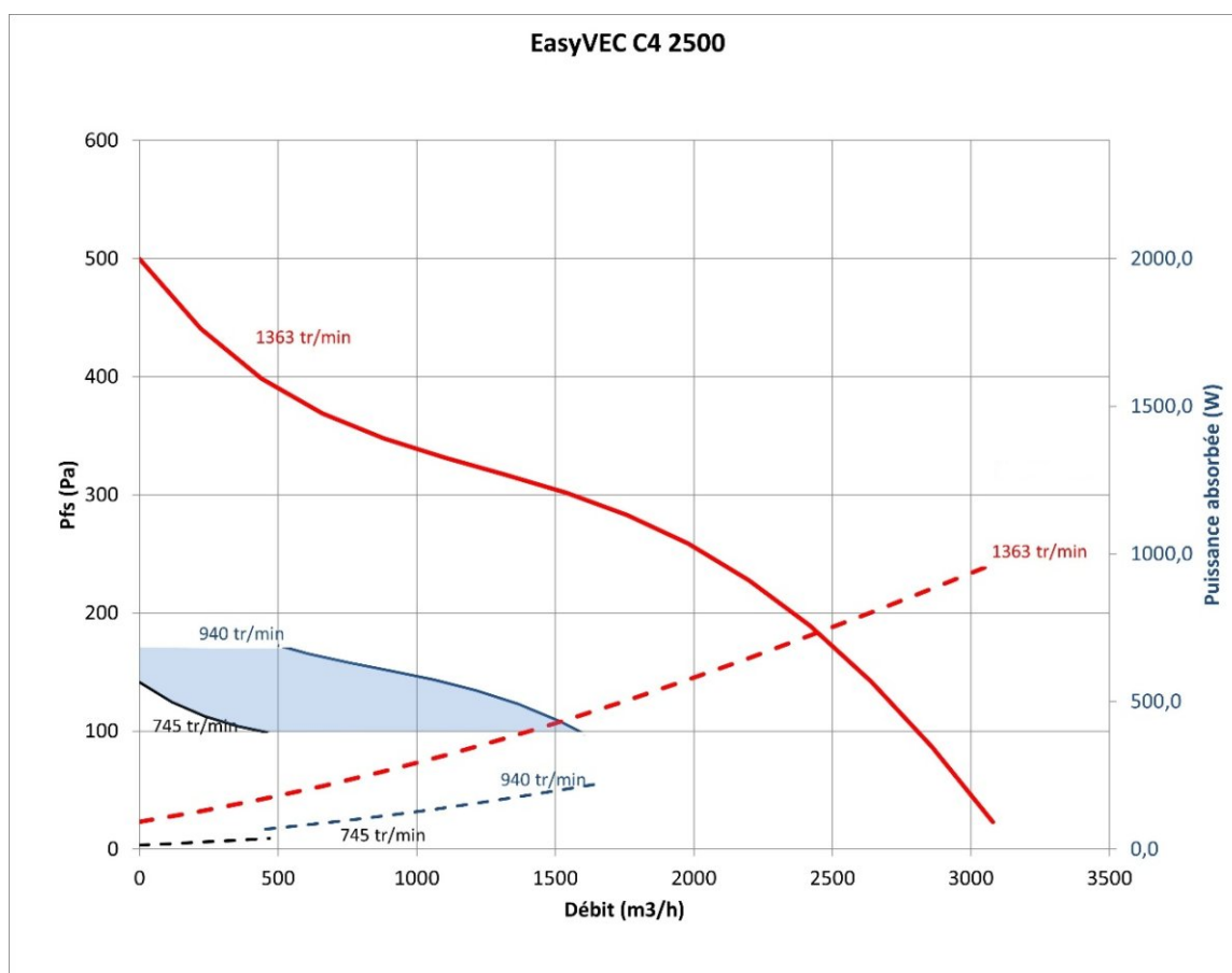
Figure 52 - EasyVEC C4 2500 (avec ou sans T.Flow Hygro+/T.Flow Nano ou T.Flow 105 / T.Flow 180)
