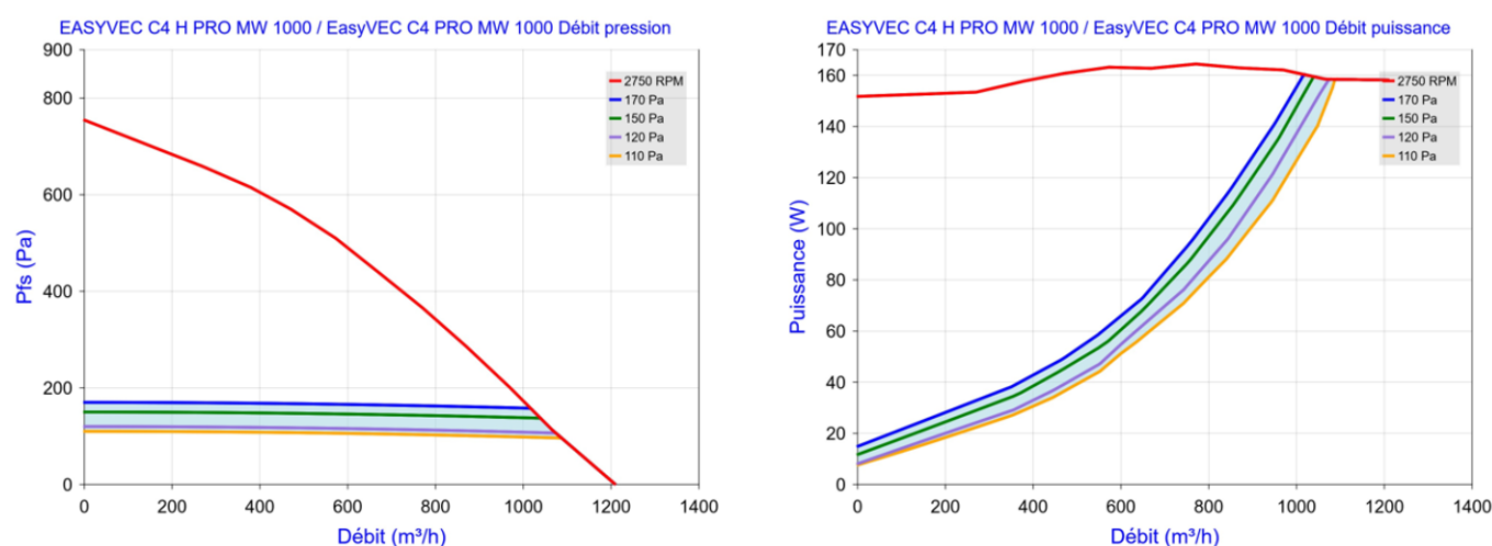
Figure 76 – EasyVEC C4 (H) PRO MW 1000 (avec ou sans T.Flow Hygro+/T.Flow Nano ou T.Flow 105 / T.Flow 180)
