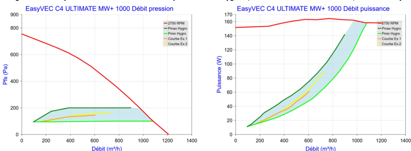
Figure 100 - EasyVEC C4 ULTIMATE MW+ 1000 (sans T.Flow Hygro+/T.Flow Nano ou T.Flow 105 / T.Flow 180)
