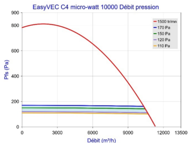
Figure 62 – EasyVEC C4 micro-watt 10000 (avec ou sans T.Flow Hygro+/T.Flow Nano ou T.Flow 105 / T.Flow 180)
