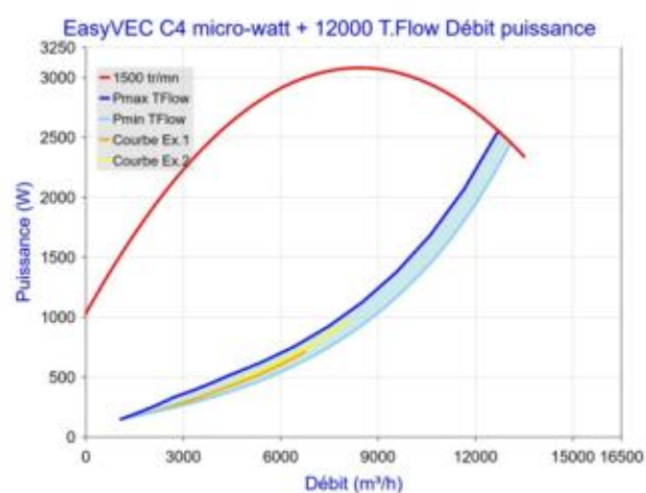
Figure 73 - EasyVEC C4 micro-watt + 12000 avec T.Flow Hygro+/ T.Flow Nano ou T.Flow 105 / T.Flow 180
