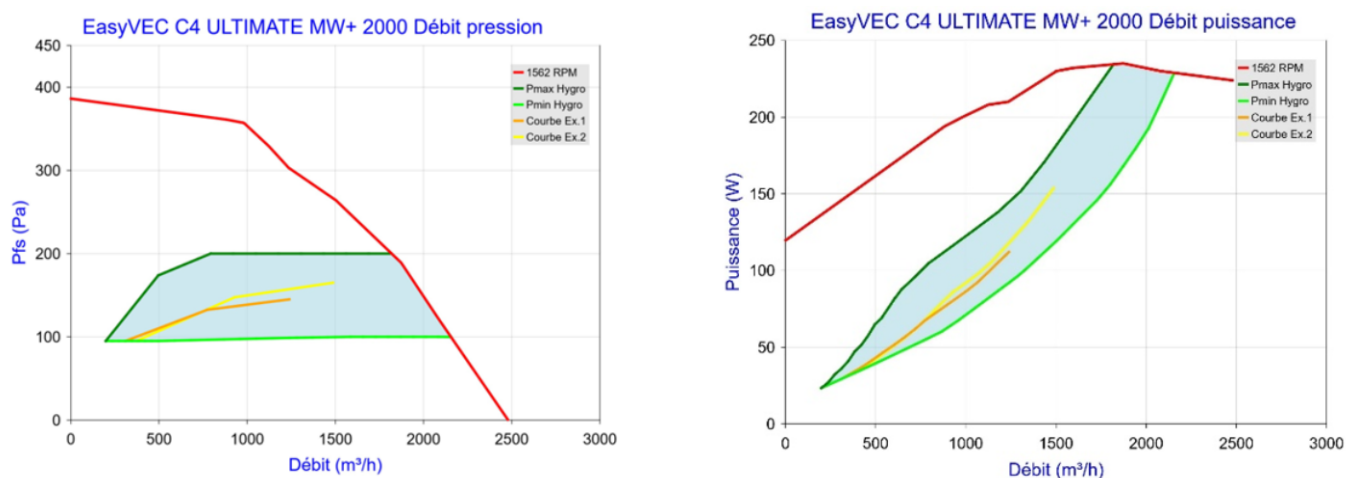
Figure 102- EasyVEC C4 ULTIMATE MW+ 2000 (sans T.Flow Hygro+/T.Flow Nano ou T.Flow 105 / T.Flow 180)
