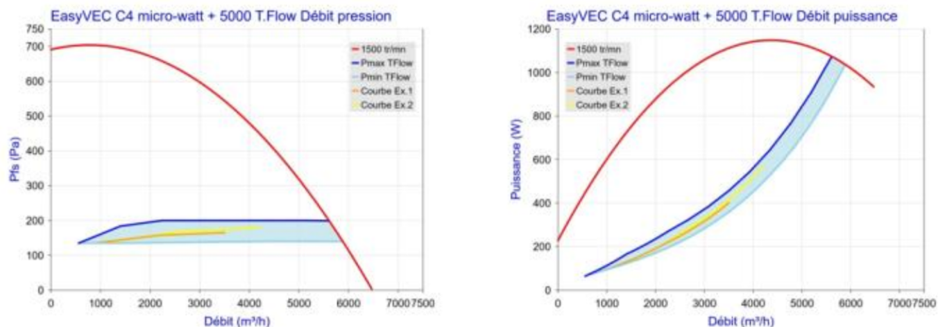
Figure 69 - EasyVEC C4 micro-watt + 5000 avec T.Flow Hygro+ / T.Flow Nano ou T.Flow 105 / T.Flow 180
