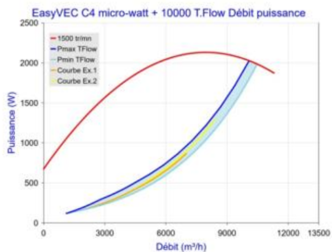
Figure 72 - EasyVEC C4 micro-watt + 10000 avec T.Flow Hygro+/ T.Flow Nano ou T.Flow 105 / T.Flow 180
