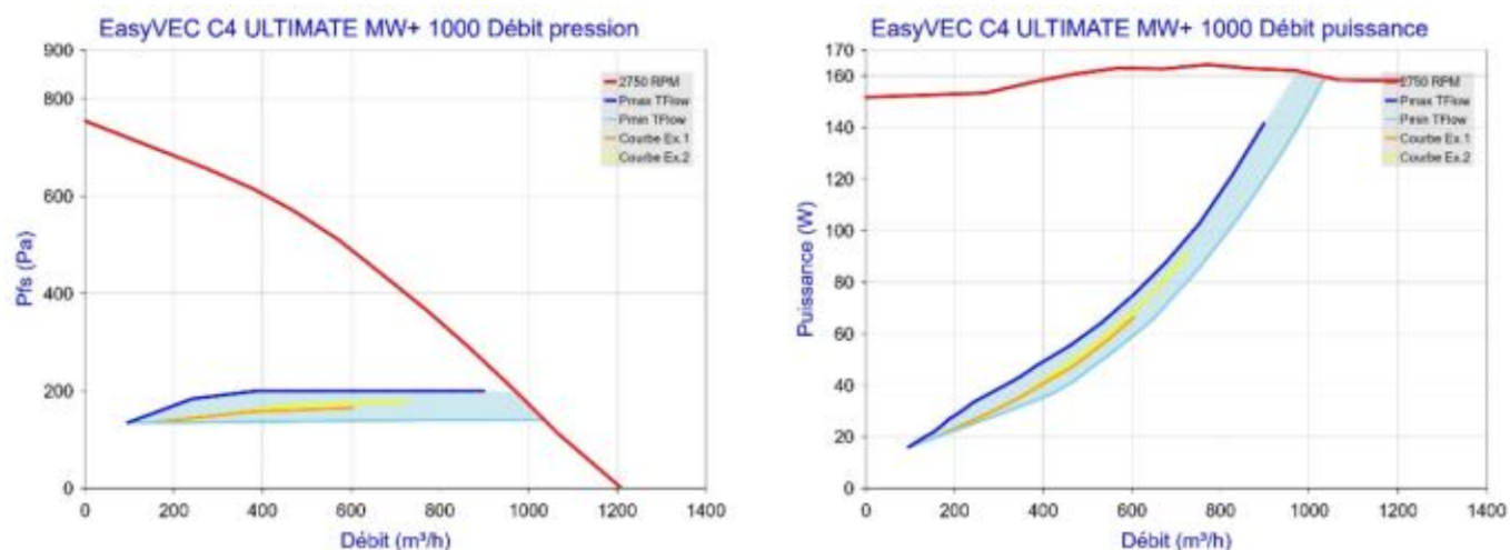
Figure 108 - EasyVEC C4 ULTIMATE MW+ 1000 avec T.Flow Hygro+/T.Flow Nano ou T.Flow 105 / T.Flow 180
