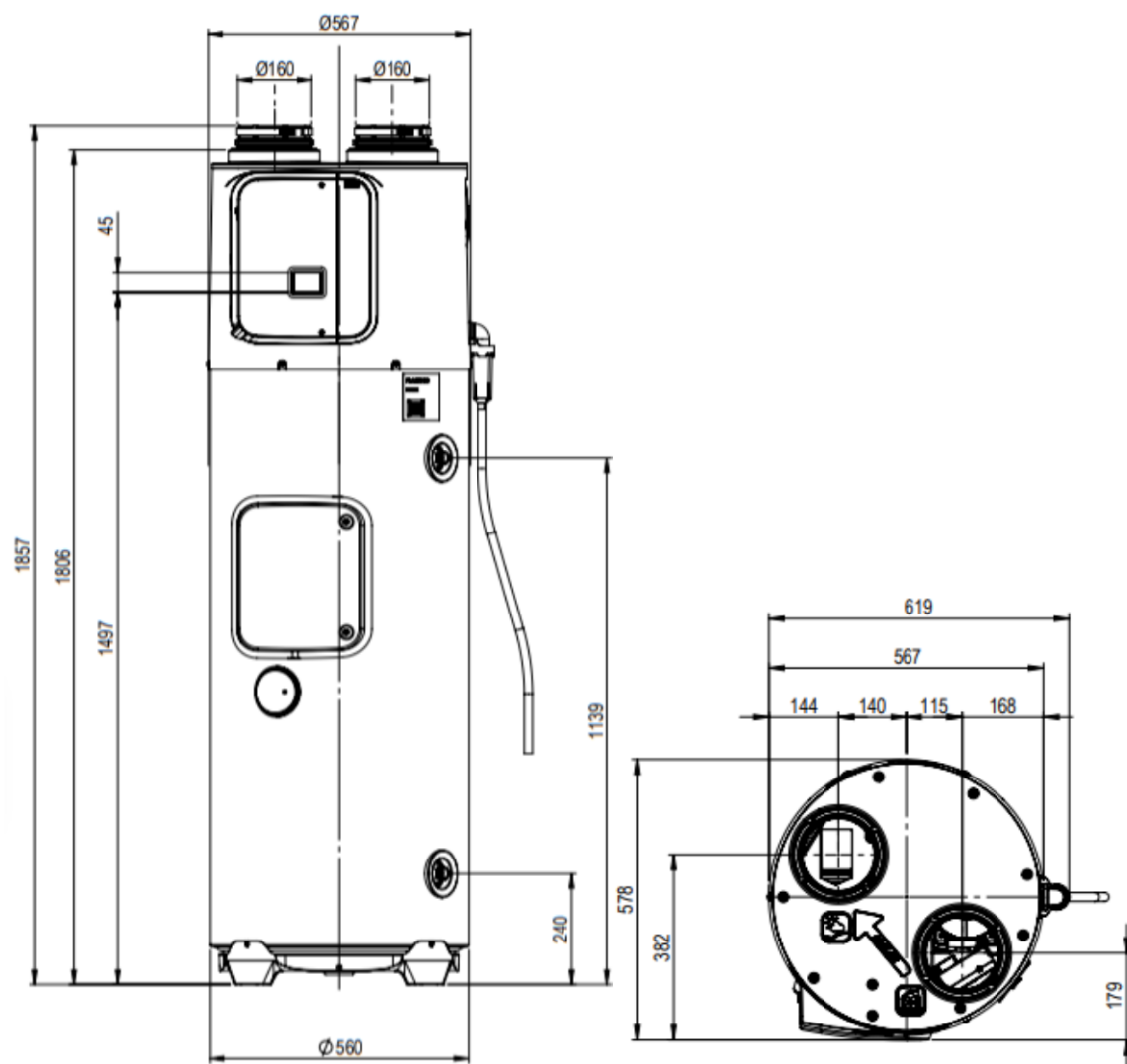
Figure 116 – Chauffe-eau thermodynamique sur air extrait « T.Flow 180 » - visuels d'encombrement
