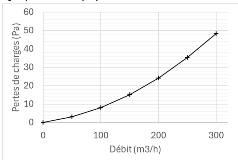
Figure 119 – Chauffe-eau thermodynamique sur air extrait
