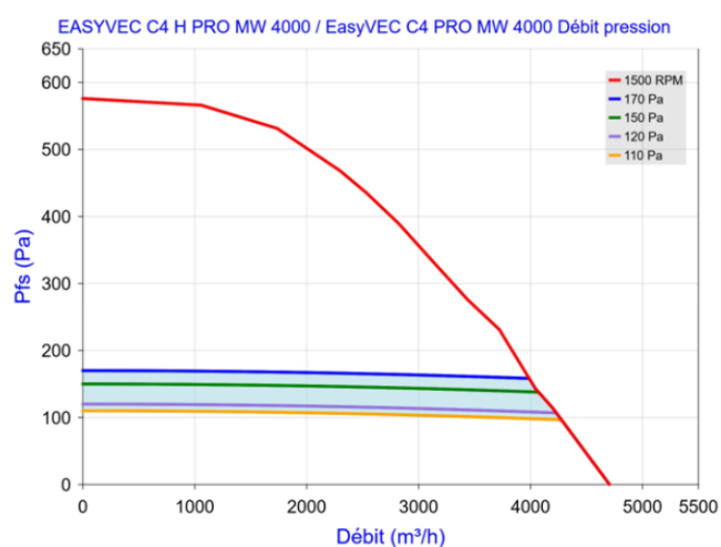
Figure 81 – EasyVEC C4 (H) PRO MW 4000 (avec ou sans T.Flow Hygro+/T.Flow Nano ou T.Flow 105 / T.Flow 180)
