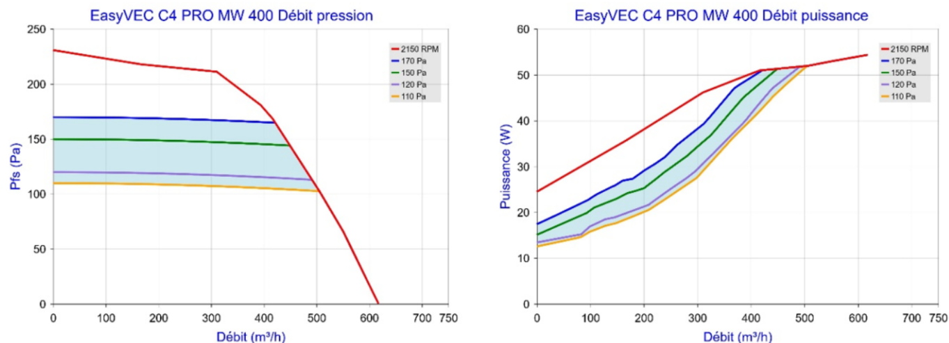
Figure 74 – EasyVEC C4 PRO MW 400 (avec ou sans T.Flow Hygro+/T.Flow Nano ou T.Flow 105 / T.Flow 180)
