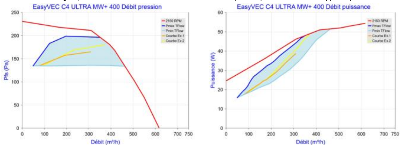
Figure 90 - EasyVEC C4 ULTRA MW+ 400 avec T.Flow Hygro+ / T.Flow Nano ou T.Flow 105 / T.Flow 180
