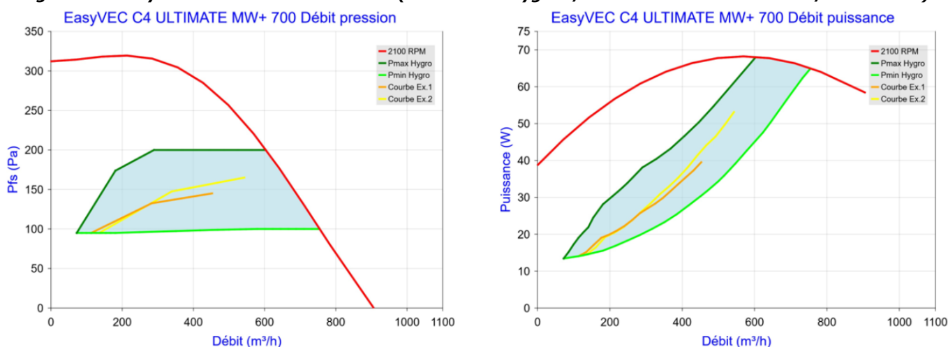
Figure 99 - EasyVEC C4 ULTIMATE MW+ 700 (sans T.Flow Hygro+/T.Flow Nano ou T.Flow 105 / T.Flow 180)
