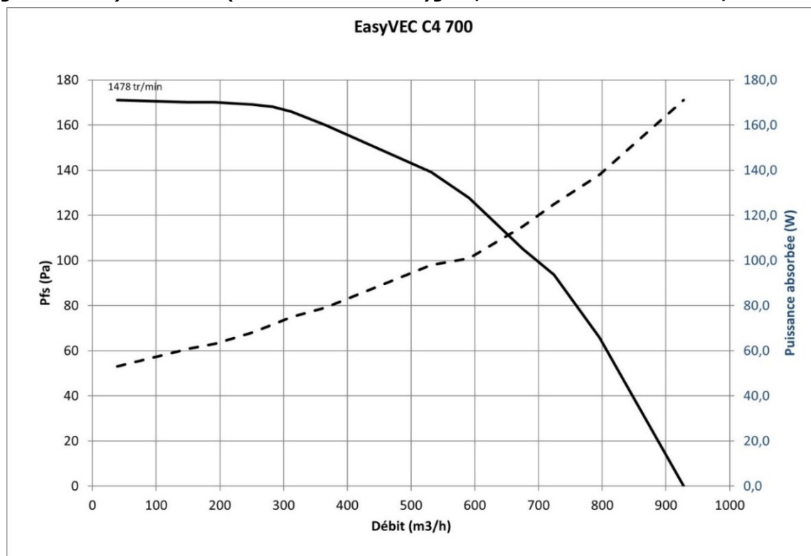
Figure 49 - EasyVEC C4 700 (avec ou sans T.Flow Hygro+/T.Flow Nano ou T.Flow 105 / T.Flow 180)
