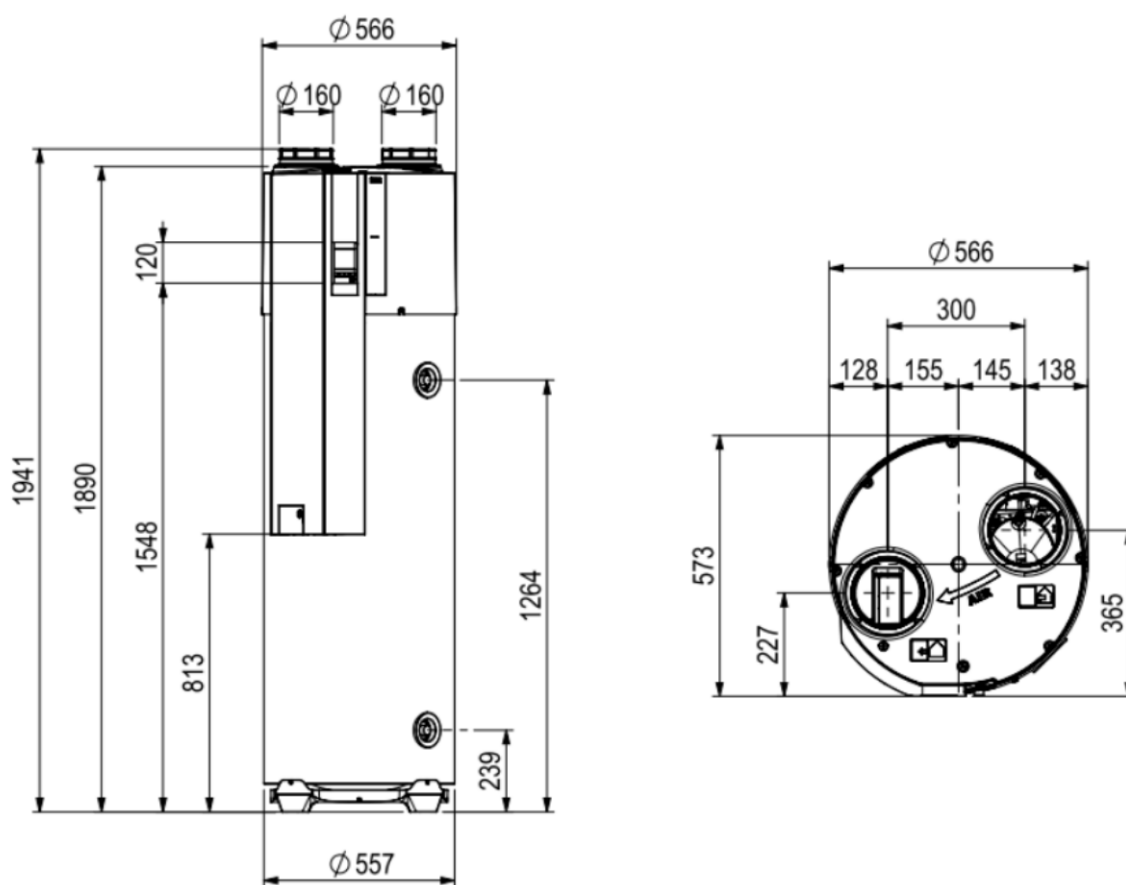
Figure 114 – Ballon d'ECS thermodynamique « B200_T.Flow Hygro+ » (pour application T.Flow Hygro+)
