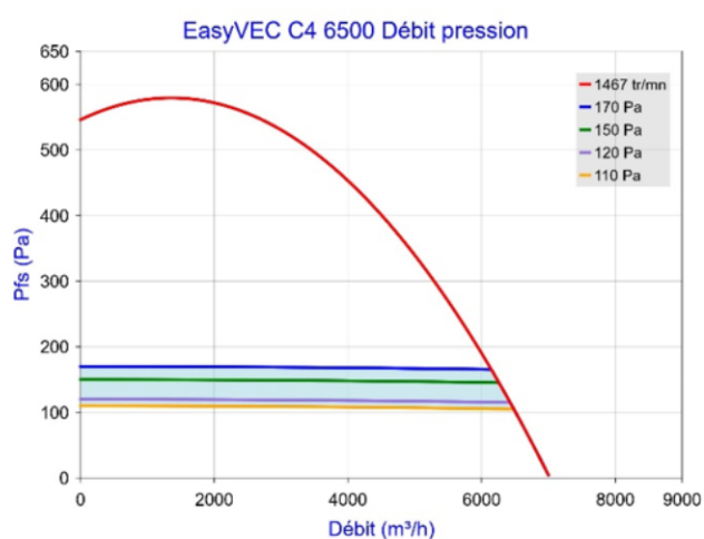
Figure 55 – EasyVEC C4 6500 (avec ou sans T.Flow Hygro+/T.Flow Nano ou T.Flow 105 / T.Flow 180)
