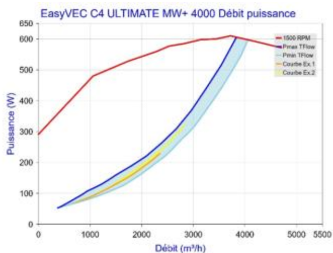
Figure 113 - EasyVEC C4 ULTIMATE MW+ 4000 avec T.Flow Hygro+/T.Flow Nano ou T.Flow 105 / T.Flow 180
