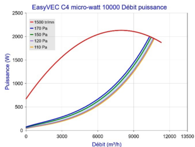
Figure 62 – EasyVEC C4 micro-watt 10000 (avec ou sans T.Flow Hygro+/T.Flow Nano ou T.Flow 105 / T.Flow 180)
