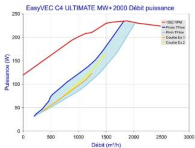
Figure 110 - EasyVEC C4 ULTIMATE MW+ 2000 avec T.Flow Hygro+/T.Flow Nano ou T.Flow 105 / T.Flow 180
