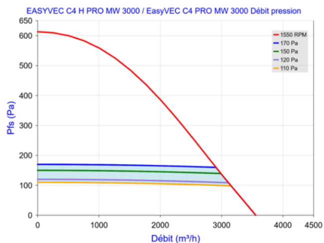
Figure 80 – EasyVEC C4 (H) PRO MW 3000 (avec ou sans T.Flow Hygro+/T.Flow Nano ou T.Flow 105 / T.Flow 180)
