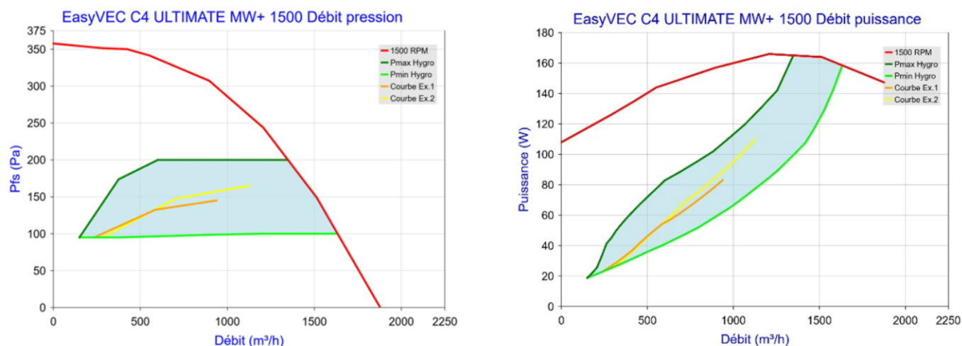
Figure 101 - EasyVEC C4 ULTIMATE MW+ 1500 (sans T.Flow Hygro+/T.Flow Nano ou T.Flow 105 / T.Flow 180)
