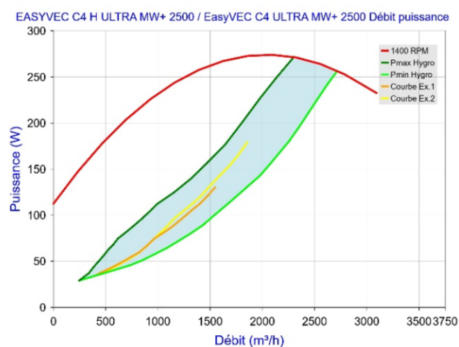
Figure 87 - EasyVEC C4 (H) ULTRA MW+ 2500 (sans T.Flow Hygro+/T.Flow Nano ou T.Flow 105 / T.Flow 180)
