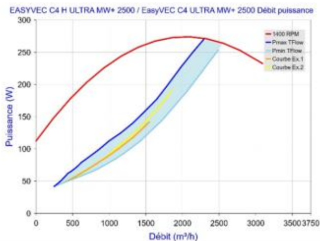
Figure 95 - EasyVEC C4 (H) ULTRA MW+ 2500 avec T.Flow Hygro+/ T.Flow Nano ou T.Flow 105 / T.Flow 180
