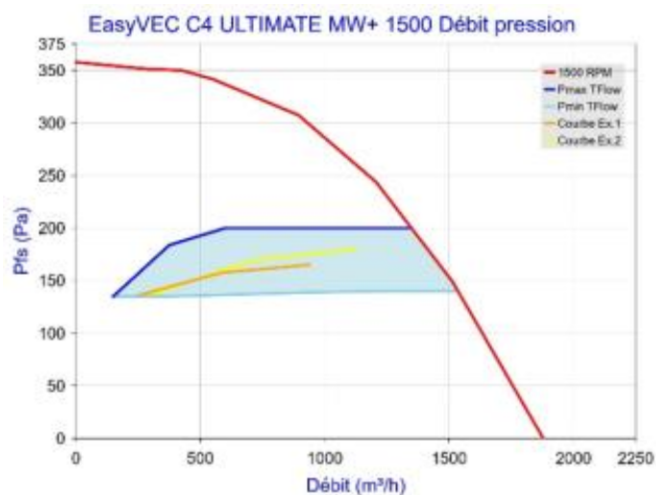
Figure 109 - EasyVEC C4 ULTIMATE MW+ 1500 avec T.Flow Hygro+/T.Flow Nano ou T.Flow 105 / T.Flow 180
