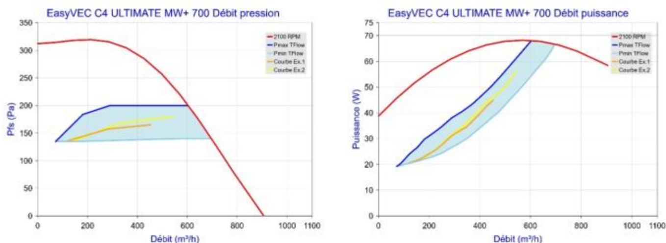
Figure 107 - EasyVEC C4 ULTIMATE MW+ 700 avec T.Flow Hygro+/T.Flow Nano ou T.Flow 105 / T.Flow 180
