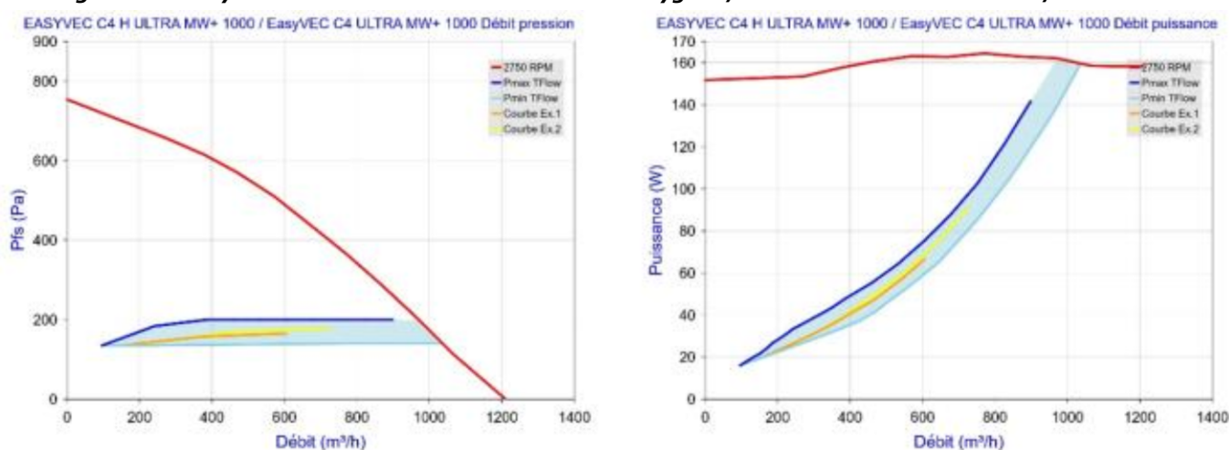
Figure 92 - EasyVEC C4 (H) ULTRA MW+ 1000 avec T.Flow Hygro+ / T.Flow Nano ou T.Flow 105 / T.Flow 180
