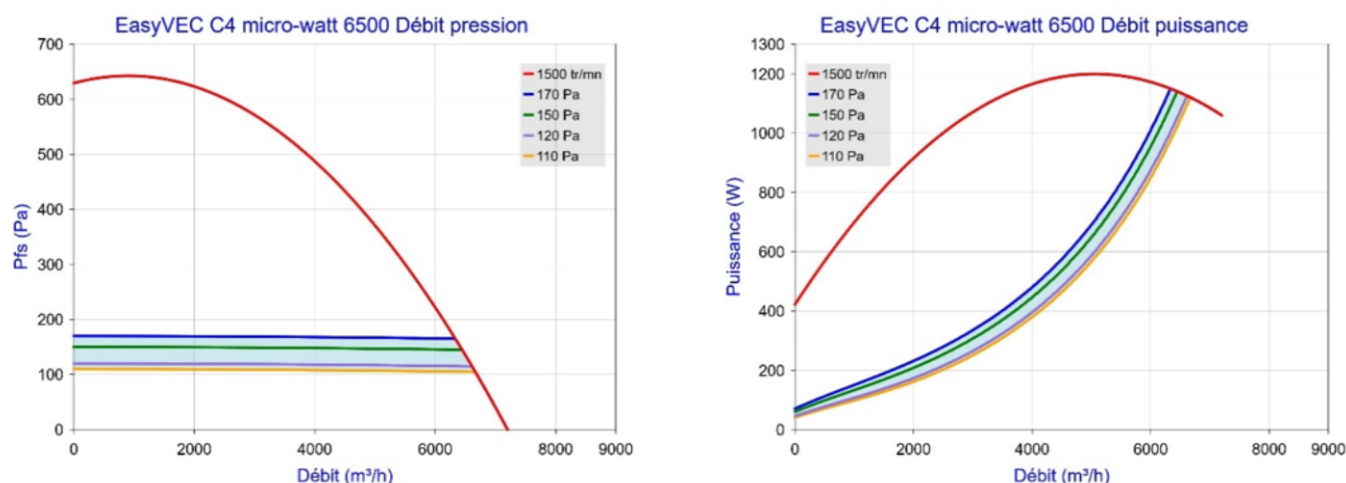
Figure 60 – EasyVEC C4 micro-watt 6500 (avec ou sans T.Flow Hygro+/T.Flow Nano ou T.Flow 105 / T.Flow 180)
