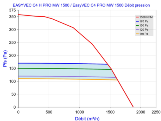
Figure 77 – EasyVEC C4 (H) PRO MW 1500 (avec ou sans T.Flow Hygro+/T.Flow Nano ou T.Flow 105 / T.Flow 180)
