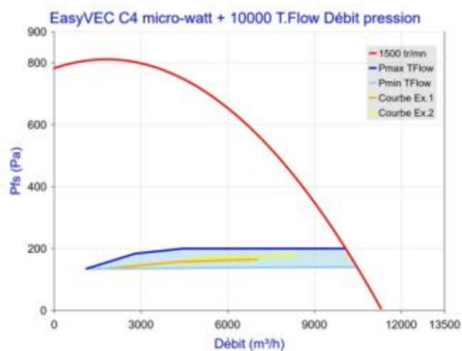
Figure 72 - EasyVEC C4 micro-watt + 10000 avec T.Flow Hygro+/ T.Flow Nano ou T.Flow 105 / T.Flow 180
