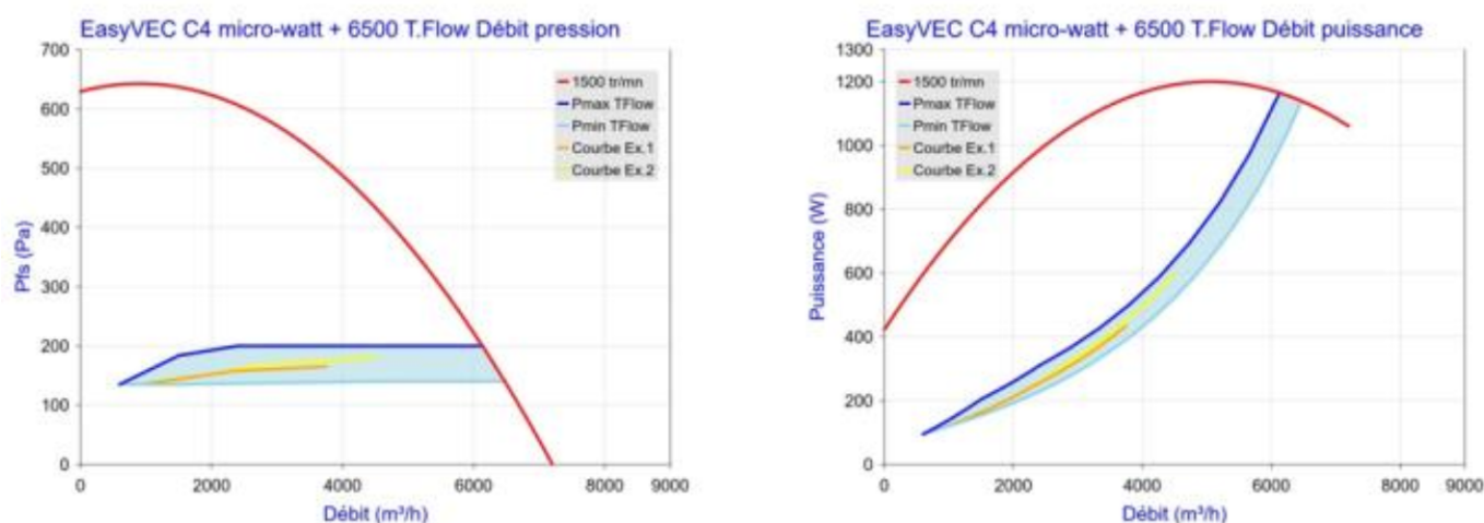
Figure 70 - EasyVEC C4 micro-watt + 6500 avec T.Flow Hygro+ / T.Flow Nano ou T.Flow 105 / T.Flow 180
