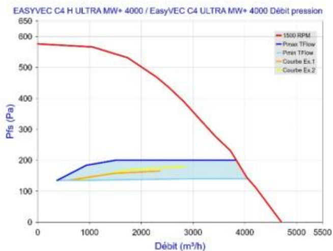
Figure 97 - EasyVEC C4 (H) ULTRA MW+ 4000 avec T.Flow Hygro+/ T.Flow Nano ou T.Flow 105 / T.Flow 180
