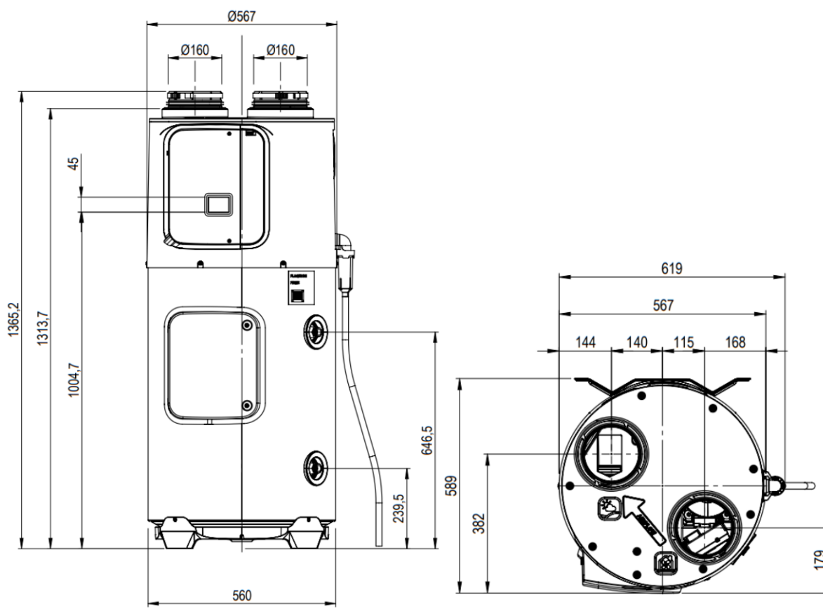
Figure 117 – Chauffe-eau thermodynamique sur air extrait « T.Flow 105 »- visuels d'encombrement
