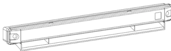
Figure 18 – Auvent acoustique standard EHL [7] et[8]
