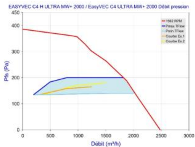
Figure 94 - EasyVEC C4 (H) ULTRA MW+ 2000 avec T.Flow Hygro+/ T.Flow Nano ou T.Flow 105 / T.Flow 180
