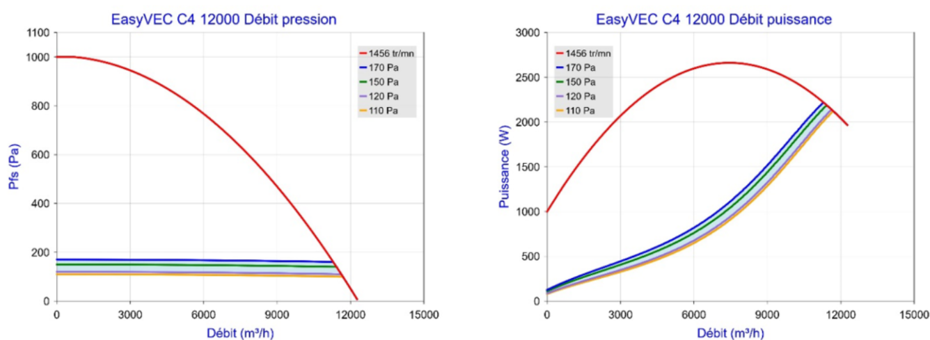
Figure 58 – EasyVEC C4 12 0000 (avec ou sans T.Flow Hygro+/T.Flow Nano ou T.Flow 105 / T.Flow 180)
