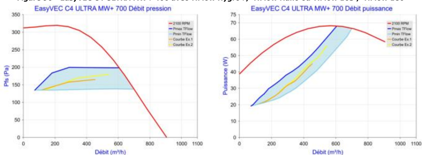
Figure 91 - EasyVEC C4 ULTRA MW+ 700 avec T.Flow Hygro+/T.Flow Nano ou T.Flow 105 / T.Flow 180
