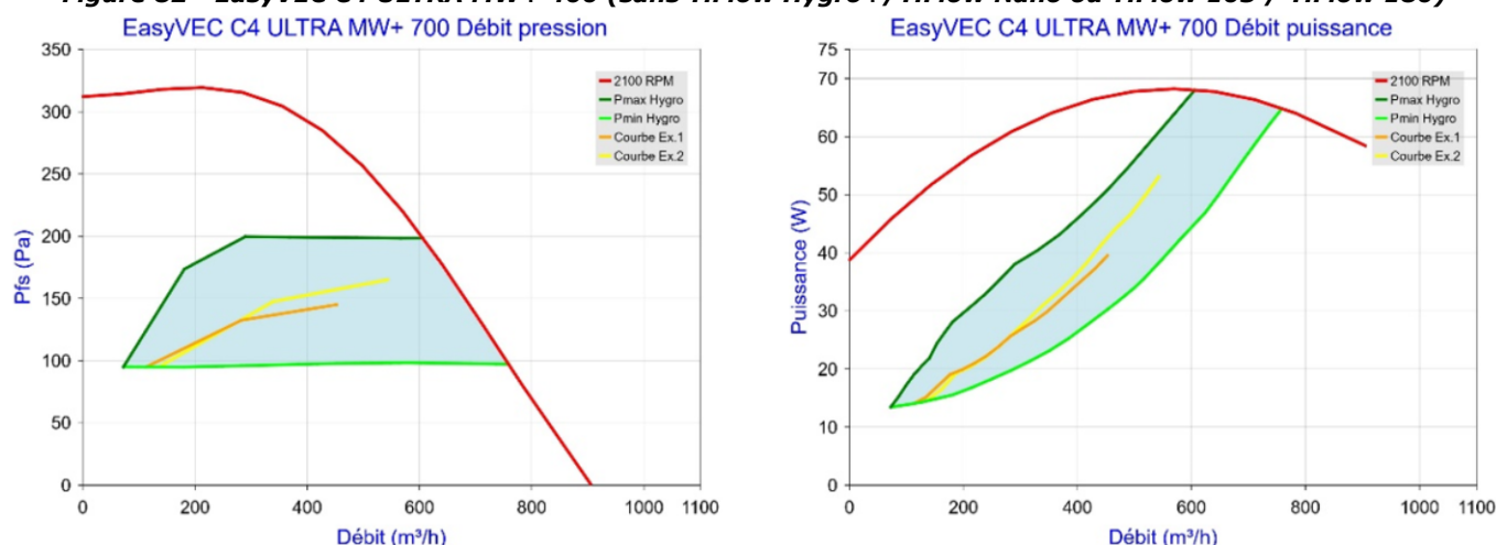
Figure 83 - EasyVEC C4 ULTRA MW+ 700 (sans T.Flow Hygro+/T.Flow Nano ou T.Flow 105 / T.Flow 180)
