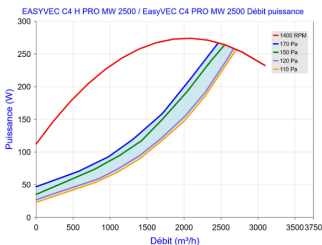
Figure 79 – EasyVEC C4 (H) PRO MW 2500 (avec ou sans T.Flow Hygro+/T.Flow Nano ou T.Flow 105 / T.Flow 180)
