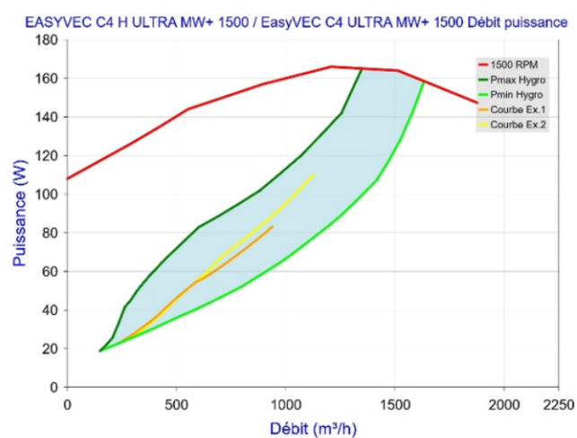
Figure 85 - EasyVEC C4 (H) ULTRA MW+ 1500 (sans T.Flow Hygro+/T.Flow Nano ou T.Flow 105 / T.Flow 180)
