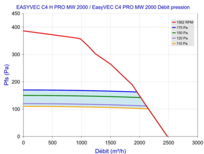
Figure 78 – EasyVEC C4 (H) PRO MW 2000 (avec ou sans T.Flow Hygro+/T.Flow Nano ou T.Flow 105 / T.Flow 180)
