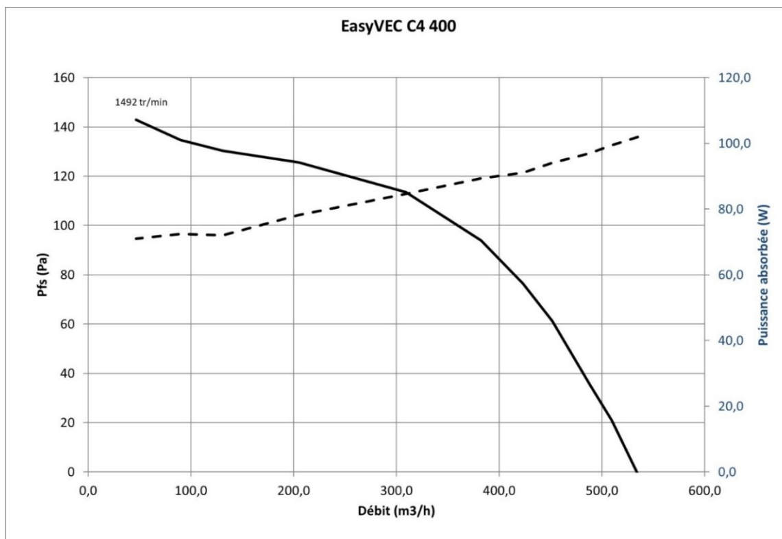
Figure 48 - EasyVEC C4 400 (avec ou sans T.Flow Hygro+/T.Flow Nano ou T.Flow 105 / T.Flow 180)
