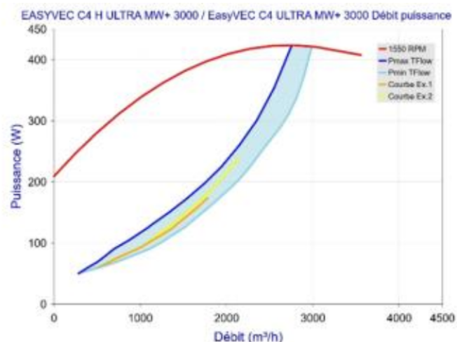
Figure 96 - EasyVEC C4 (H) ULTRA MW+ 3000 avec T.Flow Hygro+/T.Flow Nano ou T.Flow 105 / T.Flow 180
