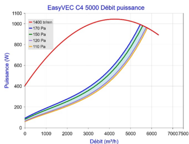
Figure 54 – EasyVEC C4 5000 (avec ou sans T.Flow Hygro+/T.Flow Nano ou T.Flow 105 / T.Flow 180)
