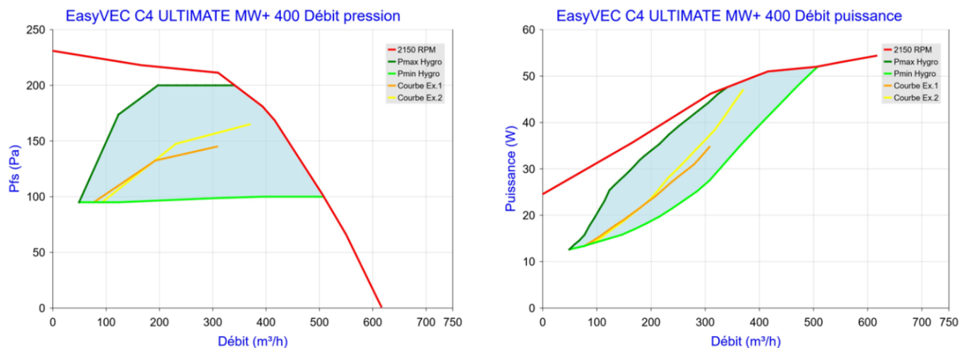
Figure 98 - EasyVEC C4 ULTIMATE MW+ 400 (sans T.Flow Hygro+/T.Flow Nano ou T.Flow 105 / T.Flow 180)
