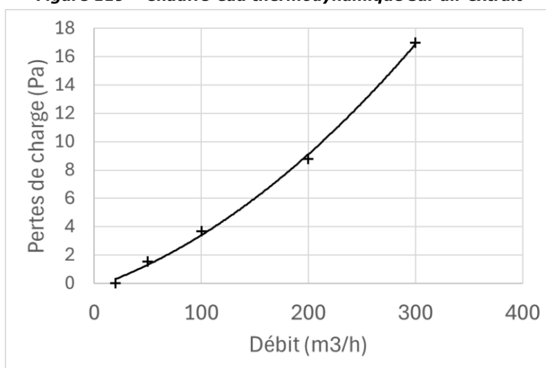
Figure 120 – Courbe de pertes de charge complémentaire modélisant l'encrassement du filtre
