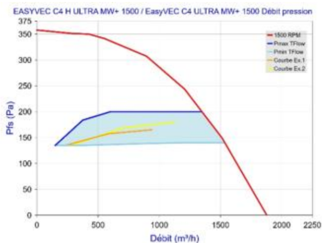
Figure 93 - EasyVEC C4 (H) ULTRA MW+ 1500 avec T.Flow Hygro+/T.Flow Nano ou T.Flow 105 / T.Flow 180
