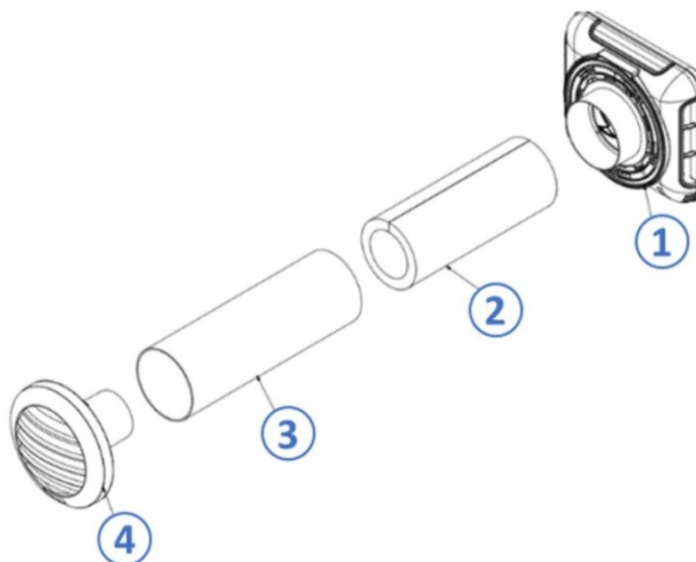
Figure 24 – Mise en œuvre entrée d'air EHT² et EFT² sans mousse Ø 100 mm L 300 mm
