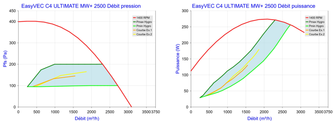
Figure 103 - EasyVEC C4 ULTIMATE MW+ 2500 (sans T.Flow Hygro+/T.Flow Nano ou T.Flow 105 / T.Flow 180)
