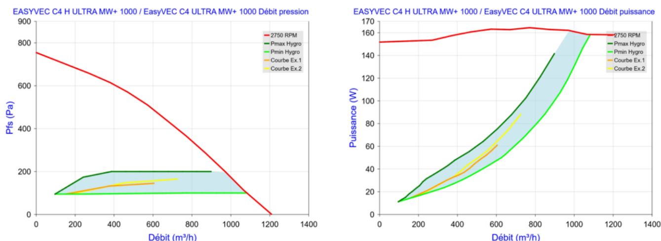
Figure 84 - EasyVEC C4 (H) ULTRA MW+ 1000 (sans T.Flow Hygro+/T.Flow Nano ou T.Flow 105 / T.Flow 180)
