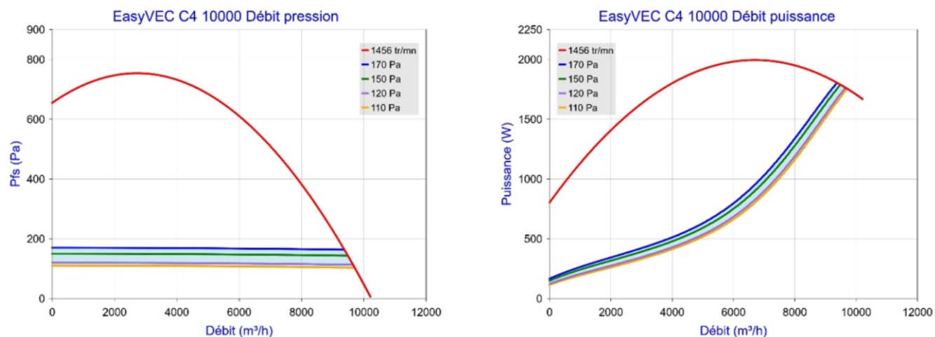
Figure 57 – EasyVEC C4 10000 (avec ou sans T.Flow Hygro+/T.Flow Nano ou T.Flow 105 / T.Flow 180)
