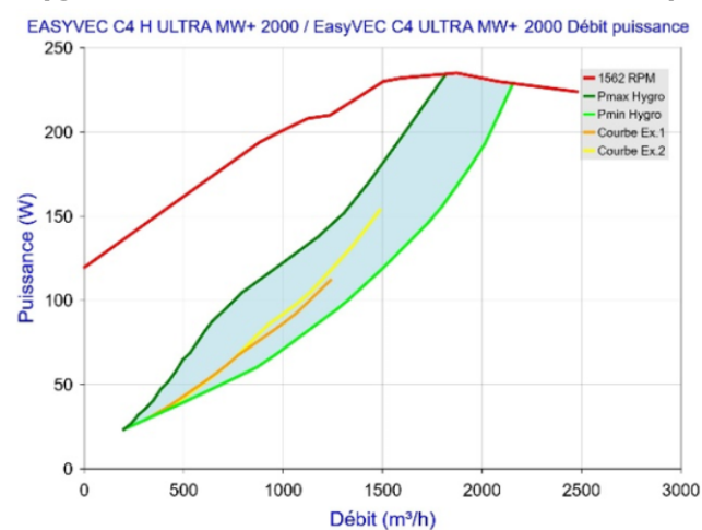
Figure 86 - EasyVEC C4 (H) ULTRA MW+ 2000 (sans T.Flow Hygro+/T.Flow Nano ou T.Flow 105 / T.Flow 180)
