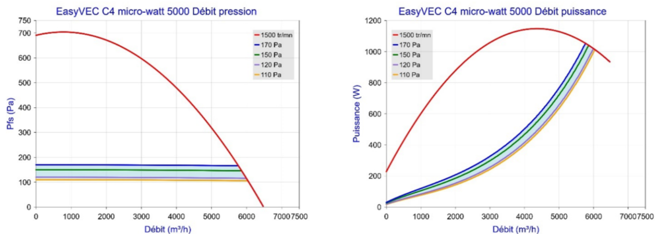
Figure 59 – EasyVEC C4 micro-watt 5000 (avec ou sans T.Flow Hygro+/T.Flow Nano ou T.Flow 105 / T.Flow 180)
