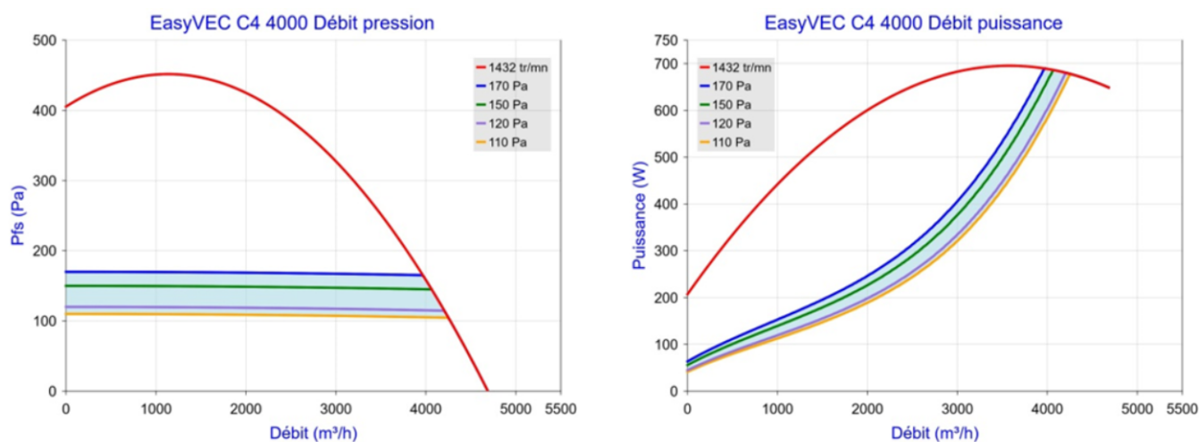
Figure 53 - EasyVEC C4 4000 (avec ou sans T.Flow Hygro+/T.Flow Nano ou T.Flow 105 / T.Flow 180)
