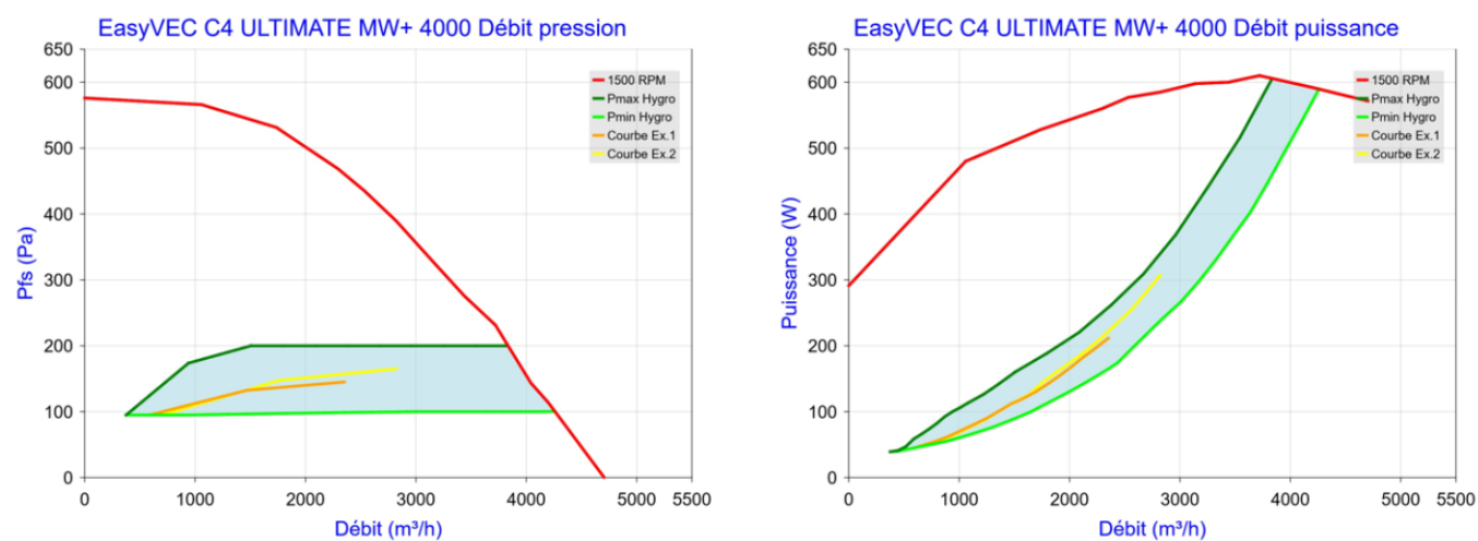
Figure 105 - EasyVEC C4 ULTIMATE MW+ 4000 (sans T.Flow Hygro+/T.Flow Nano ou T.Flow 105 / T.Flow 180)
