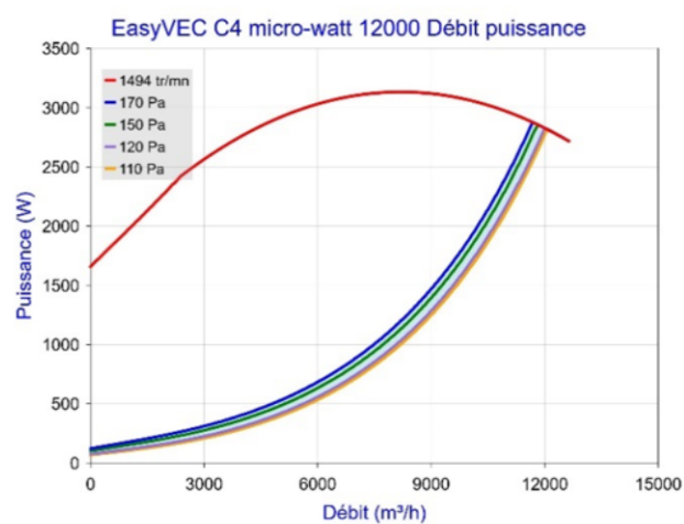
Figure 63 – EasyVEC C4 micro-watt 12000 (avec ou sans T.Flow Hygro+/T.Flow Nano ou T.Flow 105 / T.Flow 180)
