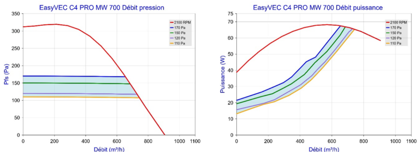
Figure 75 – EasyVEC C4 PRO MW 700 (avec ou sans T.Flow Hygro+/T.Flow Nano ou T.Flow 105 / T.Flow 180)
