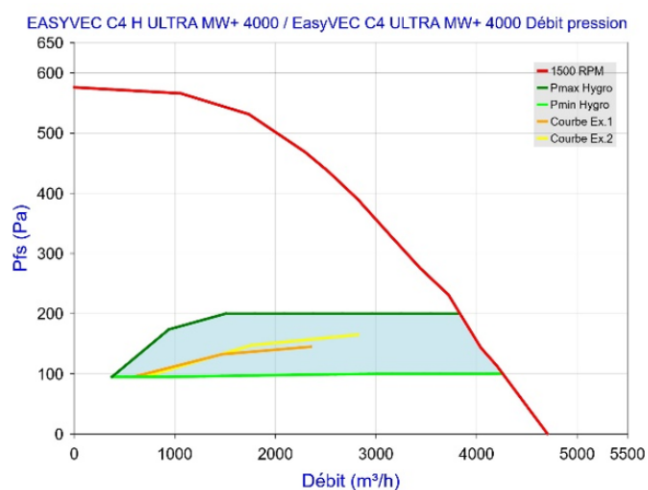
Figure 89 - EasyVEC C4 (H) ULTRA MW+ 4000 (sans T.Flow Hygro+/T.Flow Nano ou T.Flow 105 / T.Flow 180)
