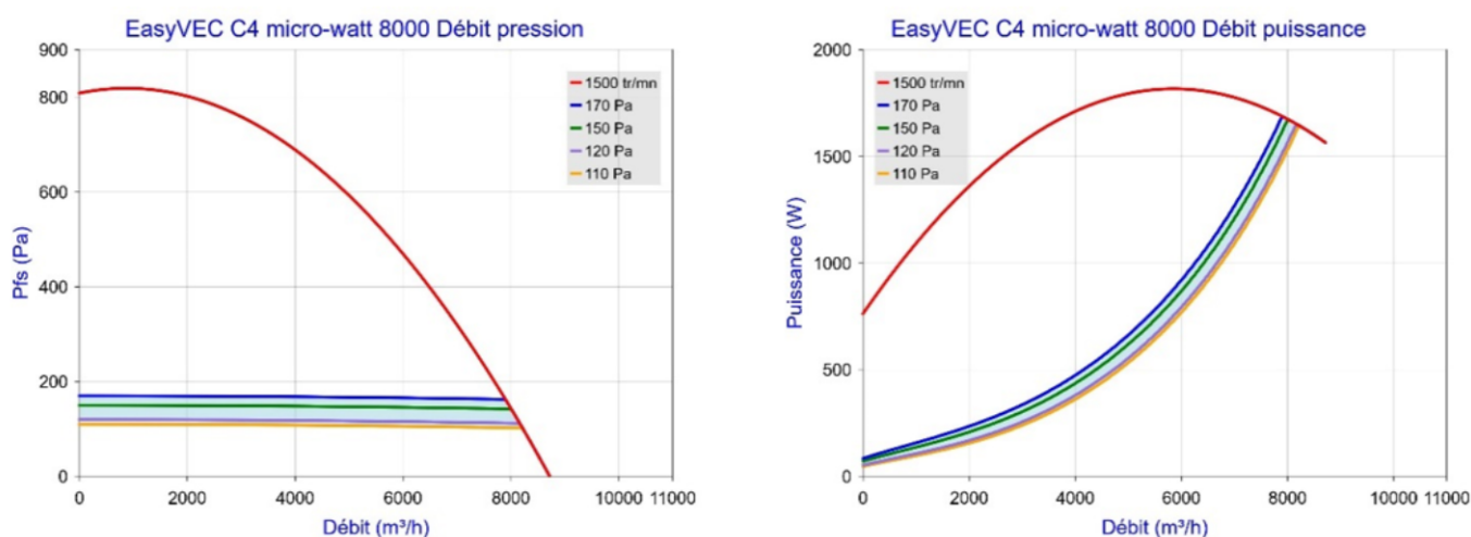
Figure 61 – EasyVEC C4 micro-watt 8000 (avec ou sans T.Flow Hygro+/T.Flow Nano ou T.Flow 105 / T.Flow 180)
