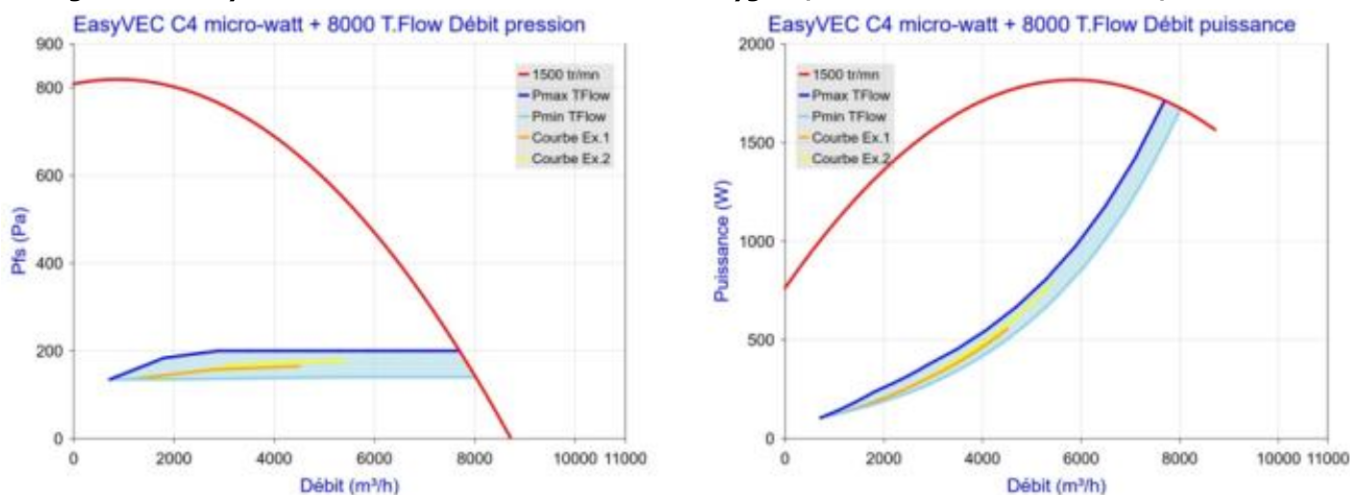
Figure 71 - EasyVEC C4 micro-watt + 8000 avec T.Flow Hygro+ / T.Flow Nano ou T.Flow 105 / T.Flow 180
