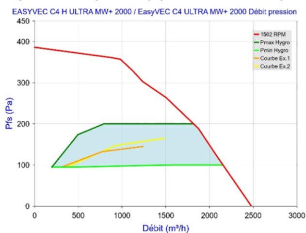
Figure 86 - EasyVEC C4 (H) ULTRA MW+ 2000 (sans T.Flow Hygro+/T.Flow Nano ou T.Flow 105 / T.Flow 180)
