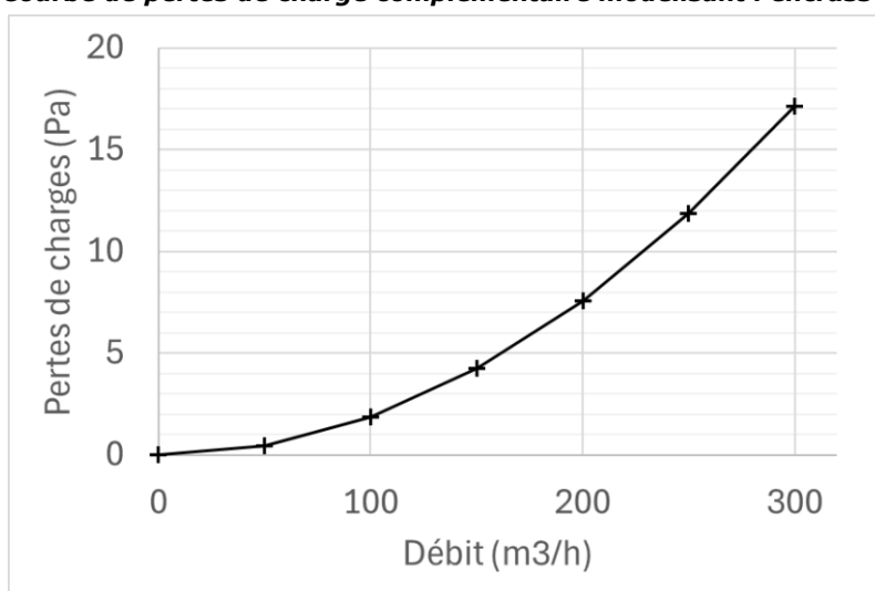
Figure 121 – Pertes de charge du caisson de répartition
