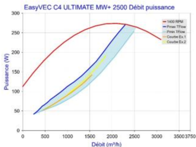
Figure 111 - EasyVEC C4 ULTIMATE MW+ 2500 avec T.Flow Hygro+/T.Flow Nano ou T.Flow 105 / T.Flow 180
