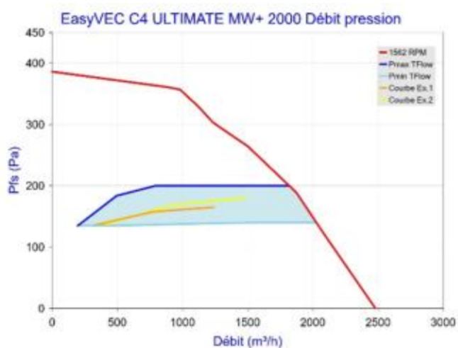
Figure 110 - EasyVEC C4 ULTIMATE MW+ 2000 avec T.Flow Hygro+/T.Flow Nano ou T.Flow 105 / T.Flow 180
