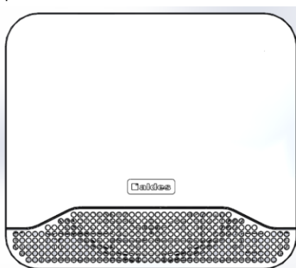
Figure 10 – Entrée d'air hygroréglable EHT 2
