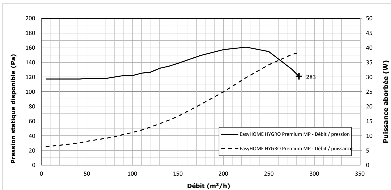
Figure 58 - Groupe d'extraction « EasyHOME HYGRO Premium MP » - courbes caractéristiques
