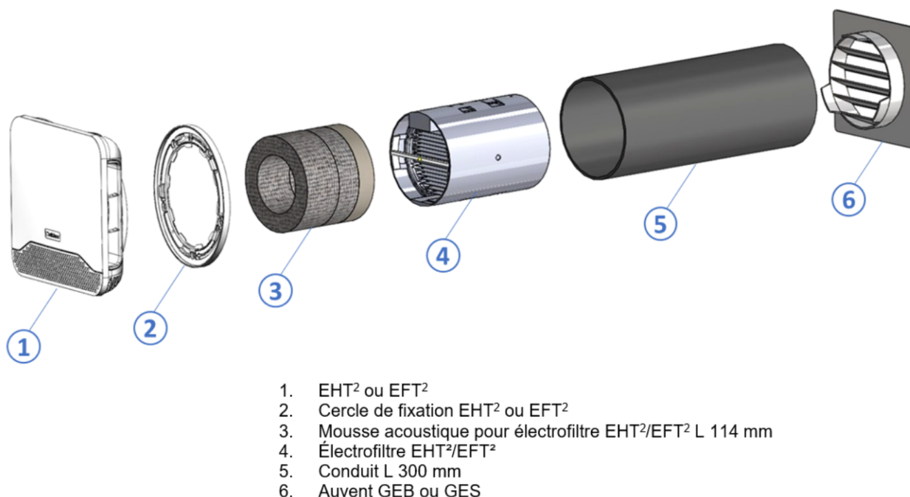
Figure 28 – Mise en œuvre entrée d'air EHT² ou EFT² avec électrofiltre EHT²/EFT² Ø 125 mm L 300 mm
