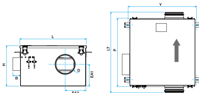
Encombrements PROVEC Compact Silence
