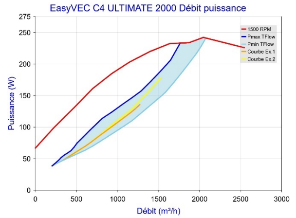
Figure 63 - EasyVEC C4 ULTIMATE 2000 avec T.Flow Hygro+/T.Flow Nano
