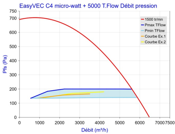
Figure 22 - EasyVEC C4 micro-watt + 5000 avec T.Flow Hygro+ / T.Flow Nano
