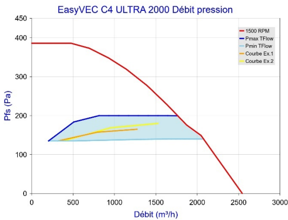
Figure 47 - EasyVEC C4 ULTRA 2000 avec T.Flow Hygro+ / T.Flow Nano
