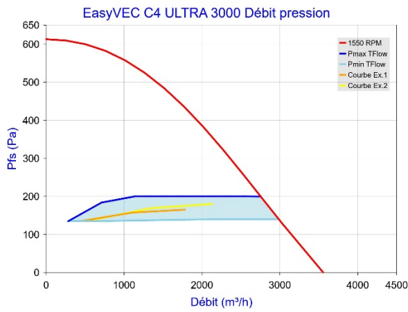
Figure 49 - EasyVEC C4 ULTRA 3000 avec T.Flow Hygro+ / T.Flow Nano
