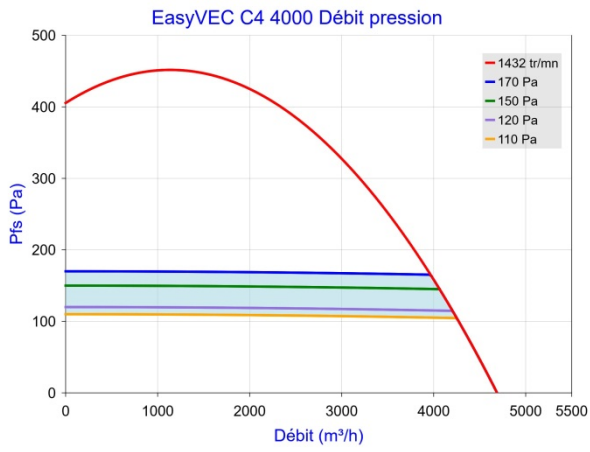
Figure 6 – EasyVEC C4 4000 (avec ou sans T.Flow Hygro+ /T.Flow Nano)
