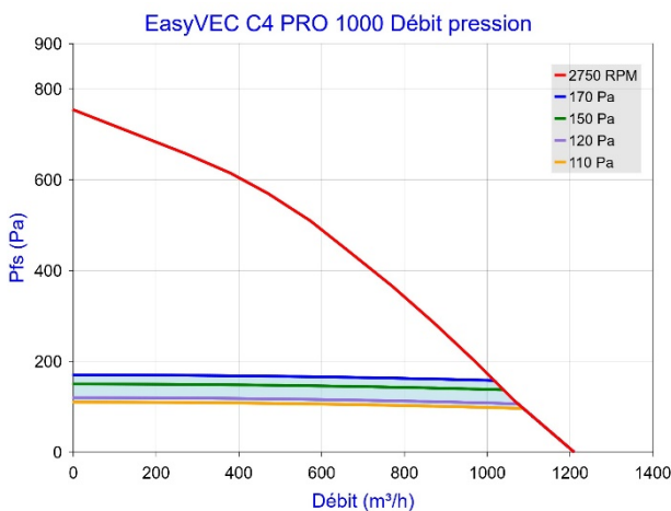
Figure 29 – EasyVEC C4 PRO 1000 (avec ou sans T.Flow Hygro+ /T.Flow Nano)
