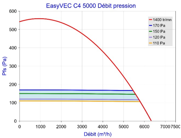
Figure 7 – EasyVEC C4 5000 (avec ou sans T.Flow Hygro+ /T.Flow Nano)
