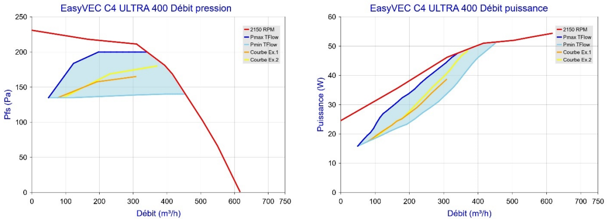
Figure 43 - EasyVEC C4 ULTRA 400 avec T.Flow Hygro+ / T.Flow Nano
