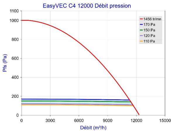
Figure 11 – EasyVEC C4 12 000 (avec ou sans T.Flow Hygro+ /T.Flow Nano)
