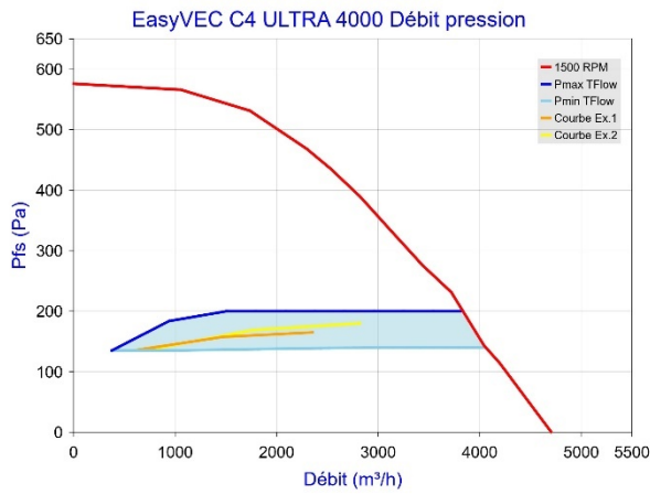
Figure 50 - EasyVEC C4 ULTRA 4000 avec T.Flow Hygro+ / T.Flow Nano
