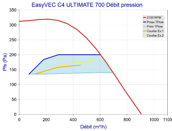
Figure 60 - EasyVEC C4 ULTIMATE 700 avec T.Flow Hygro+ /T.Flow Nano
