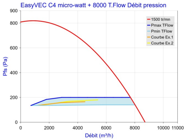
Figure 24 - EasyVEC C4 micro-watt + 8000 avec T.Flow Hygro+/ T.Flow Nano
