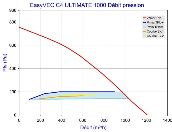
Figure 61 - EasyVEC C4 ULTIMATE 1000 avec T.Flow Hygro+ /T.Flow Nano
