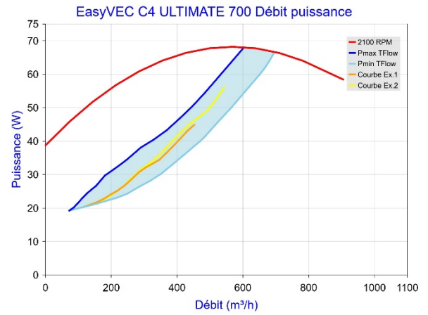
Figure 60 - EasyVEC C4 ULTIMATE 700 avec T.Flow Hygro+ /T.Flow Nano
