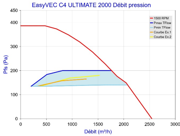
Figure 63 - EasyVEC C4 ULTIMATE 2000 avec T.Flow Hygro+/T.Flow Nano
