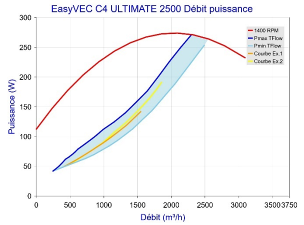
Figure 64 - EasyVEC C4 ULTIMATE 2500 avec T.Flow Hygro+/T.Flow Nano
