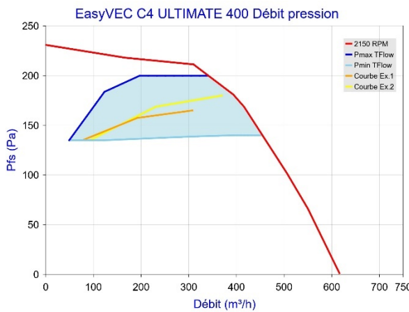
Figure 59 - EasyVEC C4 ULTIMATE 400 avec T.Flow Hygro+ /T.Flow Nano
