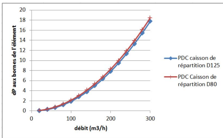
Figure 6 – application « T.Flow Hygro + » - Pertes de charge du caisson de répartition
