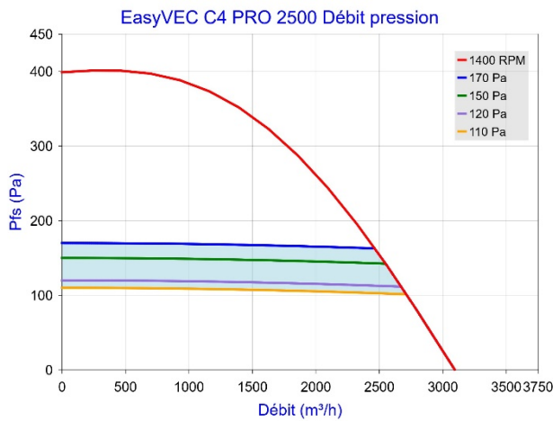
Figure 32 – EasyVEC C4 PRO 2500 (avec ou sans T.Flow Hygro+ /T.Flow Nano)
