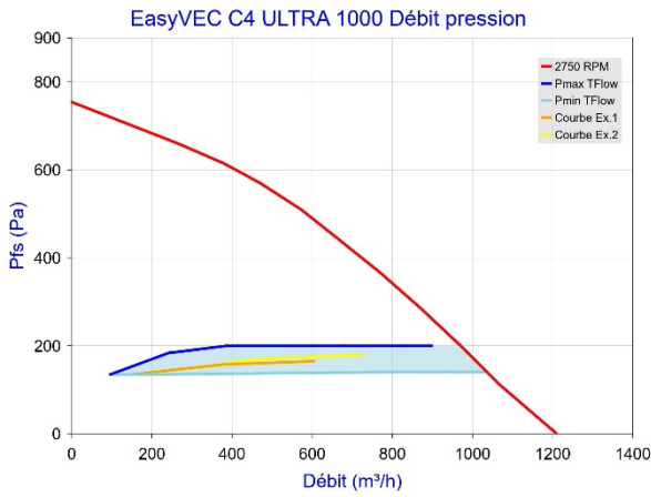
Figure 45 - EasyVEC C4 ULTRA 1000 avec T.Flow Hygro+ / T.Flow Nano
