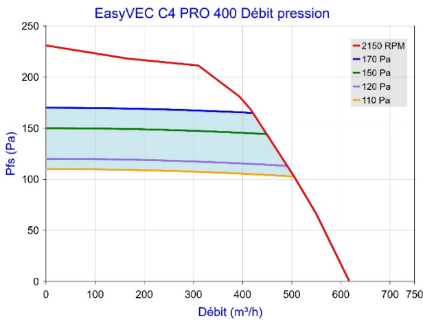
Figure 27 – EasyVEC C4 PRO 400 (avec ou sans T.Flow Hygro+ /T.Flow Nano)
