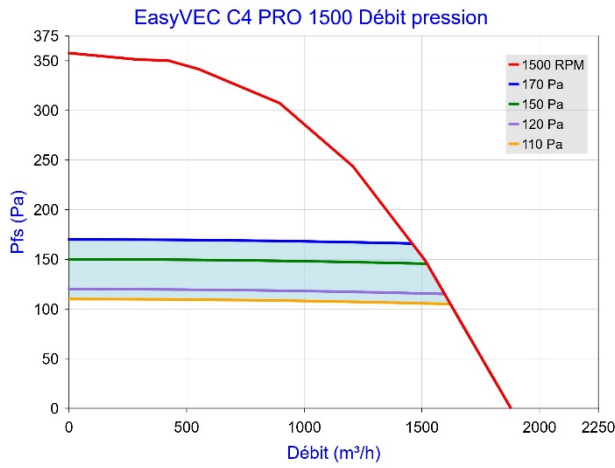
Figure 30 – EasyVEC C4 PRO 1500 (avec ou sans T.Flow Hygro+ /T.Flow Nano)
