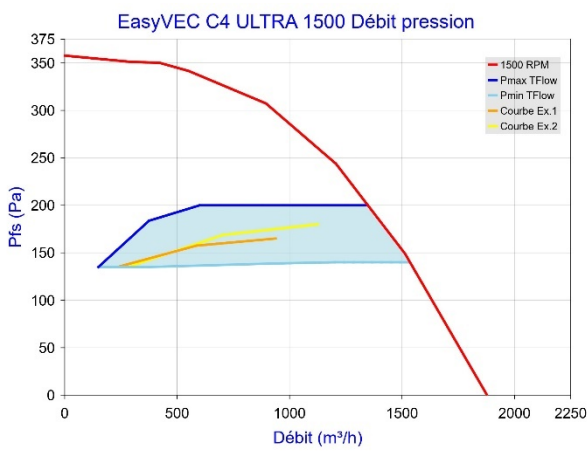
Figure 46 - EasyVEC C4 ULTRA 1500 avec T.Flow Hygro+ / T.Flow Nano
