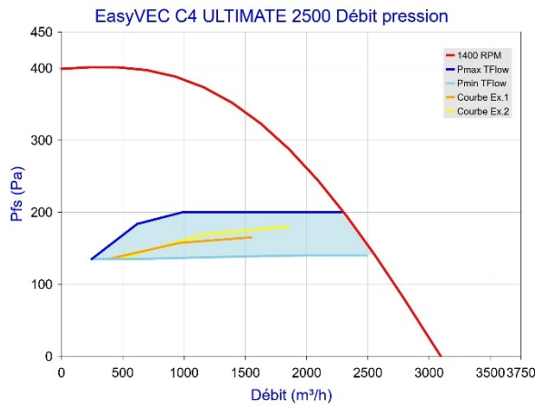
Figure 64 - EasyVEC C4 ULTIMATE 2500 avec T.Flow Hygro+/T.Flow Nano
