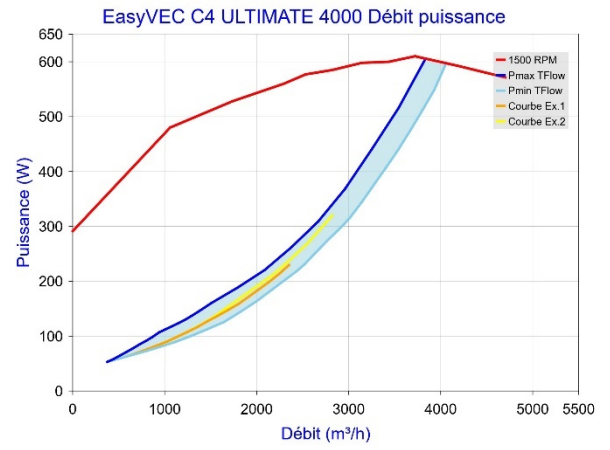
Figure 66 - EasyVEC C4 ULTIMATE 4000 avec T.Flow Hygro+/T.Flow Nano
