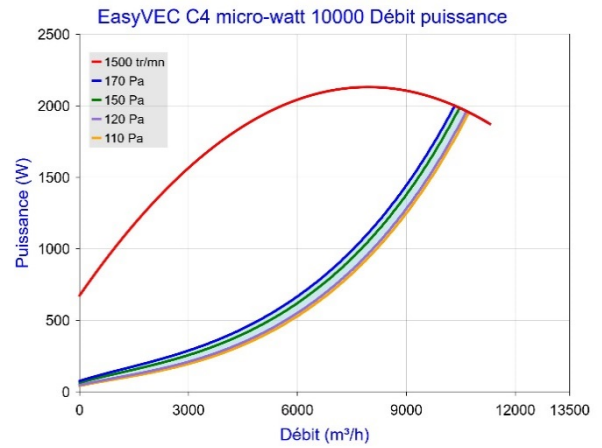
Figure 15 – EasyVEC C4 micro-watt 10000 (avec ou sans T.Flow Hygro+ /T.Flow Nano)
