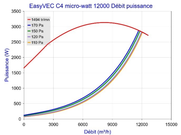
Figure 16 – EasyVEC C4 micro-watt 12000 (avec ou sans T.Flow Hygro+ /T.Flow Nano)
