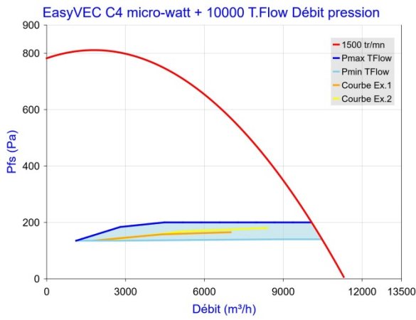
Figure 25 - EasyVEC C4 micro-watt + 10000 avec T.Flow Hygro+/ T.Flow Nano
