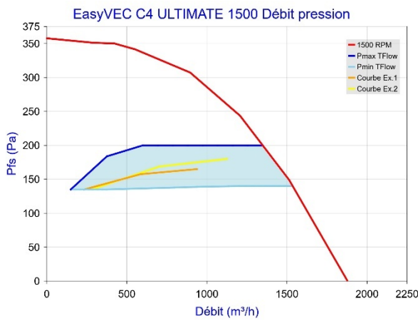
Figure 62 - EasyVEC C4 ULTIMATE 1500 avec T.Flow Hygro+ /T.Flow Nano
