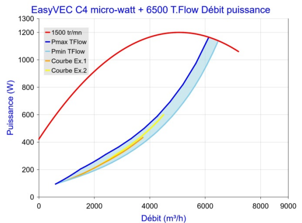
Figure 23 - EasyVEC C4 micro-watt + 6500 avec T.Flow Hygro+ / T.Flow Nano
