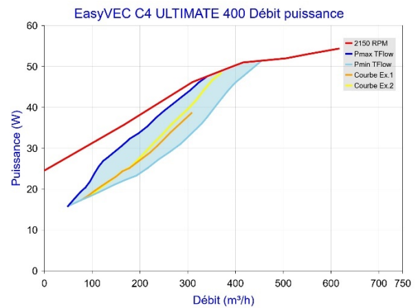
Figure 59 - EasyVEC C4 ULTIMATE 400 avec T.Flow Hygro+ /T.Flow Nano
