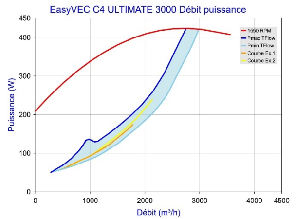
Figure 65 - EasyVEC C4 ULTIMATE 3000 avec T.Flow Hygro+/T.Flow Nano
