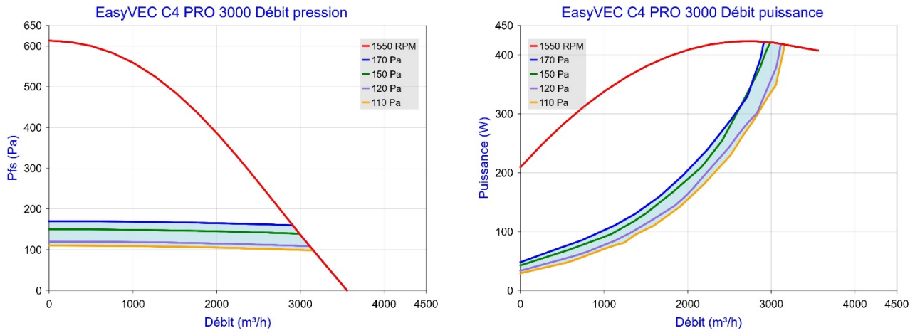
Figure 33 – EasyVEC C4 PRO 3000 (avec ou sans T.Flow Hygro+ /T.Flow Nano)
