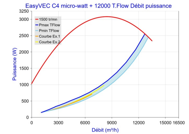
Figure 26 - EasyVEC C4 micro-watt + 12000 avec T.Flow Hygro+/ T.Flow Nano
