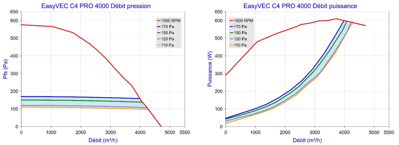
Figure 34 – EasyVEC C4 PRO 4000 (avec ou sans T.Flow Hygro+ /T.Flow Nano)
