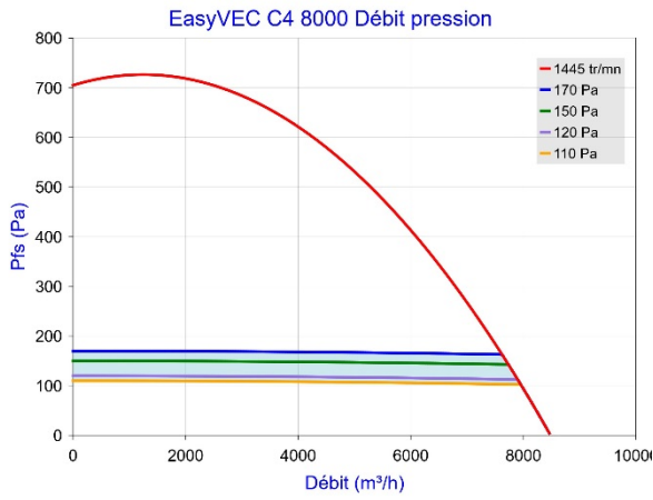
Figure 9 – EasyVEC C4 8000 (avec ou sans T.Flow Hygro+ /T.Flow Nano)
