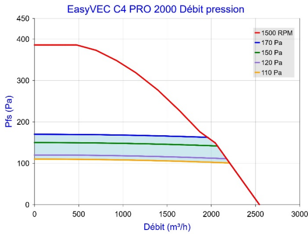
Figure 31 – EasyVEC C4 PRO 2000 (avec ou sans T.Flow Hygro+ /T.Flow Nano)
