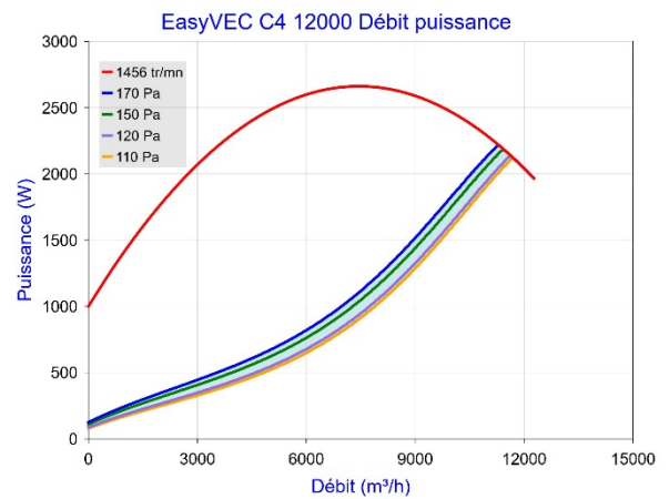
Figure 11 – EasyVEC C4 12 000 (avec ou sans T.Flow Hygro+ /T.Flow Nano)
