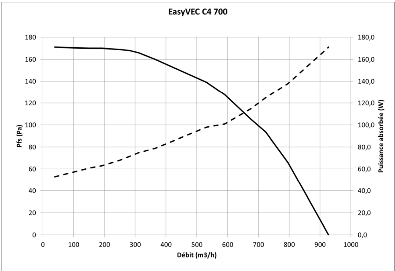
Figure 2 - EasyVEC C4 700 (avec ou sans T.Flow Hygro+ /T.Flow Nano)
