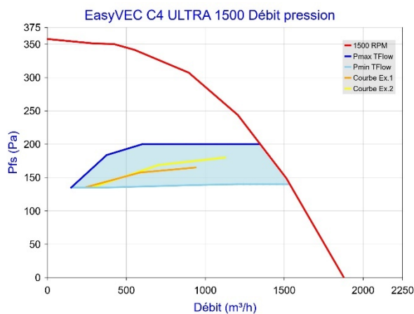
Figure 46 - EasyVEC C4 ULTRA 1500 avec T.Flow Hygro+ / T.Flow Nano
