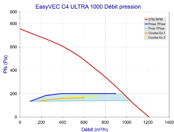
Figure 45 - EasyVEC C4 ULTRA 1000 avec T.Flow Hygro+ / T.Flow Nano
