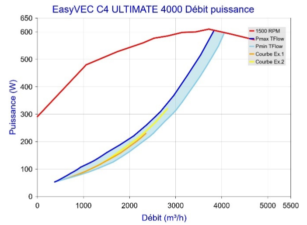
Figure 66 - EasyVEC C4 ULTIMATE 4000 avec T.Flow Hygro+ / T.Flow Nano
