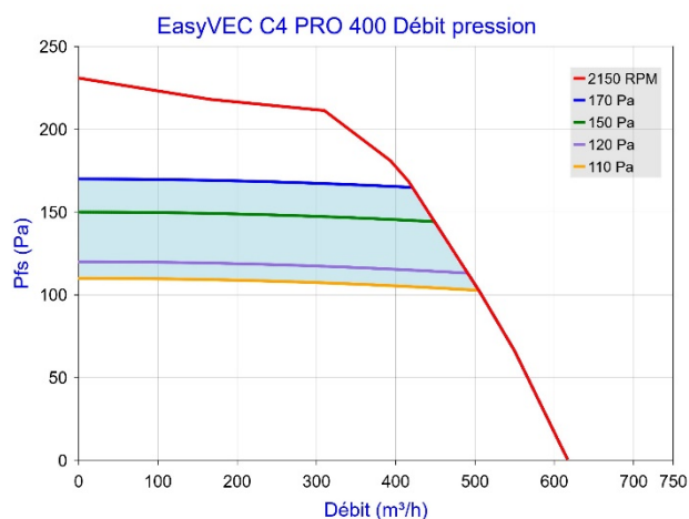
Figure 27 – EasyVEC C4 PRO 400 (avec ou sans T.Flow Hygro+ / T.Flow Nano)
