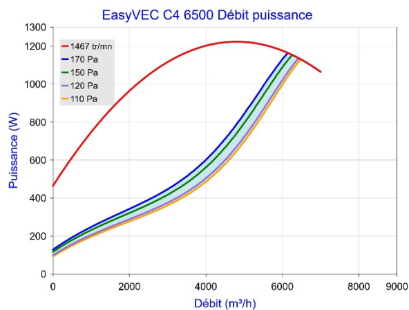
Figure 8 – EasyVEC C4 6500 (avec ou sans T.Flow Hygro+ / T.Flow Nano)
