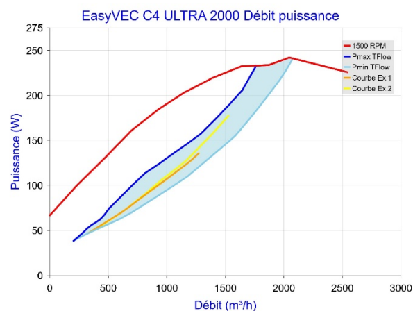
Figure 47 - EasyVEC C4 ULTRA 2000 avec T.Flow Hygro+ / T.Flow Nano
