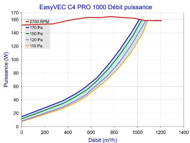
Figure 29 – EasyVEC C4 PRO 1000 (avec ou sans T.Flow Hygro+ / T.Flow Nano)
