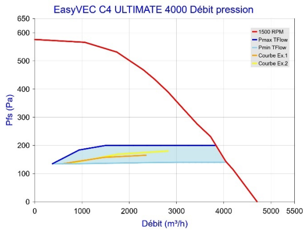
Figure 66 - EasyVEC C4 ULTIMATE 4000 avec T.Flow Hygro+ / T.Flow Nano
