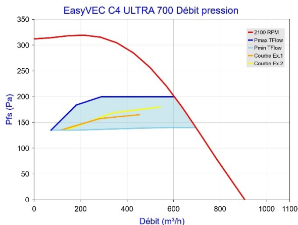
Figure 44 - EasyVEC C4 ULTRA 700 avec T.Flow Hygro+ / T.Flow Nano
