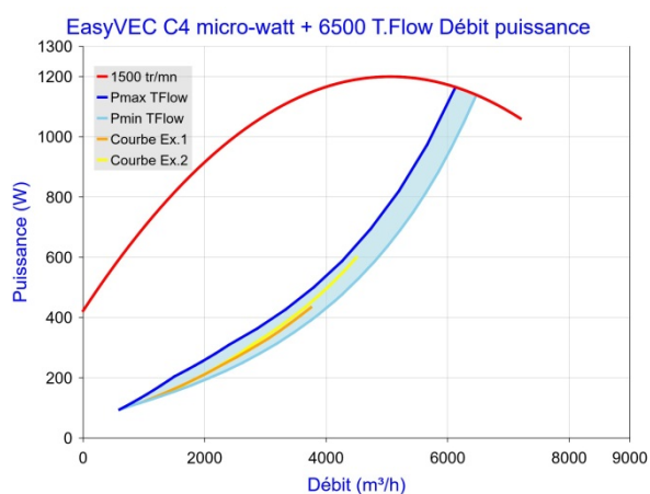
Figure 23 - EasyVEC C4 micro-watt + 6500 avec T.Flow Hygro+ / T.Flow Nano
