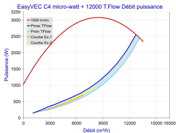
Figure 26 - EasyVEC C4 micro-watt + 12000 avec T.Flow Hygro+ / T.Flow Nano
