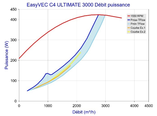
Figure 65 - EasyVEC C4 ULTIMATE 3000 avec T.Flow Hygro+ / T.Flow Nano
