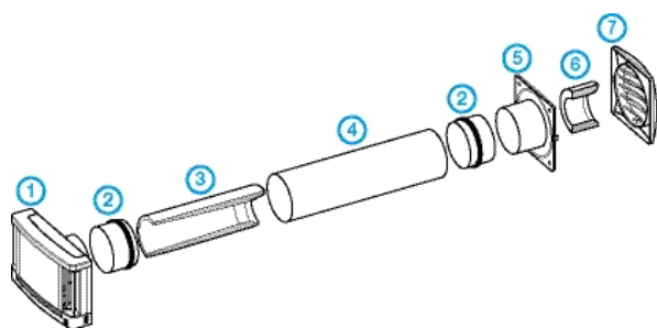
Figure 22 – Mise en œuvre entrée d'air EHT
