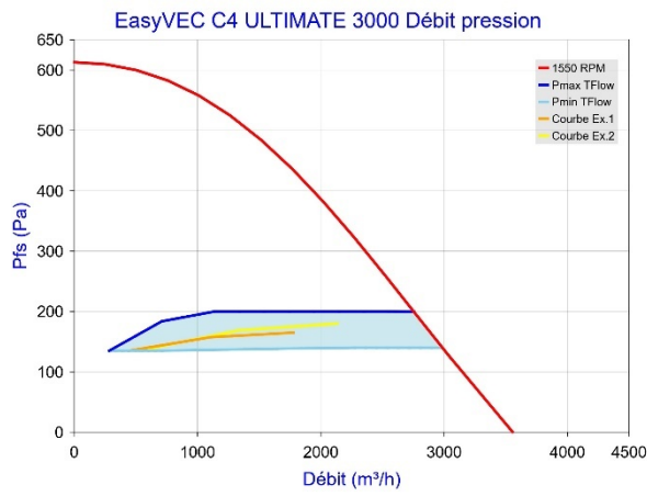
Figure 65 - EasyVEC C4 ULTIMATE 3000 avec T.Flow Hygro+ / T.Flow Nano
