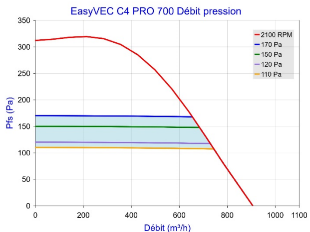
Figure 28 – EasyVEC C4 PRO 700 (avec ou sans T.Flow Hygro+ / T.Flow Nano)
