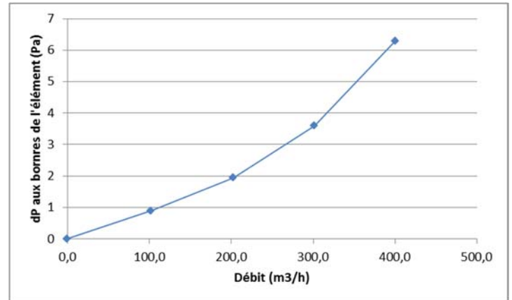
Figure 5 – Courbe de pertes de charge complémentaire modélisant l'encrassement du filtre
