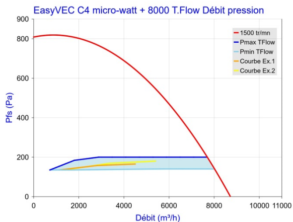
Figure 24 - EasyVEC C4 micro-watt + 8000 avec T.Flow Hygro+ / T.Flow Nano
