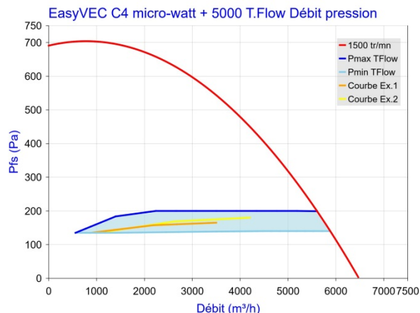
Figure 22 - EasyVEC C4 micro-watt + 5000 avec T.Flow Hygro+ / T.Flow Nano
