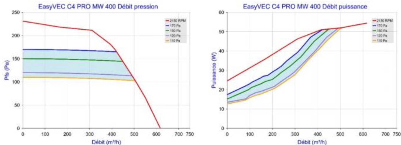
Figure 74 – EasyVEC C4 PRO MW 400 (avec ou sans T.Flow Hygro+/T.Flow Nano)
