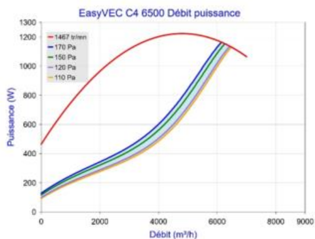
Figure 55 – EasyVEC C4 6500 (avec ou sans T.Flow Hygro+/T.Flow Nano)
