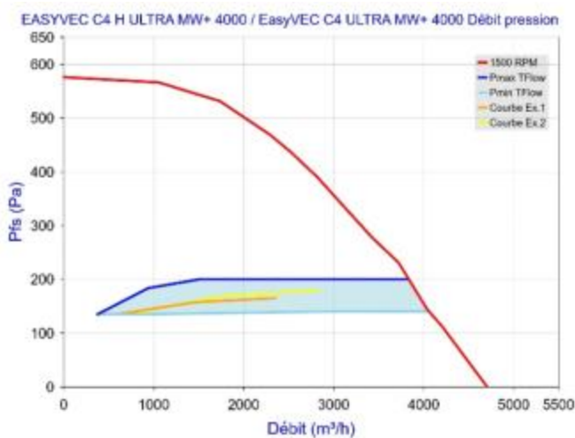
Figure 97 - EasyVEC C4 (H) ULTRA MW+ 4000 avec T.Flow Hygro+/ T.Flow Nano
