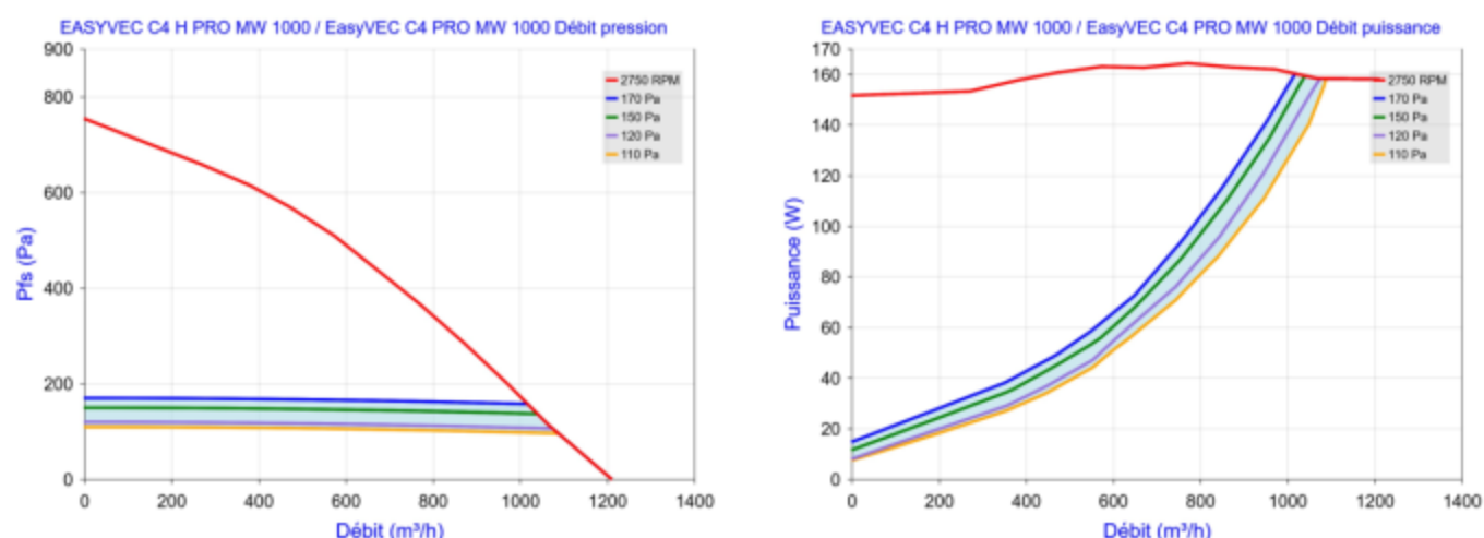
Figure 76 – EasyVEC C4 (H) PRO MW 1000 (avec ou sans T.Flow Hygro+/T.Flow Nano)
