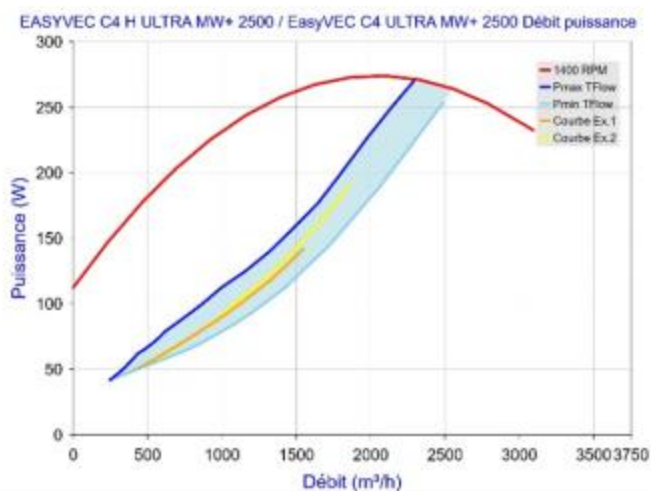
Figure 95 - EasyVEC C4 (H) ULTRA MW+ 2500 avec T.Flow Hygro+/ T.Flow Nano
