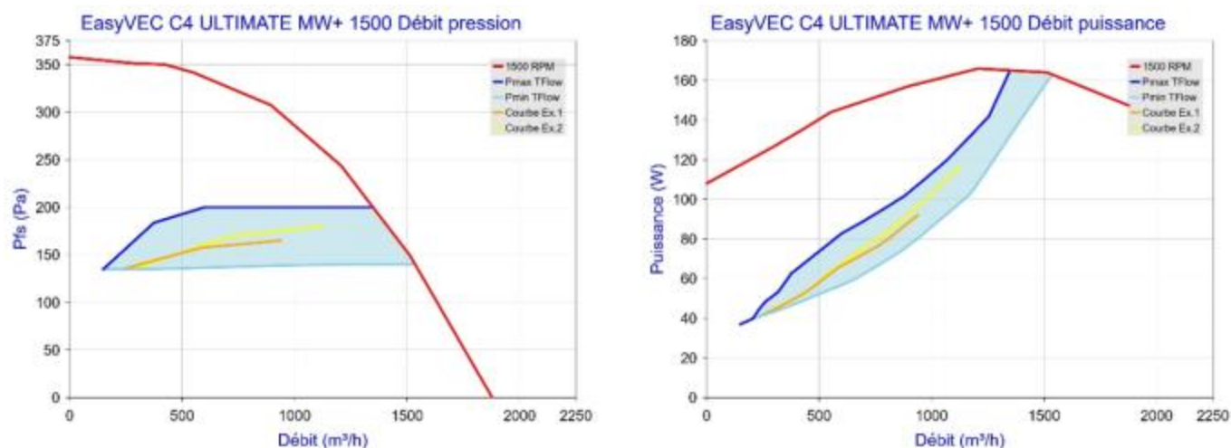
Figure 109 - EasyVEC C4 ULTIMATE MW+ 1500 avec T.Flow Hygro+/T.Flow Nano
