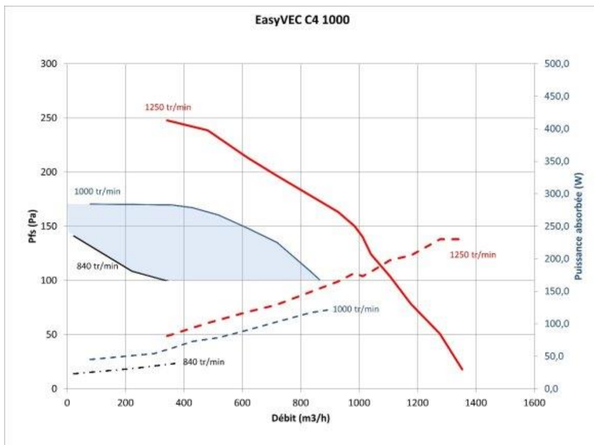
Figure 50 - EasyVEC C4 1000 (avec ou sans T.Flow Hygro+/T.Flow Nano)
