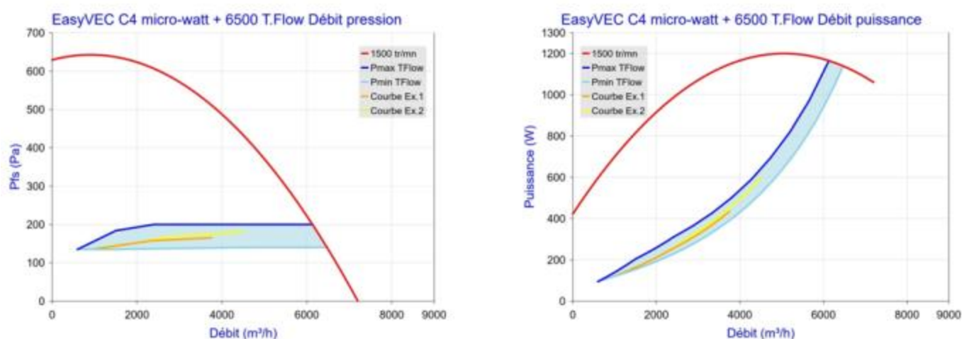
Figure 70 - EasyVEC C4 micro-watt + 6500 avec T.Flow Hygro+/ T.Flow Nano
