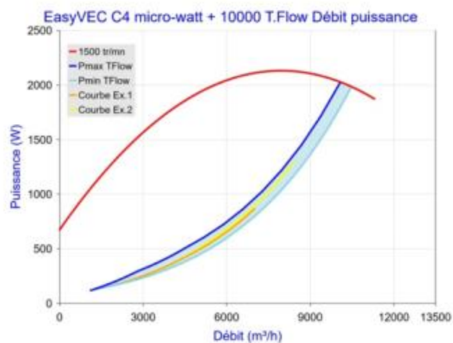
Figure 72 - EasyVEC C4 micro-watt + 10000 avec T.Flow Hygro+/ T.Flow Nano
