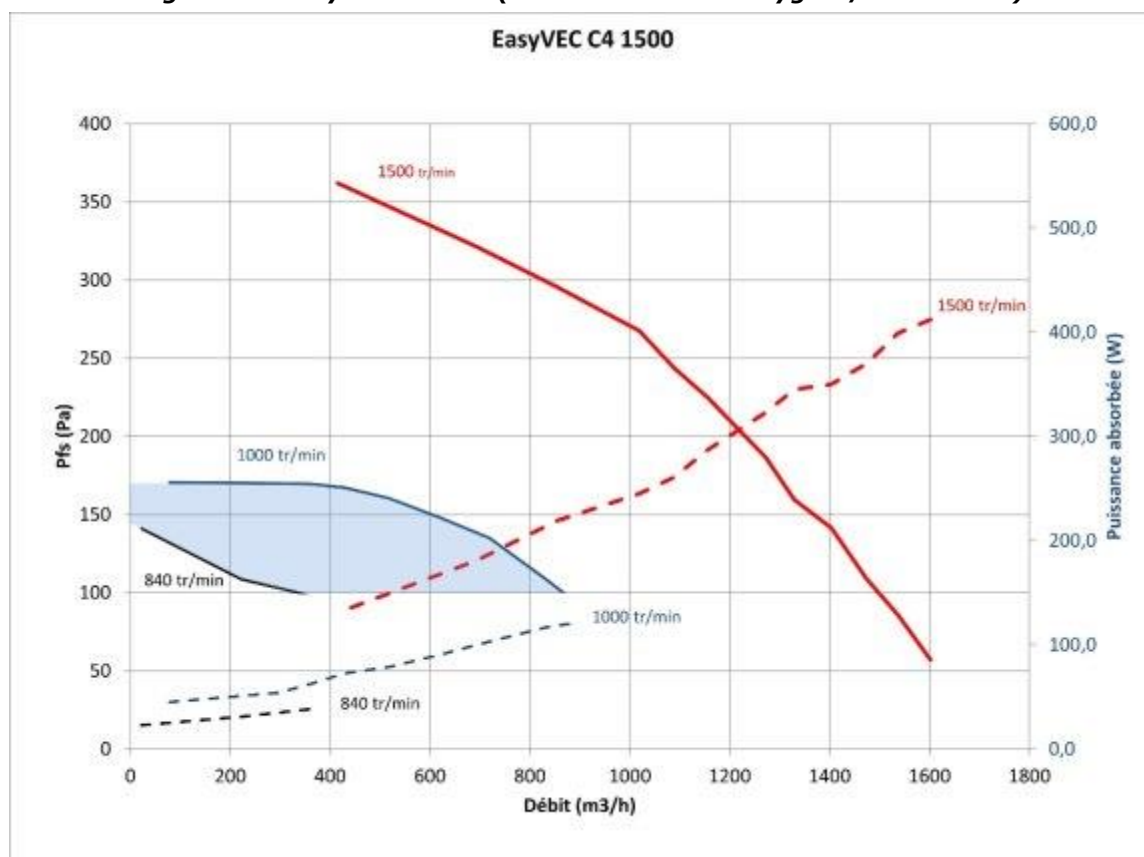
Figure 51 - EasyVEC C4 1500 (avec ou sans T.Flow Hygro+/T.Flow Nano)
