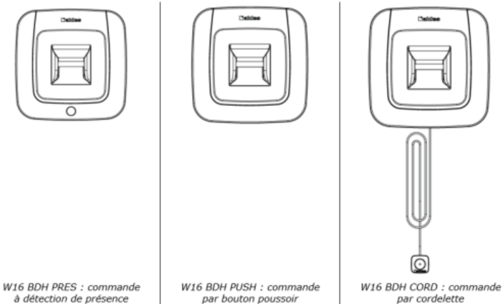
Figure 46 – Visuels des bouches fixes temporisées W16 (WC)
