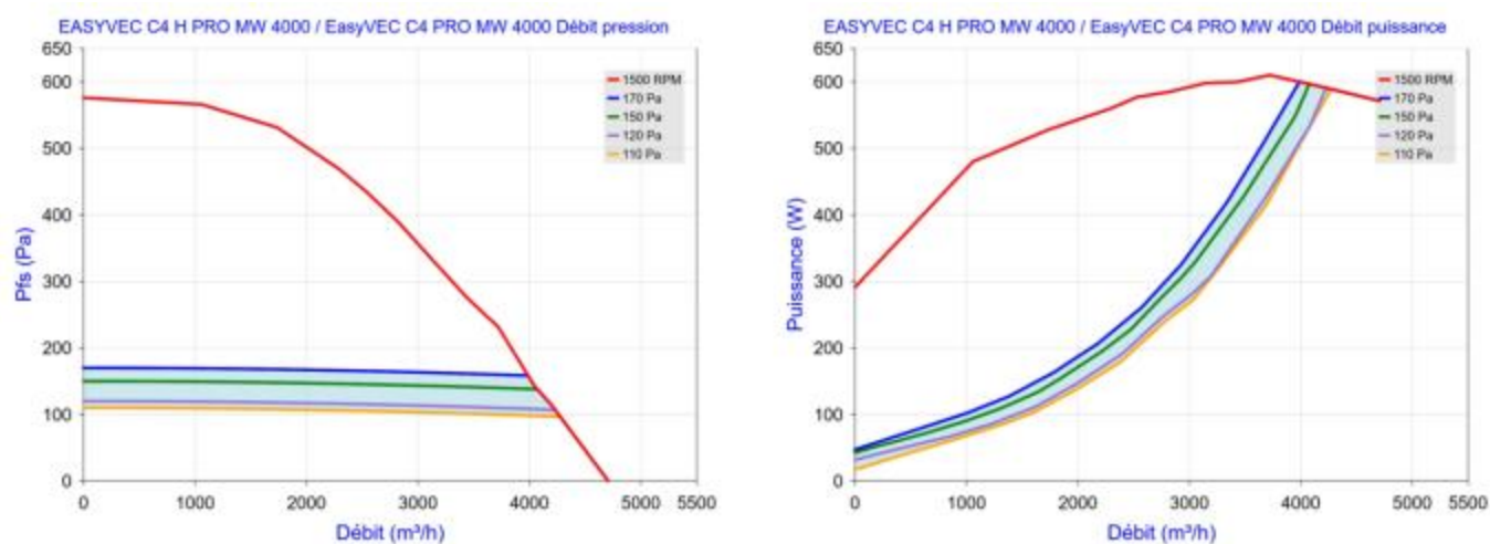
Figure 81 – EasyVEC C4 (H) PRO MW 4000 (avec ou sans T.Flow Hygro+/T.Flow Nano)
