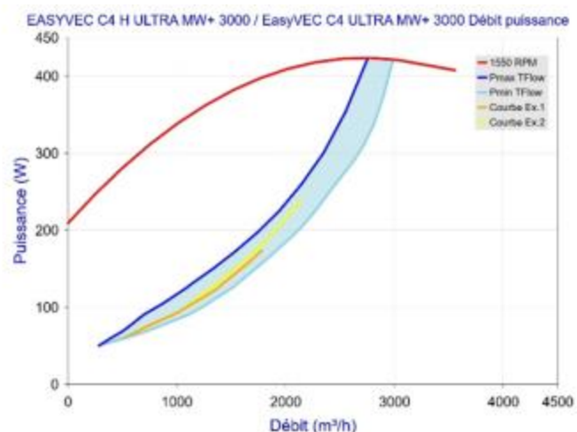
Figure 96 - EasyVEC C4 (H) ULTRA MW+ 3000 avec T.Flow Hygro+/T.Flow Nano
