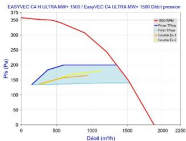
Figure 93 - EasyVEC C4 (H) ULTRA MW+ 1500 avec T.Flow Hygro+/T.Flow Nano
