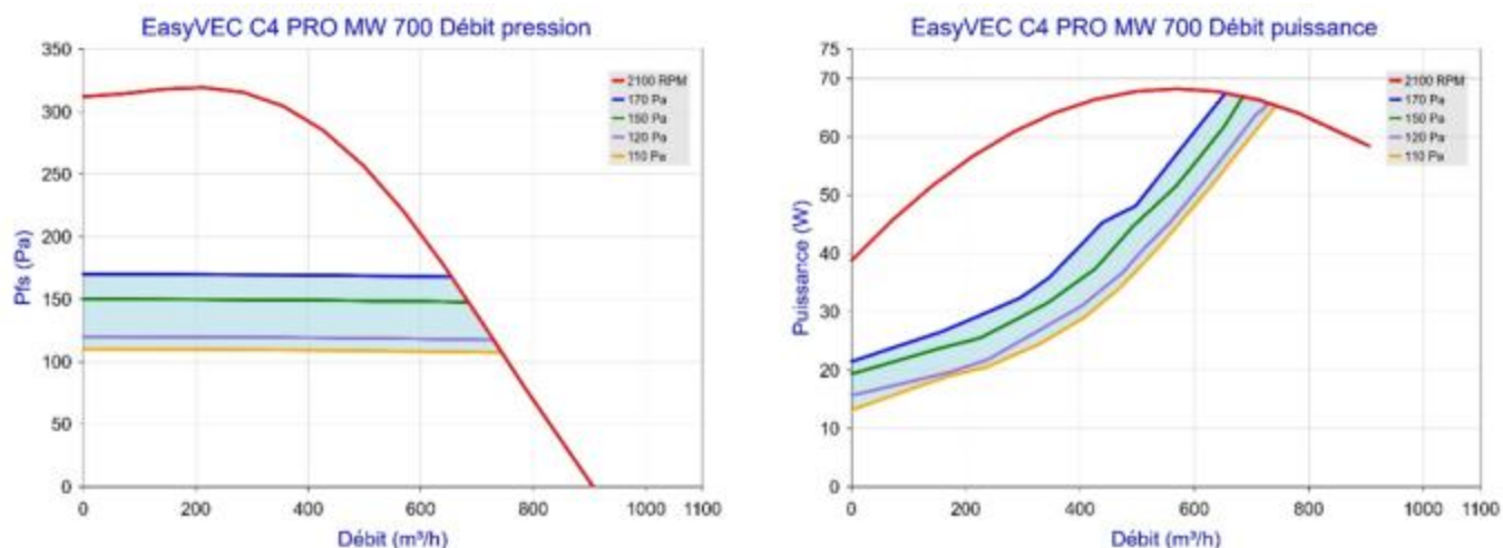
Figure 75 – EasyVEC C4 PRO MW 700 (avec ou sans T.Flow Hygro+/T.Flow Nano)
