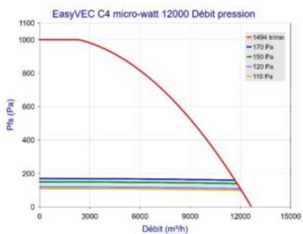
Figure 63 – EasyVEC C4 micro-watt 12000 (avec ou sans T.Flow Hygro+/T.Flow Nano)
