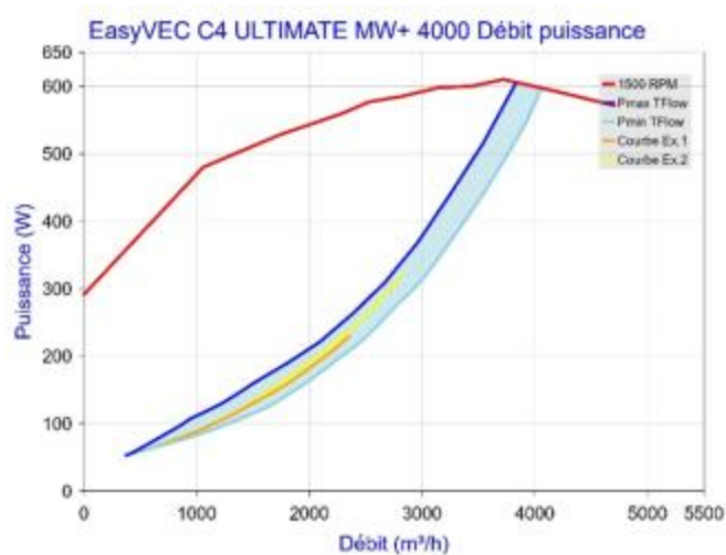
Figure 113 - EasyVEC C4 ULTIMATE MW+ 4000 avec T.Flow Hygro+/T.Flow Nano
