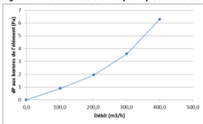
Figure 118 – Courbe de pertes de charge complémentaire modélisant l'encrassement du filtre
