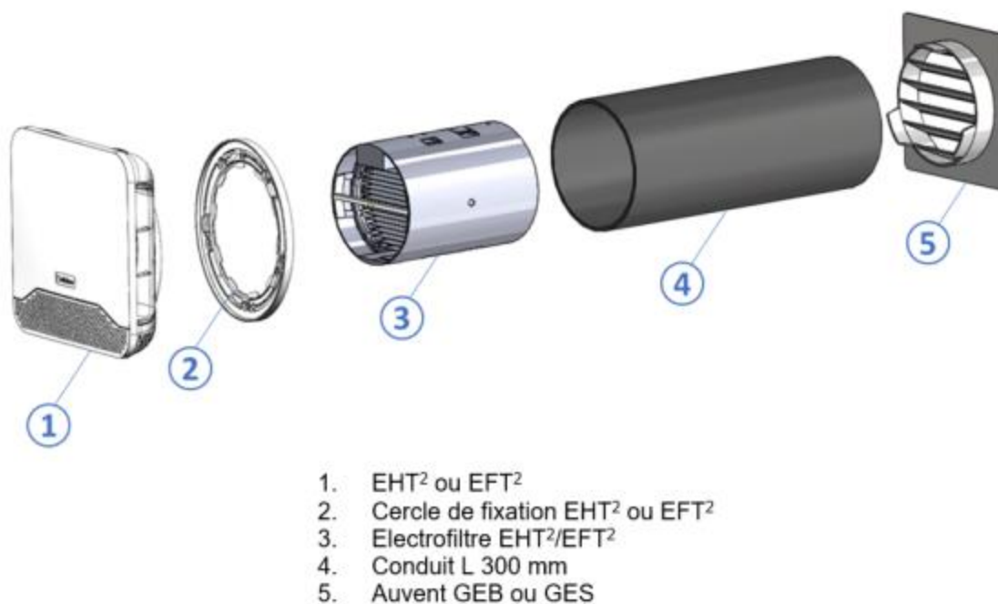
Figure 27 – Mise en œuvre entrée d'air EHT 2 ou EFT 2 avec électrofiltre EHT 2 /EFT 2 sans mousse Ø 125 mm L 300 mm
