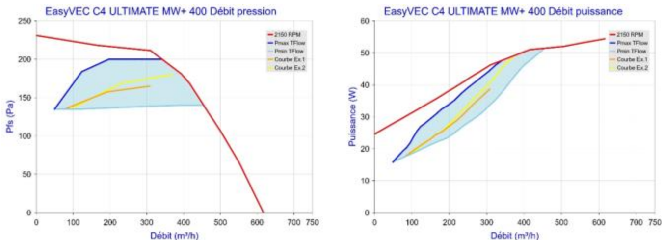
Figure 106 - EasyVEC C4 ULTIMATE MW+ 400 avec T.Flow Hygro+/T.Flow Nano
