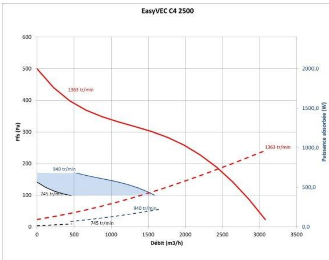
Figure 52 - EasyVEC C4 2500 (avec ou sans T.Flow Hygro+/T.Flow Nano)
