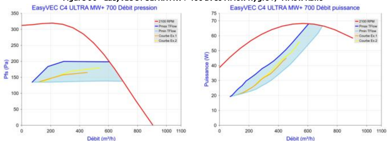
Figure 91 - EasyVEC C4 ULTRA MW+ 700 avec T.Flow Hygro+/T.Flow Nano
