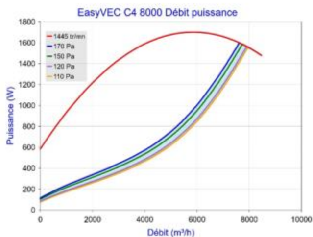
Figure 56 – EasyVEC C4 8000 (avec ou sans T.Flow Hygro+/T.Flow Nano)
