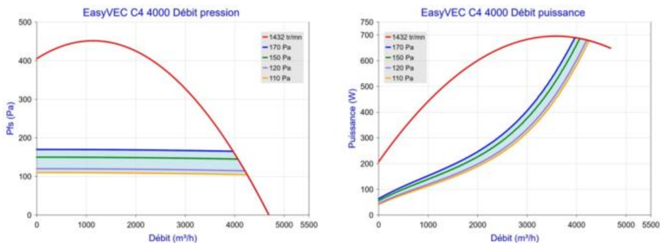
Figure 53 - EasyVEC C4 4000 (avec ou sans T.Flow Hygro+/T.Flow Nano)
