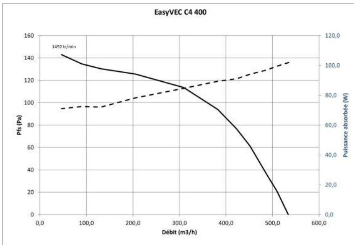
Figure 48 - EasyVEC C4 400 (avec ou sans T.Flow Hygro+/T.Flow Nano)
