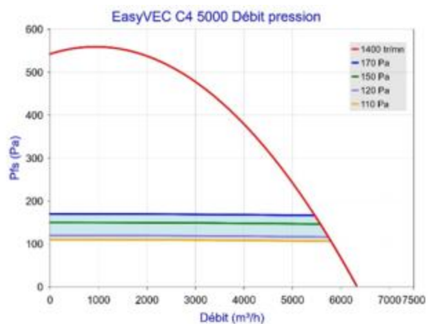
Figure 54 – EasyVEC C4 5000 (avec ou sans T.Flow Hygro+/T.Flow Nano)
