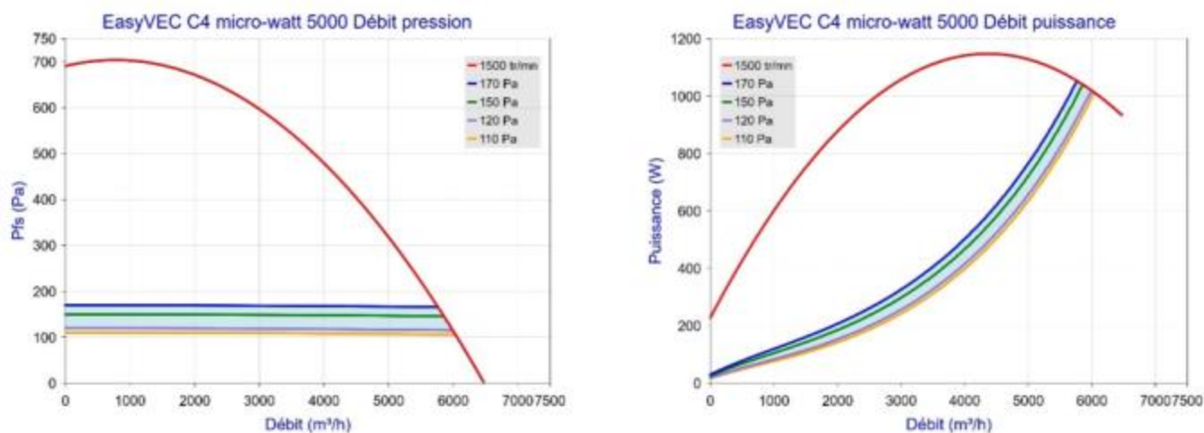
Figure 59 – EasyVEC C4 micro-watt 5000 (avec ou sans T.Flow Hygro+/T.Flow Nano)
