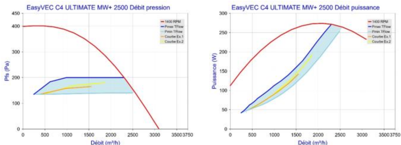
Figure 111 - EasyVEC C4 ULTIMATE MW+ 2500 avec T.Flow Hygro+/T.Flow Nano
