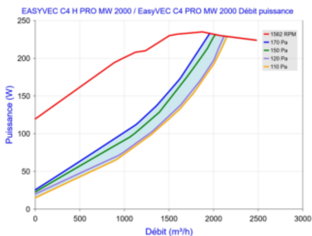
Figure 78 – EasyVEC C4 (H) PRO MW 2000 (avec ou sans T.Flow Hygro+/T.Flow Nano)
