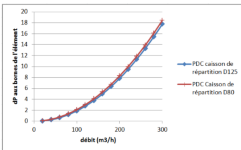
Figure 119 – Application « T.Flow Hygro+ » - Pertes de charge du caisson de répartition
