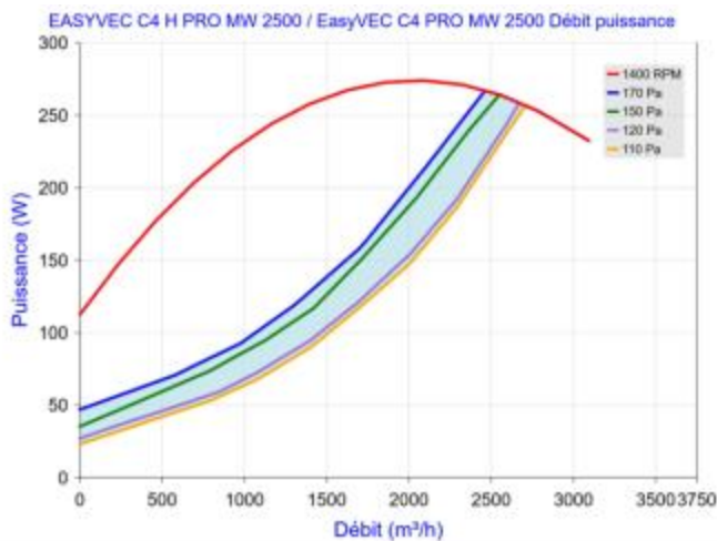
Figure 79 – EasyVEC C4 (H) PRO MW 2500 (avec ou sans T.Flow Hygro+/T.Flow Nano)
