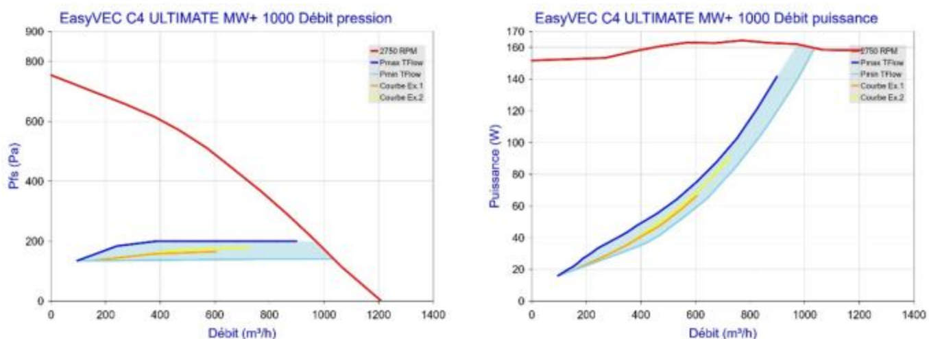
Figure 108 - EasyVEC C4 ULTIMATE MW+ 1000 avec T.Flow Hygro+/T.Flow Nano
