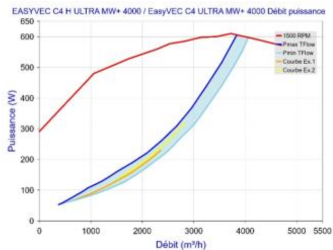
Figure 97 - EasyVEC C4 (H) ULTRA MW+ 4000 avec T.Flow Hygro+/ T.Flow Nano
