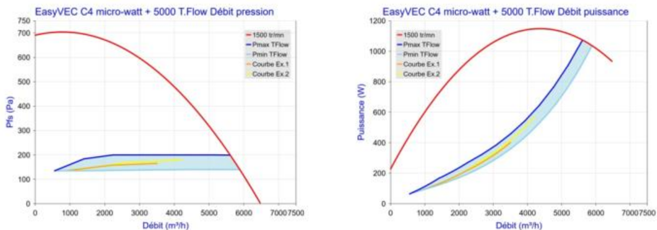
Figure 69 - EasyVEC C4 micro-watt + 5000 avec T.Flow Hygro+/ T.Flow Nano
