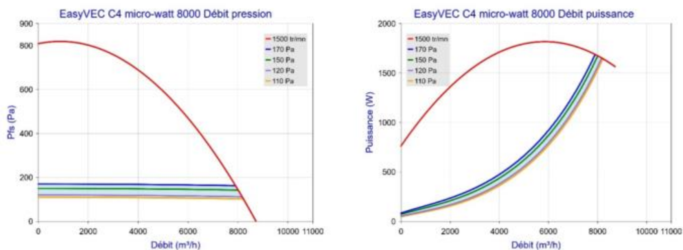
Figure 61 – EasyVEC C4 micro-watt 8000 (avec ou sans T.Flow Hygro+/T.Flow Nano)
