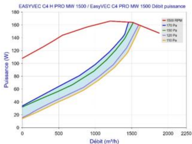
Figure 77 – EasyVEC C4 (H) PRO MW 1500 (avec ou sans T.Flow Hygro+/T.Flow Nano)
