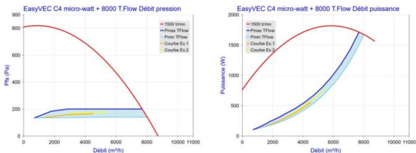
Figure 71 - EasyVEC C4 micro-watt + 8000 avec T.Flow Hygro+/ T.Flow Nano
