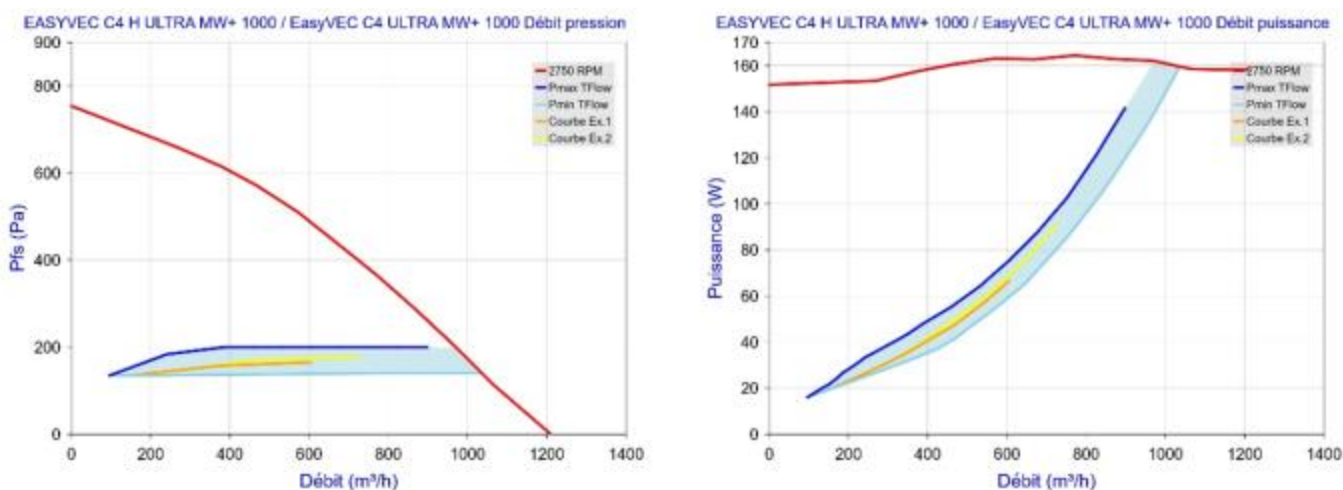
Figure 92 - EasyVEC C4 (H) ULTRA MW+ 1000 avec T.Flow Hygro+/ T.Flow Nano
