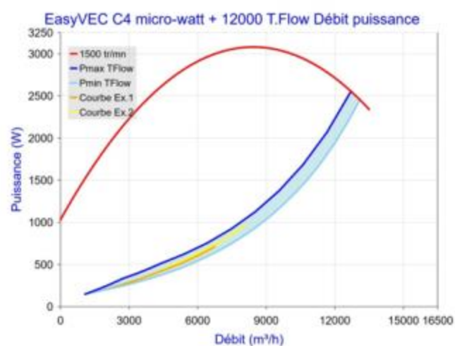
Figure 73 - EasyVEC C4 micro-watt + 12000 avec T.Flow Hygro+/ T.Flow Nano
