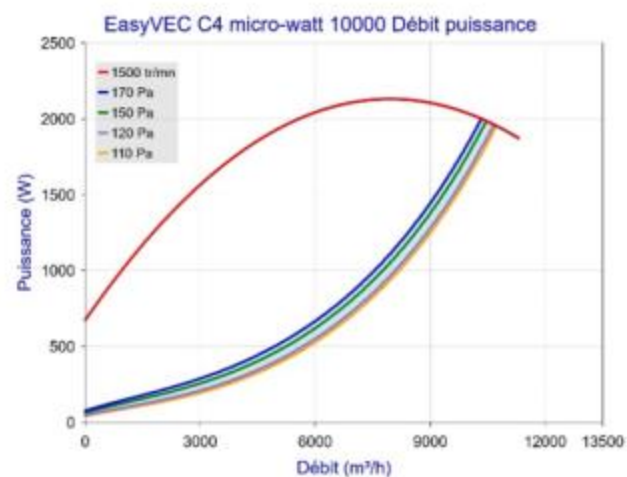
Figure 62 – EasyVEC C4 micro-watt 10000 (avec ou sans T.Flow Hygro+/T.Flow Nano)
