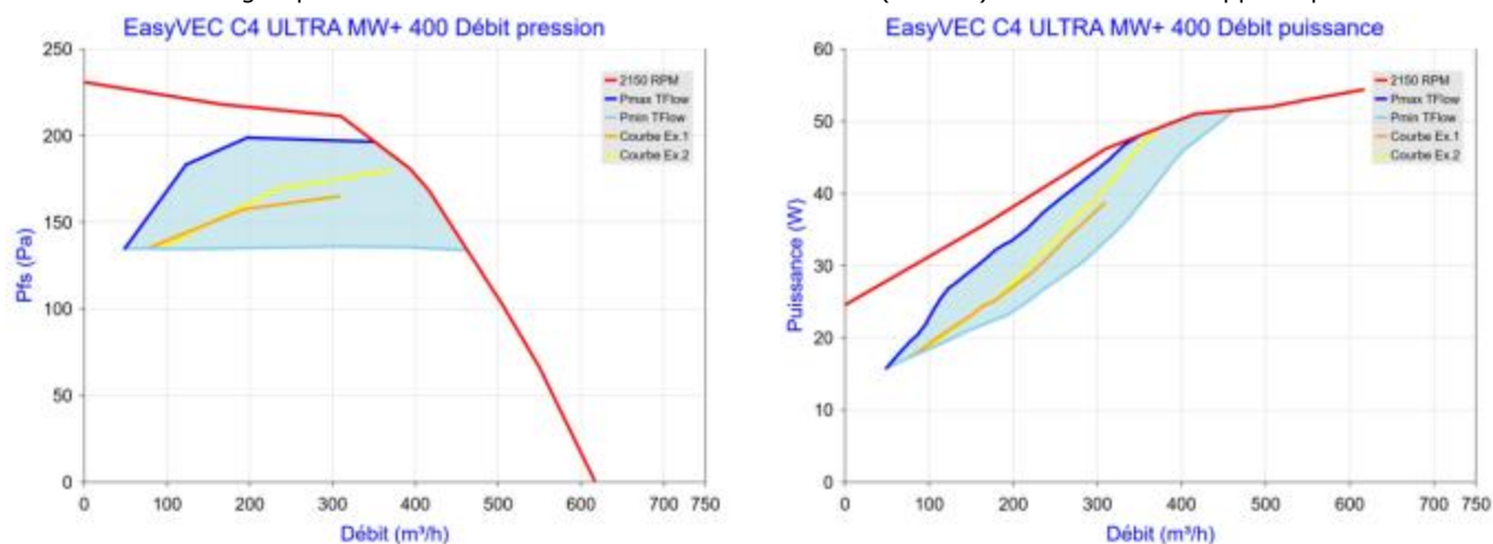
Figure 90 - EasyVEC C4 ULTRA MW+ 400 avec T.Flow Hygro+/ T.Flow Nano
