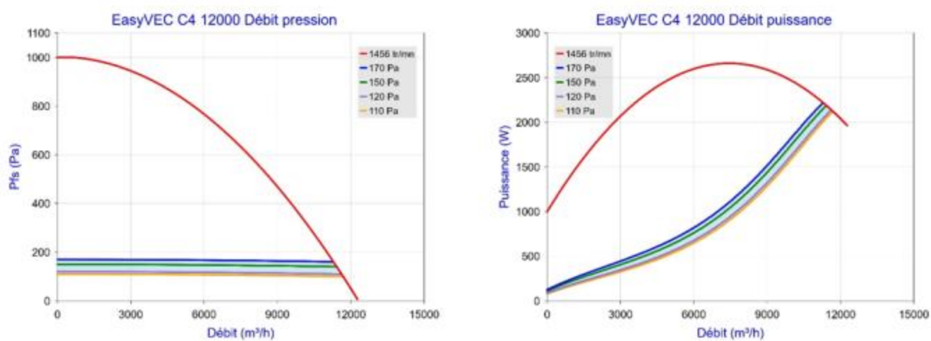
Figure 58 – EasyVEC C4 12 000 (avec ou sans T.Flow Hygro+/T.Flow Nano)
