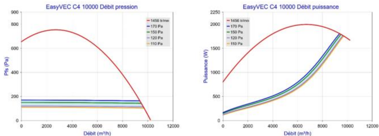
Figure 57 – EasyVEC C4 10000 (avec ou sans T.Flow Hygro+/T.Flow Nano)
