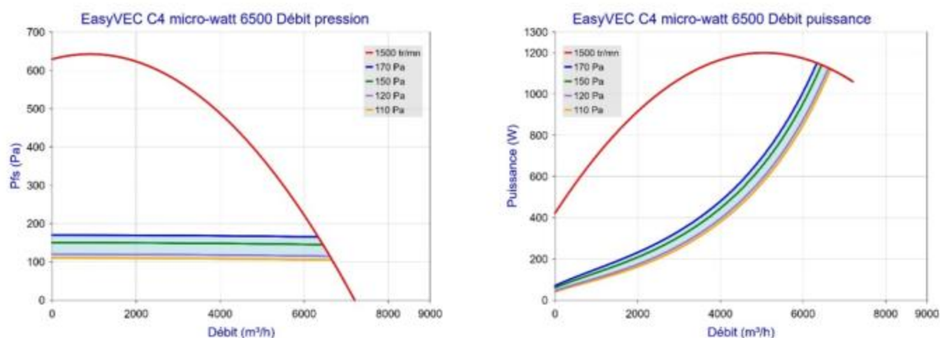
Figure 60 – EasyVEC C4 micro-watt 6500 (avec ou sans T.Flow Hygro+/T.Flow Nano)
