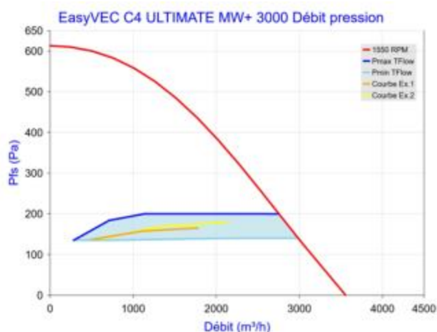
Figure 112 - EasyVEC C4 ULTIMATE MW+ 3000 avec T.Flow Hygro+/T.Flow Nano
