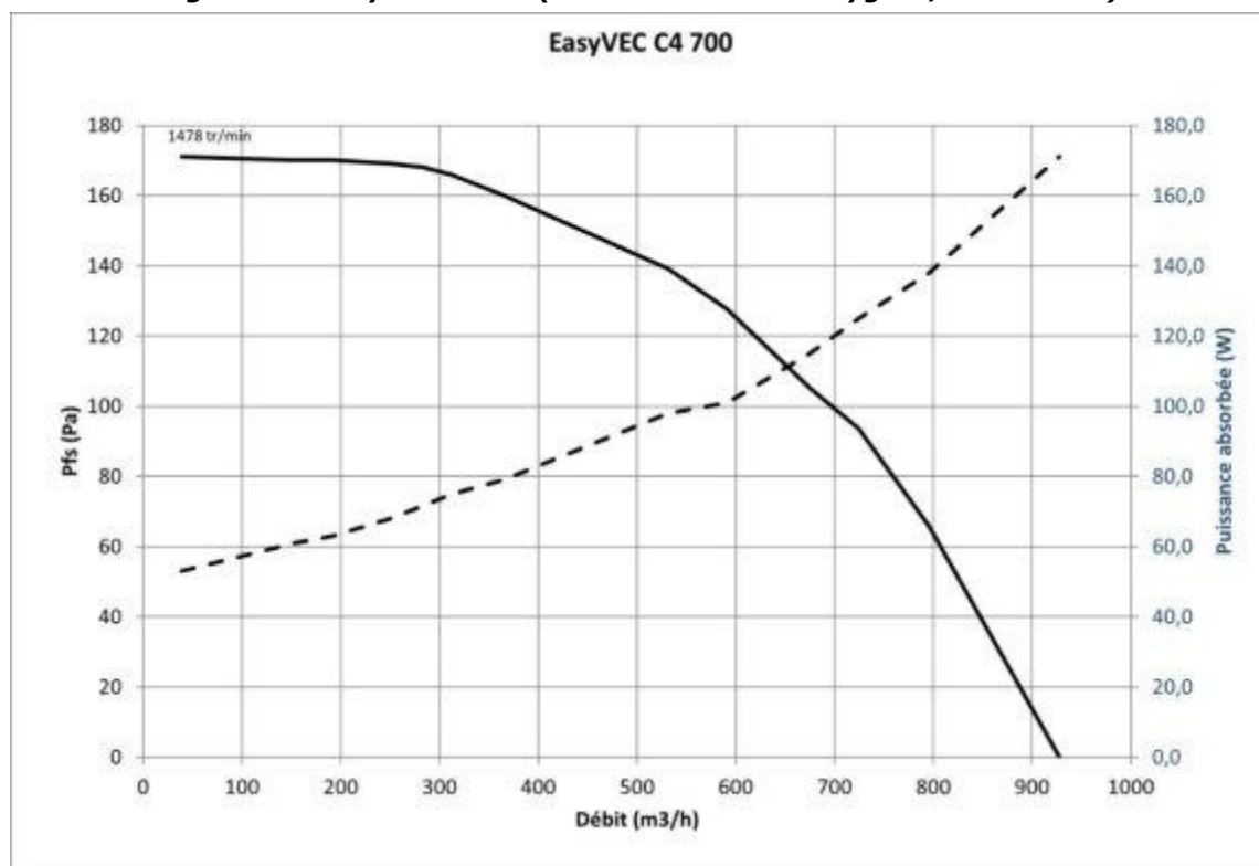
Figure 49 - EasyVEC C4 700 (avec ou sans T.Flow Hygro+/T.Flow Nano)
