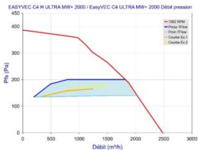
Figure 94 - EasyVEC C4 (H) ULTRA MW+ 2000 avec T.Flow Hygro+/ T.Flow Nano
