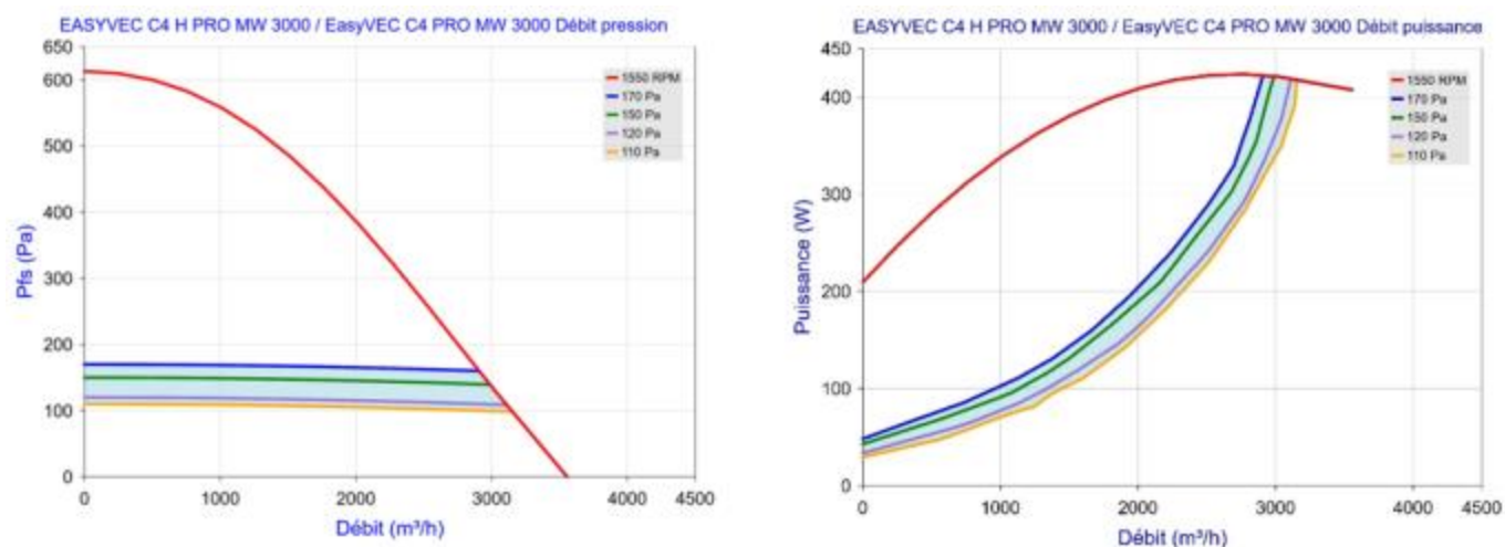
Figure 80 – EasyVEC C4 (H) PRO MW 3000 (avec ou sans T.Flow Hygro+/T.Flow Nano)
