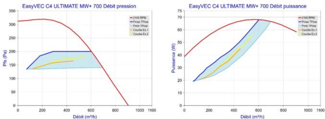
Figure 107 - EasyVEC C4 ULTIMATE MW+ 700 avec T.Flow Hygro+/T.Flow Nano
