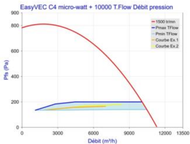
Figure 72 - EasyVEC C4 micro-watt + 10000 avec T.Flow Hygro+/ T.Flow Nano
