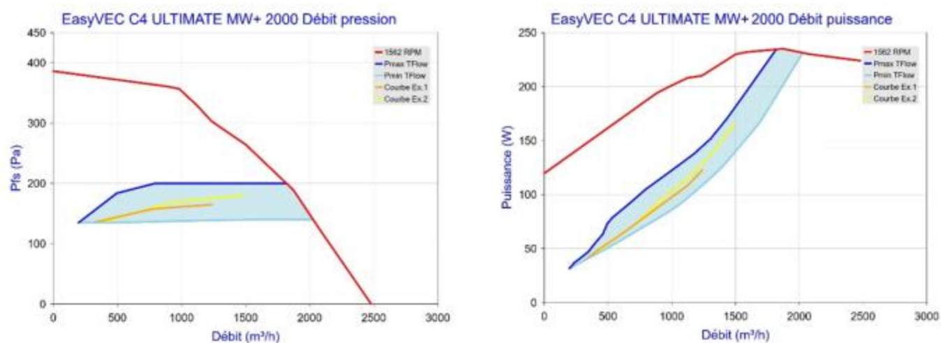
Figure 110 - EasyVEC C4 ULTIMATE MW+ 2000 avec T.Flow Hygro+/T.Flow Nano
