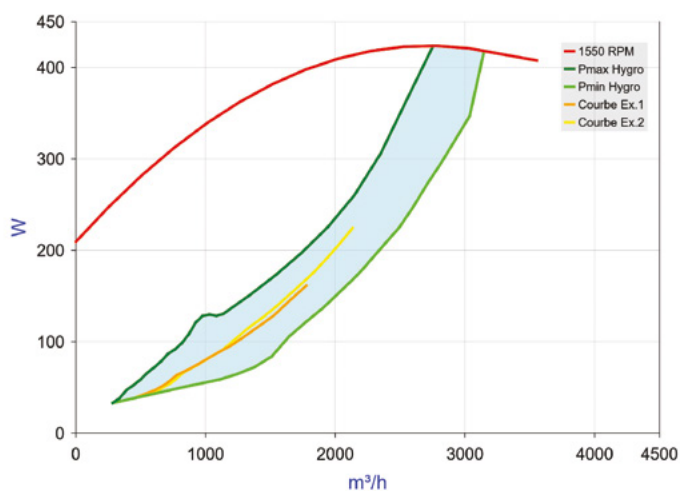
EasyVEC® C4 ULTRA-MW+ 3 000 - Débit puissance
