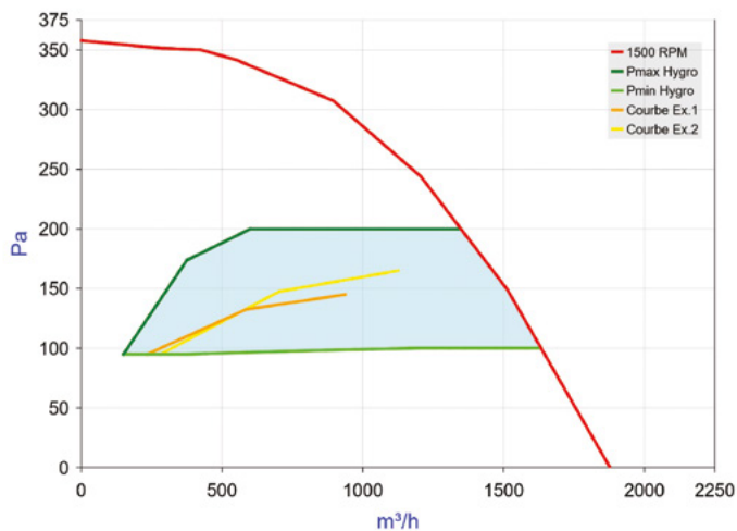
EasyVEC® C4 ULTIMATE-MW+ 2 000 - Débit pression
