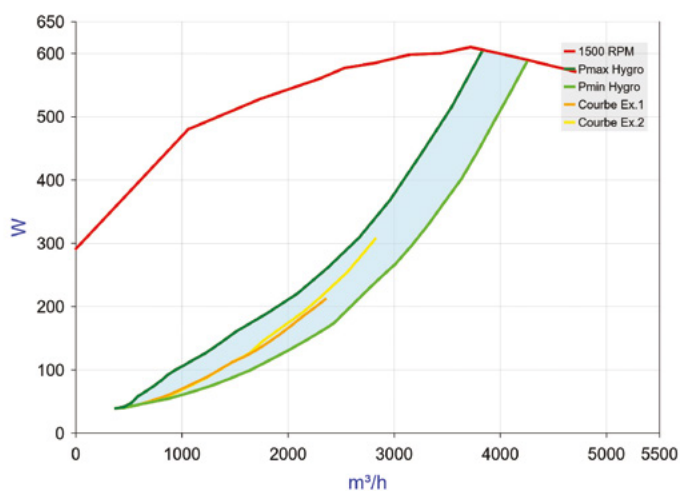
EasyVEC® C4 ULTRA-MW+ 4 000 - Débit puissance
