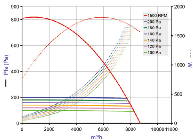
EasyVEC® C4 micro-watt 8 000 - Débit pression / puissance
