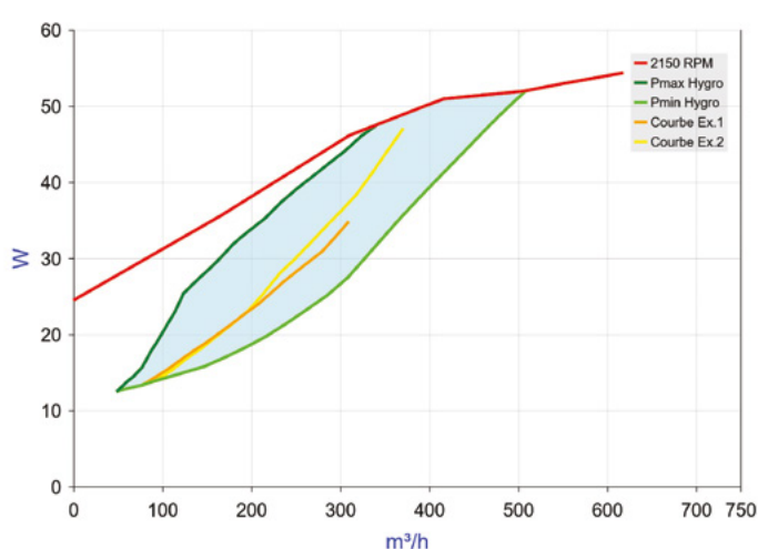
EasyVEC® C4 ULTRA-MW+ 700 - Débit puissance
