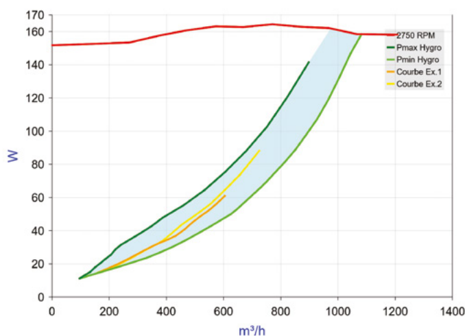
EasyVEC® C4 ULTRA-MW+ 1 000 - Débit puissance
