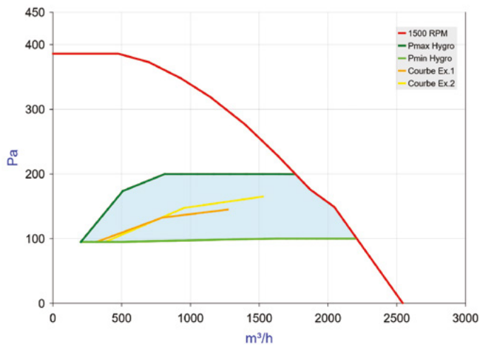
EasyVEC® C4 ULTIMATE-MW+ 2 500 - Débit pression
