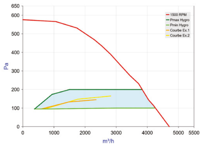
EasyVEC® C4 ULTRA-MW+ 4 000 - Débit pression
