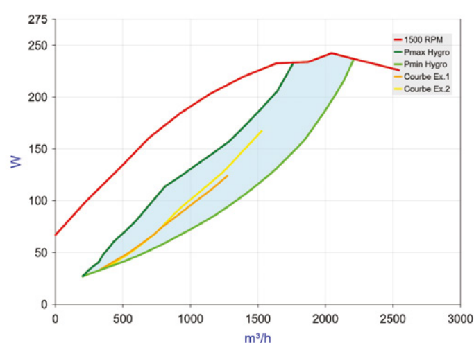
EasyVEC® C4 ULTRA-MW+ 2 000 - Débit puissance
