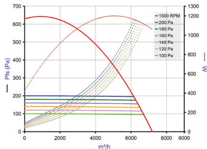
EasyVEC® C4 micro-watt 6 500 - Débit pression / puissance
