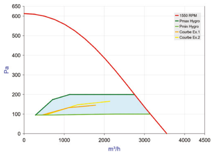
EasyVEC® C4 ULTRA-MW+ 3 000 - Débit pression
