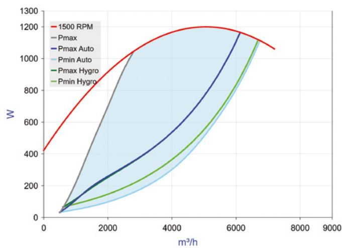
EasyVEC® C4 micro-watt+ 8 000 - Débit puissance
