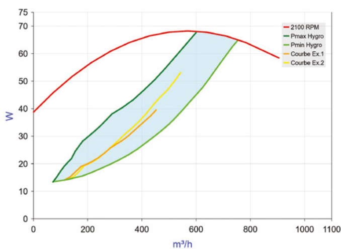
EasyVEC® C4 ULTRA-MW+ 700 - Débit puissance
