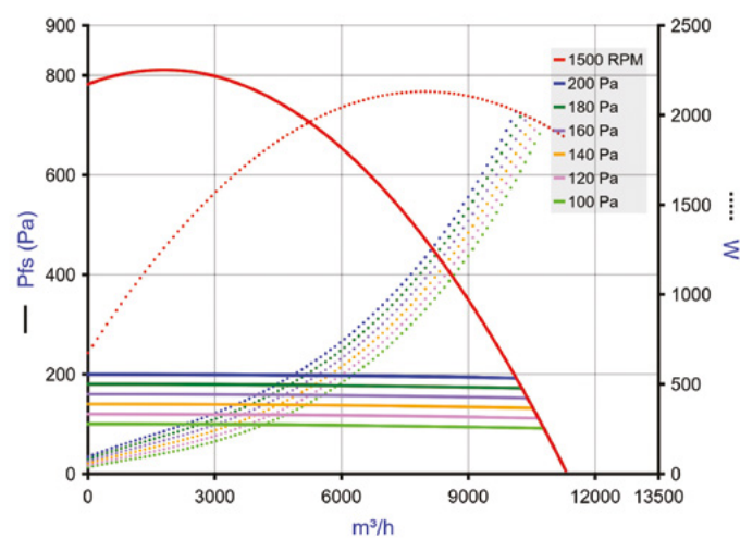
EasyVEC® C4 micro-watt 10 000 - Débit pression / puissance
