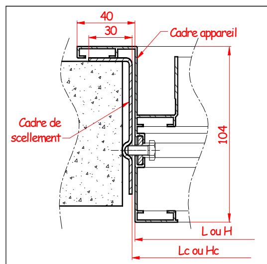
6 - Présenter l'OXYTONE LAMES dans le cadre de scellement, puis brider l'ensemble à l'aide des vis de blocage.
