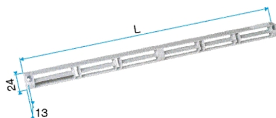
Figure 15 – Auvent standard pour mini EA 30 [2]
