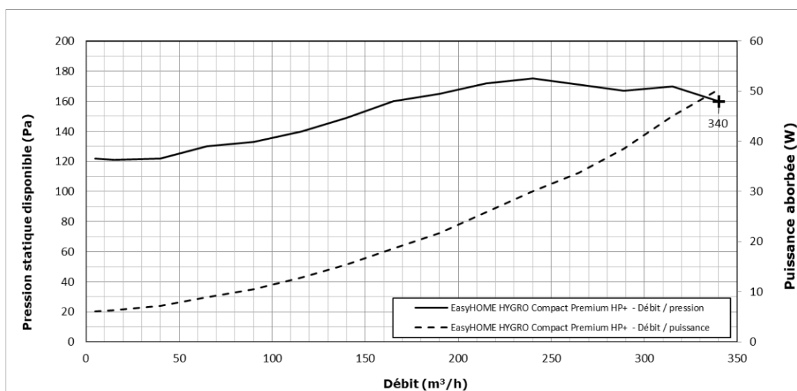
Figure 57 - Groupe d'extraction « EasyHOME HYGRO COMPACT Premium HP+ » - courbes caractéristiques
