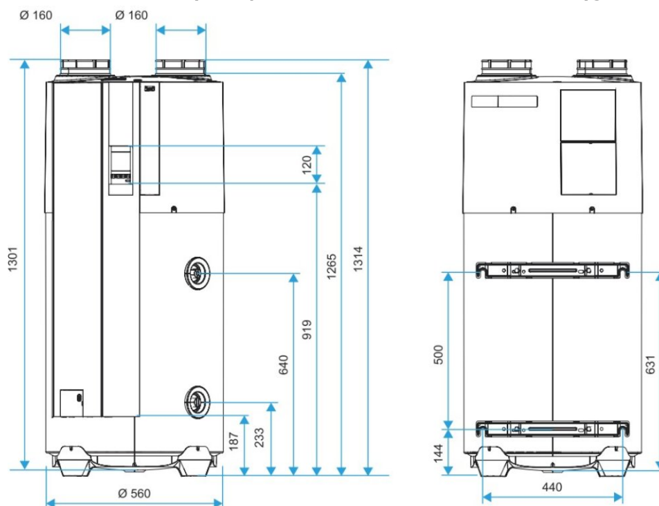
Figure 47 – Chauffe-eau thermodynamique sur air extrait « B100-FAN_T.Flow Nano MP » - visuels
