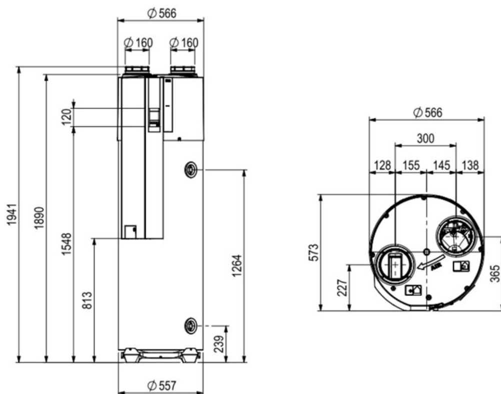
Figure 46 – Chauffe-eau thermodynamique sur air extrait « B200-FAN_T.Flow Hygro+ MP » - visuels
