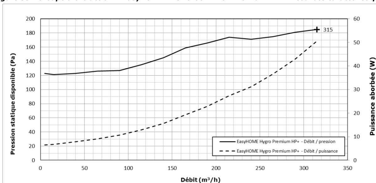
Figure 56 - Groupe d'extraction « EasyHOME HYGRO Premium HP+ » - courbes caractéristiques
