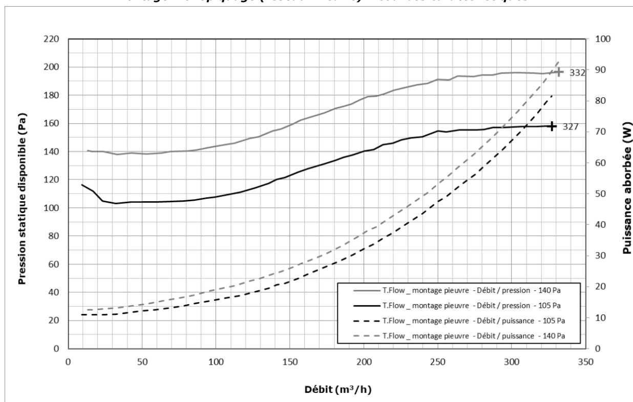
Figure 59 – Chauffe-eau thermodynamiques sur air extrait « B200-FAN_T.Flow Hygro+ MP » et « B100-FAN_T.Flow Nano MP » Montage multipiquage (réseau en pieuvre) – courbes caractéristiques
