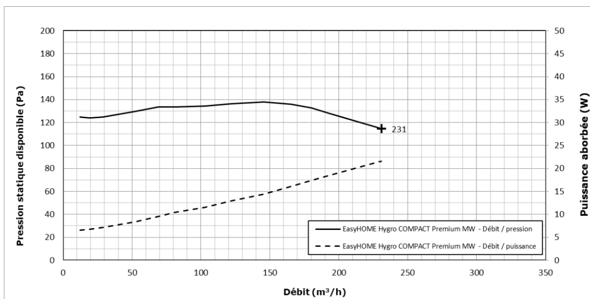
Figure 54 - Groupe d'extraction « EasyHOME HYGRO COMPACT Premium MW » - courbes caractéristiques
