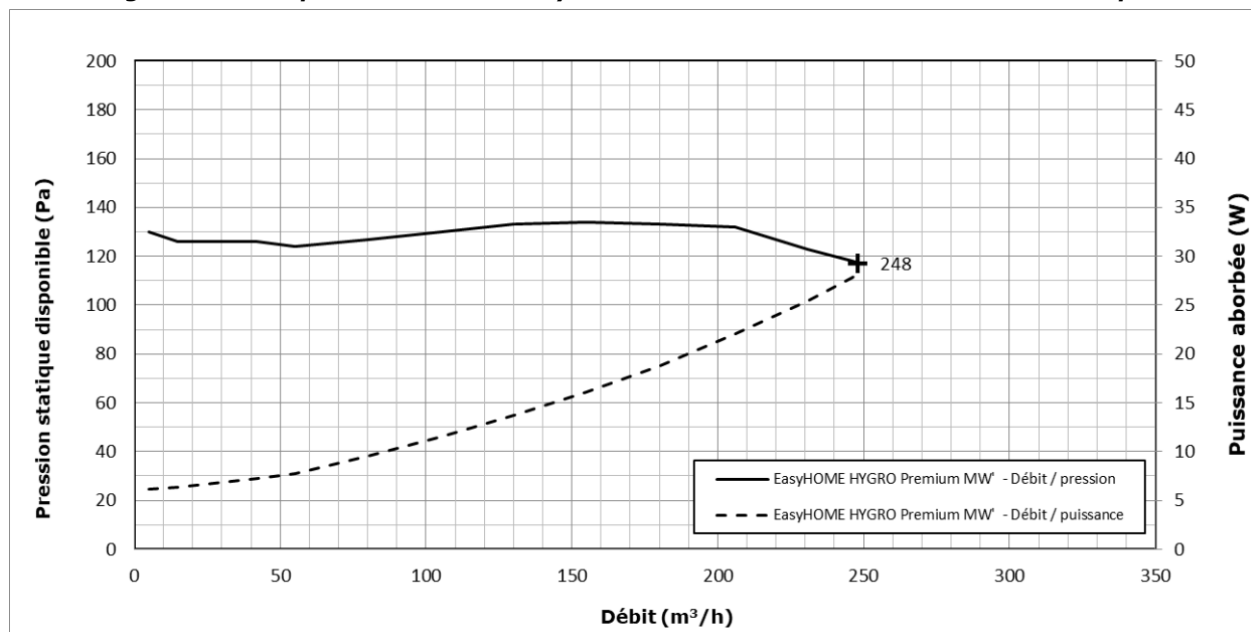
Figure 50 - Groupe d'extraction « EasyHOME HYGRO Premium MW' » - courbes caractéristiques
