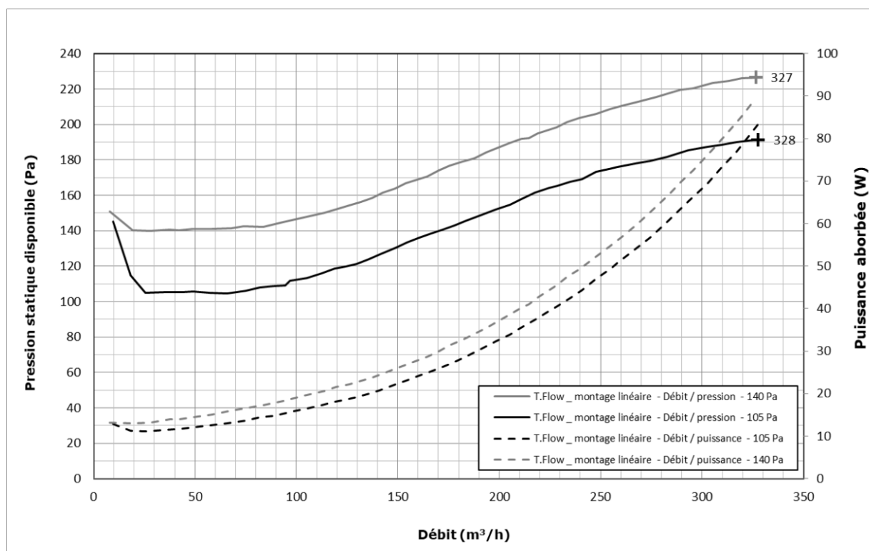
Figure 58 – Chauffe-eau thermodynamiques sur air extrait « B200-FAN_T.Flow Hygro+ MP » et « B100-FAN_T.Flow Nano MP » Montage monopiquage (réseau linéaire) – courbes caractéristiques
