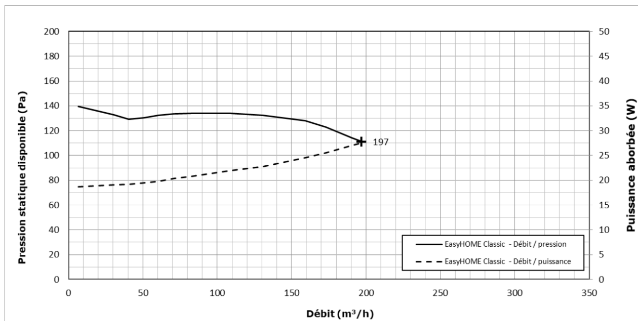
Figure 49 - Groupe d'extraction « EasyHOME HYGRO Classic » - courbes caractéristiques
