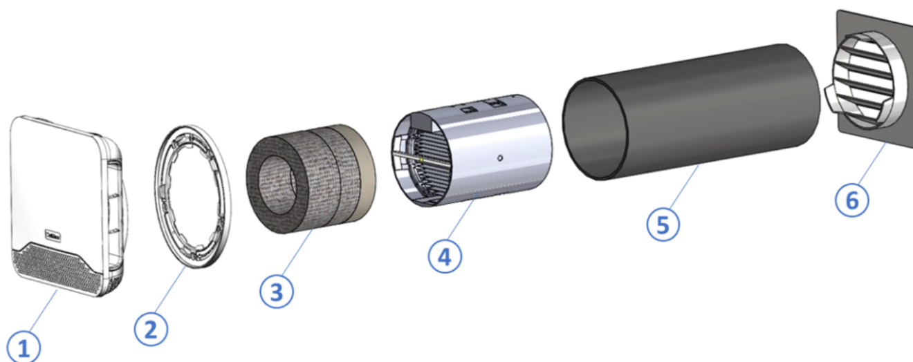
Figure 27 – Mise en œuvre entrée d'air EHT² ou EFT² avec électrofiltre EHT²/EFT² sans mousse Ø 125 mm L 300 mm
