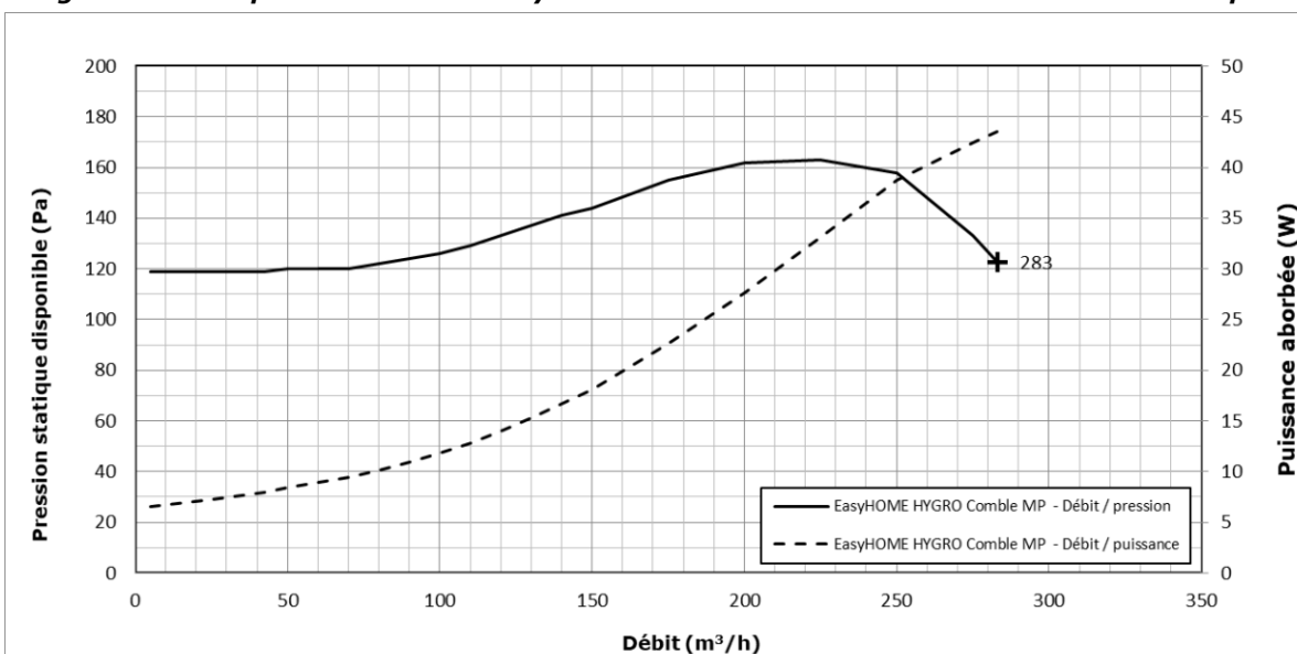
Figure 52 - Groupe d'extraction « EasyHOME HYGRO Comble MP » - courbes caractéristiques
