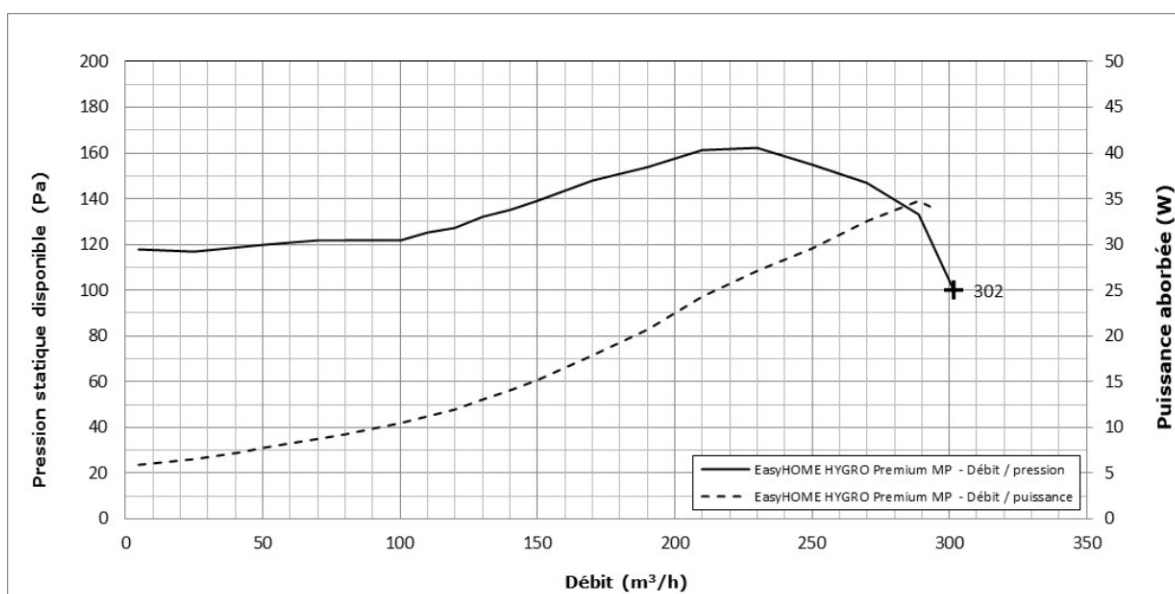
Figure 51 - Groupe d'extraction « EasyHOME HYGRO Premium MP » - courbes caractéristiques
