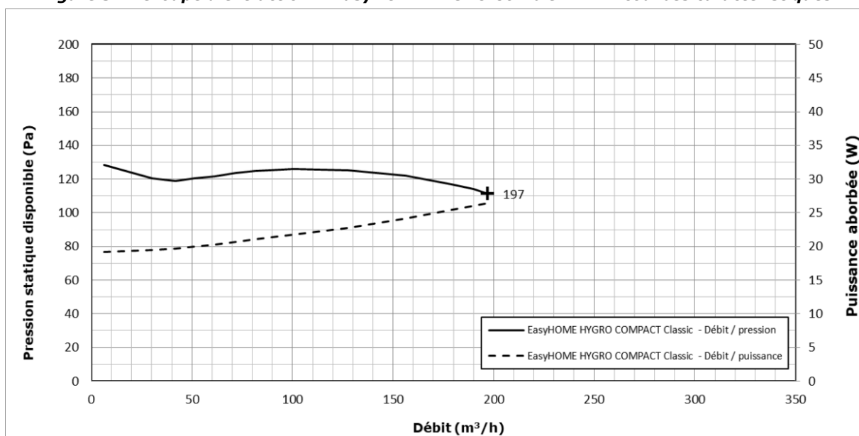
Figure 53 - Groupe d'extraction « EasyHOME HYGRO COMPACT Classic » - courbes caractéristiques
