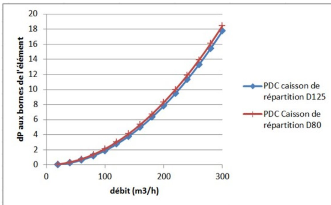
Figure 60 – Caissons de répartition pour chauffe-eau thermodynamique sur air extrait « B200-FAN_T.Flow Hygro+ » et « B100-FAN_T.Flow Nano MP » - courbes caractéristiques
