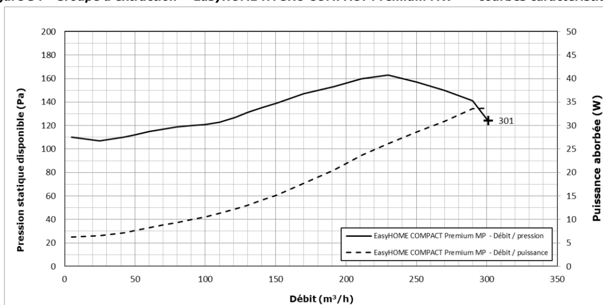
Figure 55 - Groupe d'extraction « EasyHOME HYGRO COMPACT Premium MP » - courbes caractéristiques
