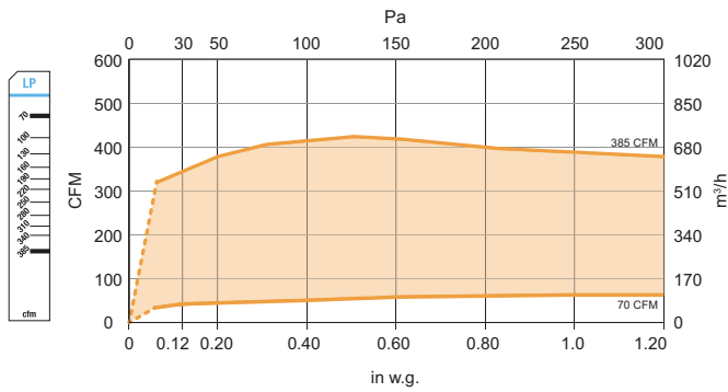
Basse pression
