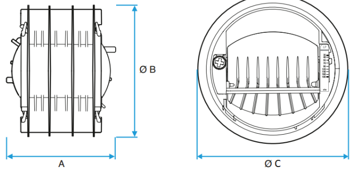
VUE LATÉRALE
