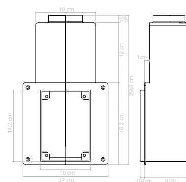
Encombrement contre-prise mur brique pour flexible rétractable
