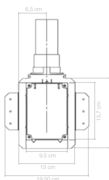
Encombrement contre-prise cloison sèche pour flexible rétractable
