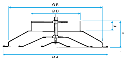
Diffuseur A 842
