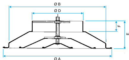
Diffuseur A 842
