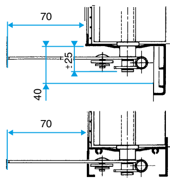
Poignée de commande manuelle AG 645
