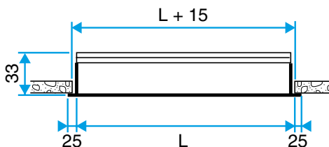
Diffuseur ALD 610 - 620
