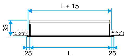
Diffuseur ALD 610 - 620
