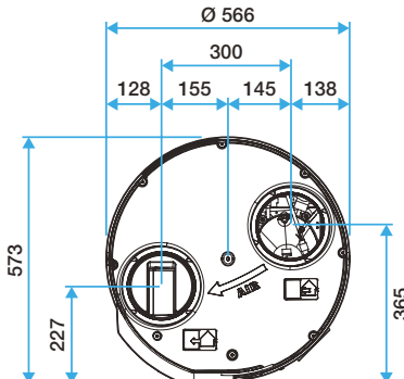
Encadrement T.Flow® Hygro+ - Raccordement aéraulique
