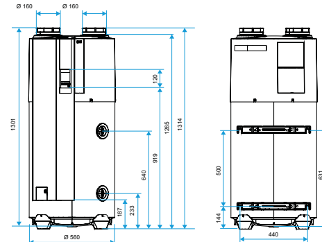
Encadrement T.Flow® Nano
