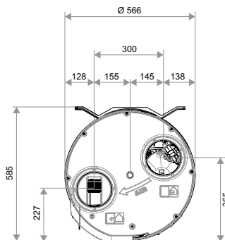
Encadrement T.Flow® Hygro+ - Raccordement aéraulique
