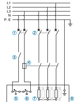
Raccordement pour BCA triphasée
