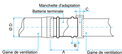
Installation en gaine
