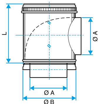
Schéma d'encombrement Caisson Piquage Acoustique et Aéraulique en aluminium
