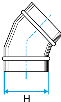
Schéma d'encombrement Coude Vertical Oblong 45°
