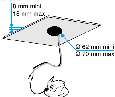
Installation électrique Optic Mod
