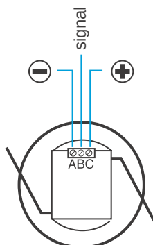
Installation électrique Optic Mod 2
