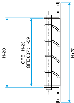
Encombrement vue de profil (mm)
