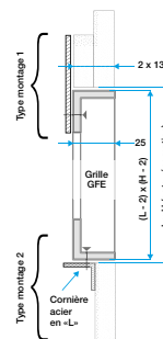
Exemple de mise en oeuvre GFE 007 - Cadre apparent
