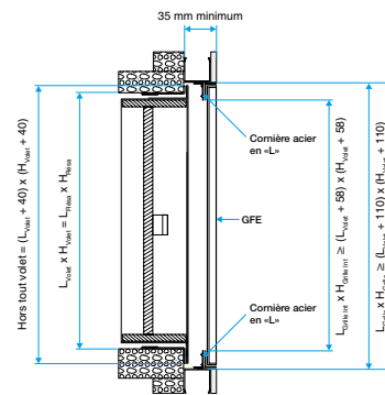
Cotes nominales pour installation devant un volet OPTONE
