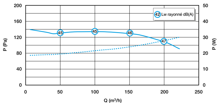
Courbe aéraulique et acoustique EasyHOME Hygro Classic
