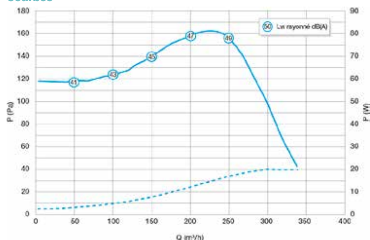
Courbes aéraulique, de consommation et valeurs acoustiques EasyHOME HYGRO MP
