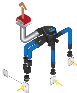
Installation avec conduits semi-rigides OPTIFLEX® isolés
