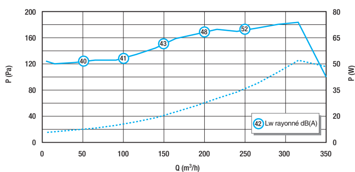
Courbe aérodynamique et acoustique EasyHOME Hygro Premium HP+
