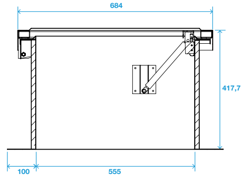
Encombremment SOS VELONE - Kit Souche Terrasse
