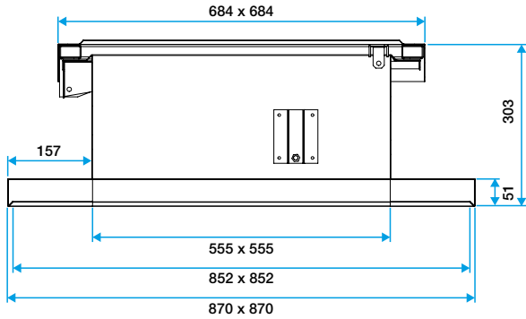
Encombremment SOS VELONE - Kit Rehausse
