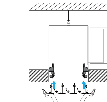
Diffuseur de soufflage avec fixation S3
