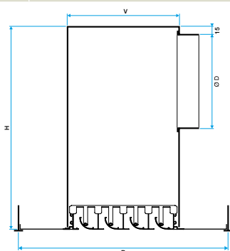
Avec montage sur plafond avec profil T (modèle soufflage)
