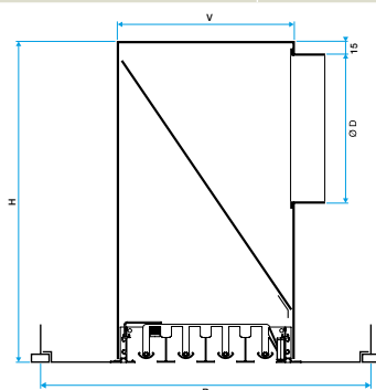
Avec montage sur plafond avec profil Fine-Line (modèle reprise avec filtre)
