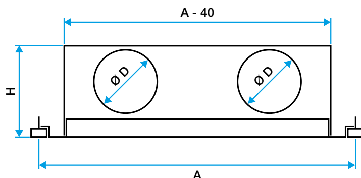
Avec montage sur plafond avec profil Fine-Line (modèle reprise avec filtre)
