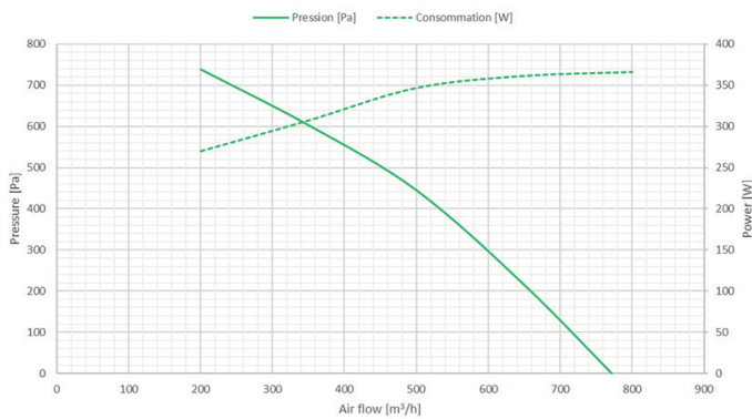
Courbe aéraulique DFE R TOP 700
