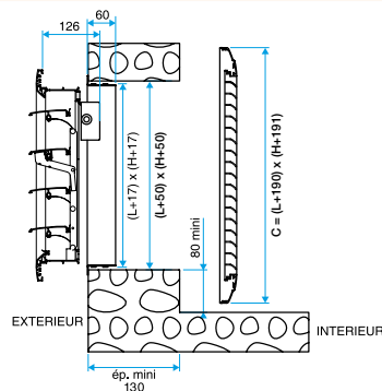
Encombrement avec GFAP 007 (mm)
