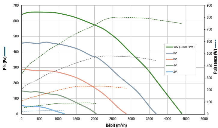
Courbes aérauliques et consommations électriques
