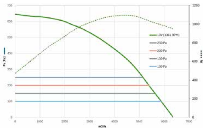
Courbes aérauliques et consommations électriques
