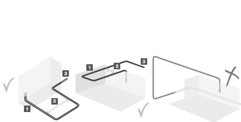
Encombrement coude allongé 90°
