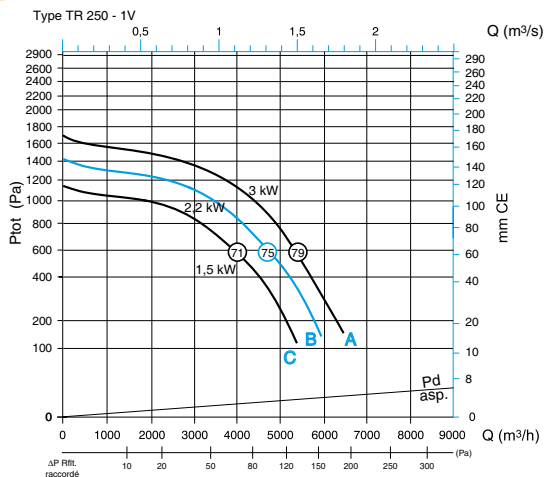
Caractéristiques aérauliques ProtectONE® TR 250 - 1V
