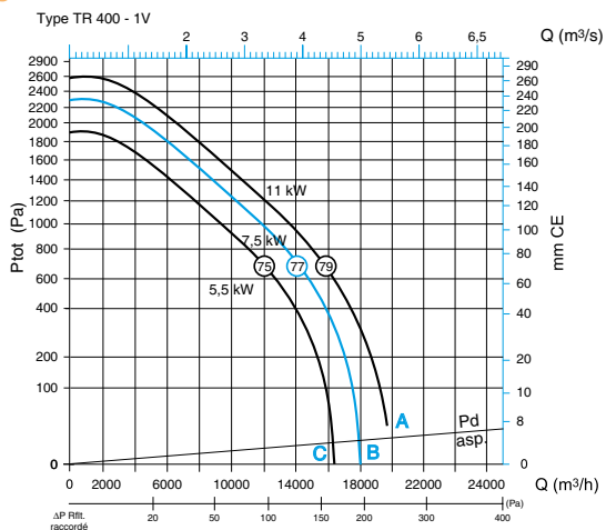
Caractéristiques aéroulliques ProtectONE® TR 400 - 1V
