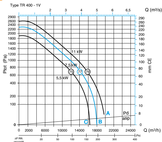
Caractéristiques aérauliques ProtectONE® TR 400 - 1V
