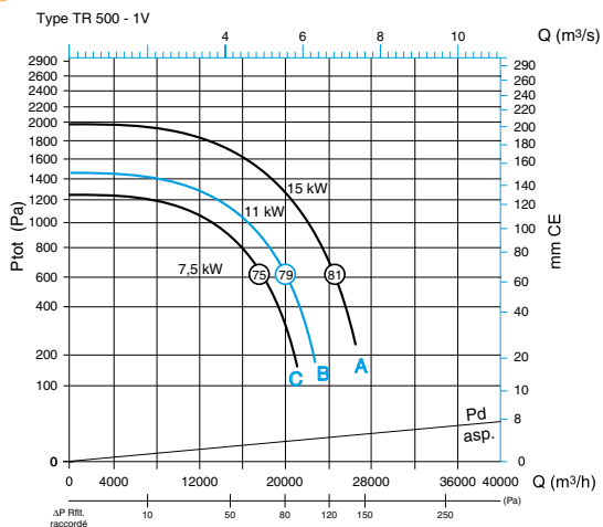
Caractéristiques aéroulliques ProtectONE® TR 500 - 1V
