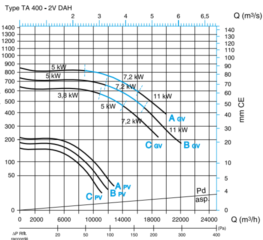
Caractéristiques aérauliques ProtectONE® TA 400 - 2V - DAH
