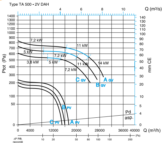
Caractéristiques aérouliques ProtectONE® TA 500 - 2V - DAH
