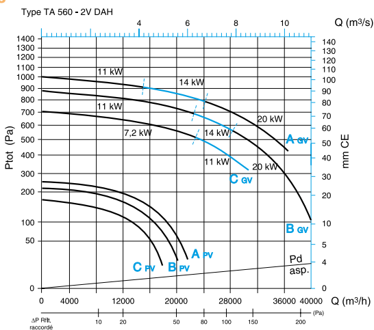
Caractéristiques aérouliques ProtectONE® TA 560 - 2V - DAH
