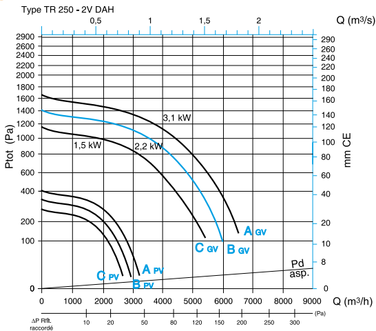
Caractéristiques aérauliques ProtectONE® TR 250 - 2V - DAH
