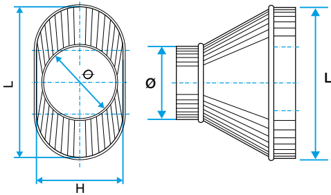
Schéma d'encombrement Réduction Concentrique Oblongue Cylindrique
