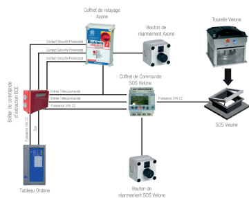
Principe d'installation et câblage du SOS VELONE
