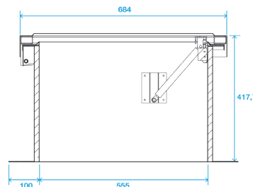
Encombrement SOS VELONE - Kit Souche Terrasse
