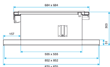
Encombrement SOS VELONE - Kit Rehausse
