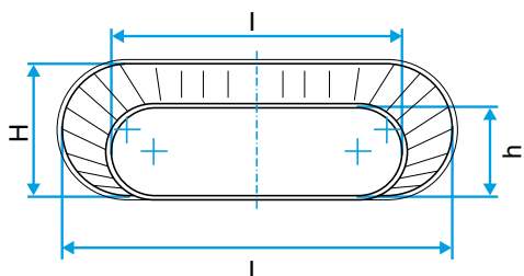
Schéma d'encombrement Réduction Oblongue Tangentielle sur Plat
