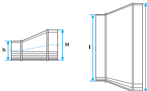
Schéma d'encombrement Réduction Oblongue Tangentielle sur Plat
