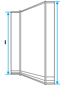
Schéma d'encombrement Réduction Oblongue Tangentielle sur Plat
